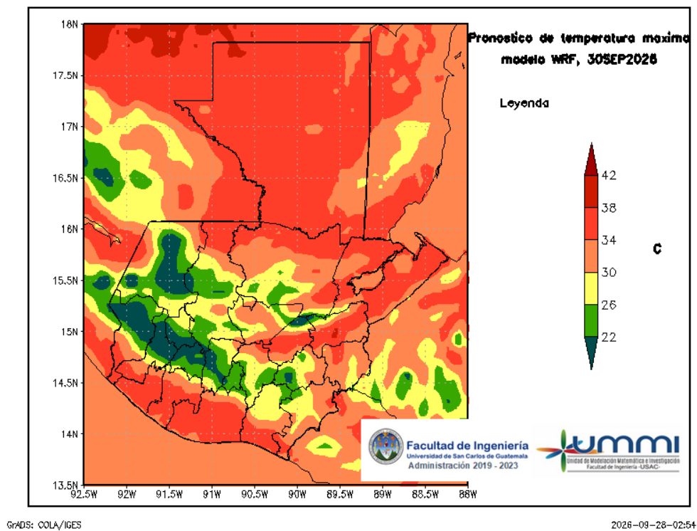
Figura 6: Pronóstico de temperatura máxima diaria del 30 de September
