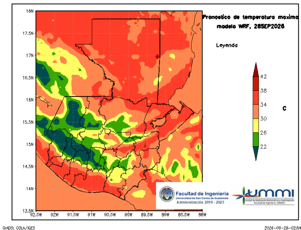
Figura 4: Pronóstico de temperatura máxima diaria del 28 de September
