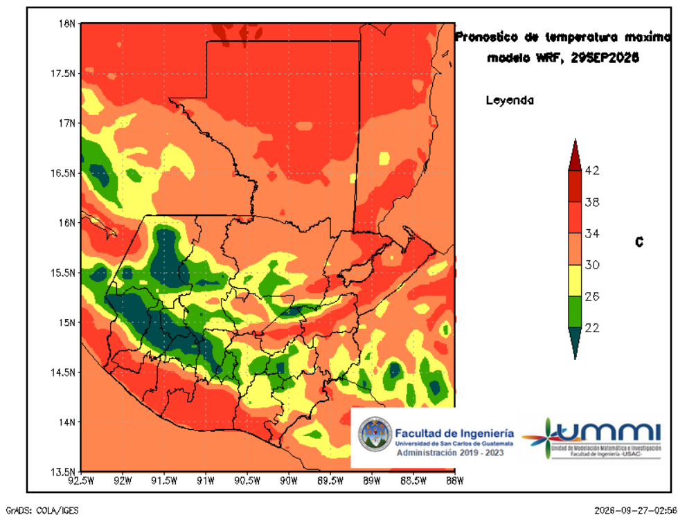
Figura 6: Pronóstico de temperatura máxima diaria del 29 de September
