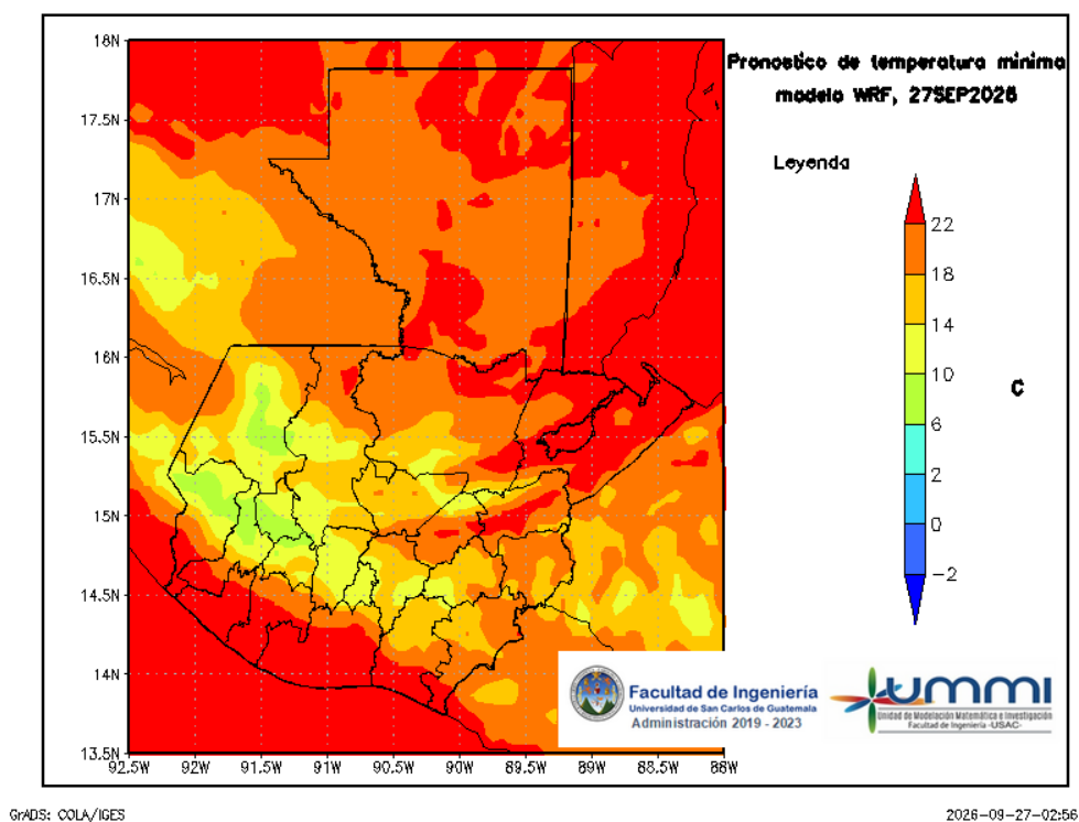
Figura 7: Pronóstico de temperatura mínima diaria del 28 de September
