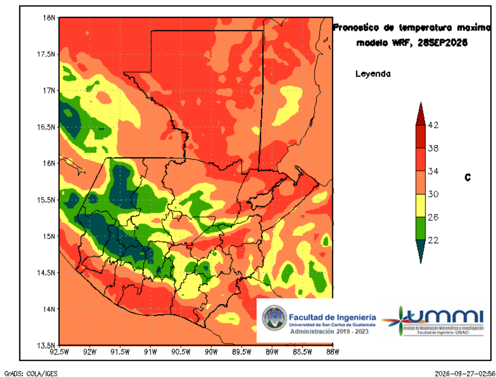
Figura 5: Pronóstico de temperatura máxima diaria del 28 de September
