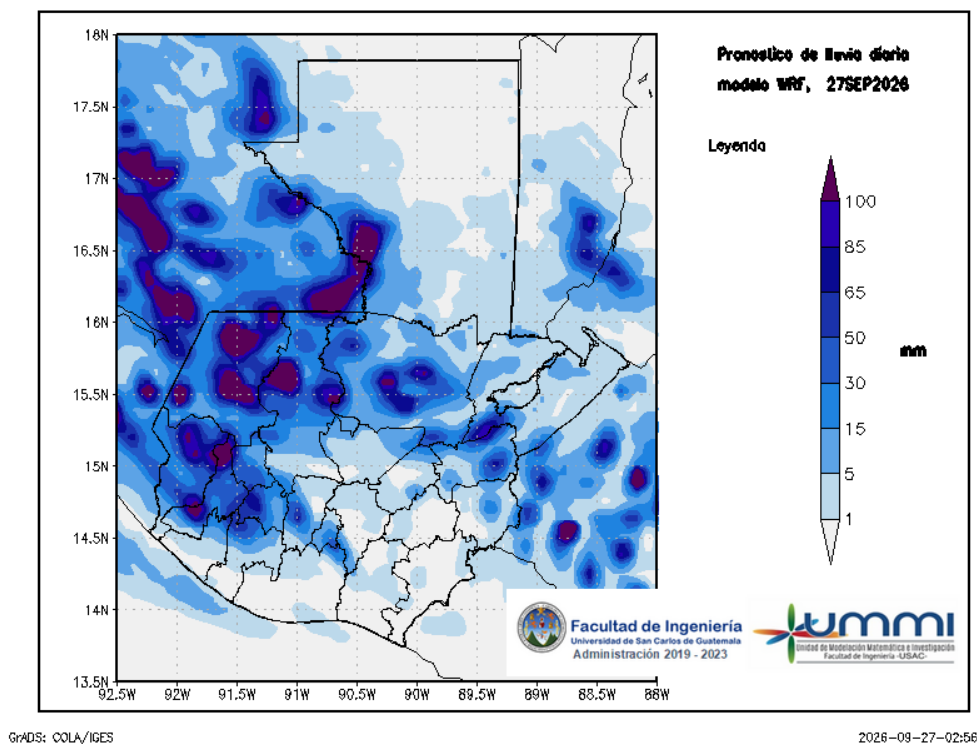
Figura 1: Pronóstico de lluvia diaria del 27 de September
