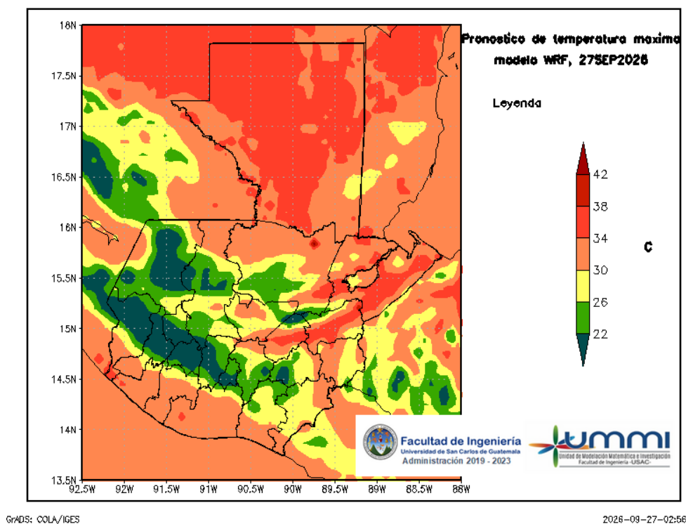
Figura 4: Pronóstico de temperatura máxima diaria del 27 de September
