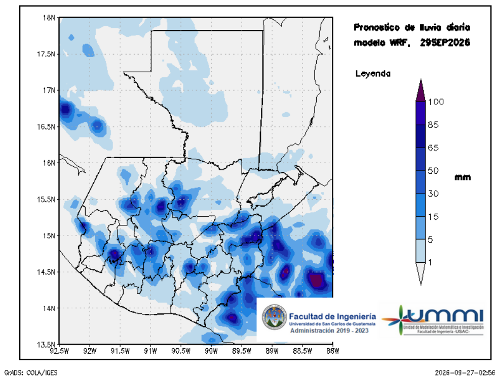
Figura 3: Pronóstico de lluvia diaria del 29 de September
