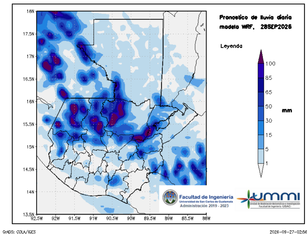
Figura 2: Pronóstico de lluvia diaria del 28 de September
