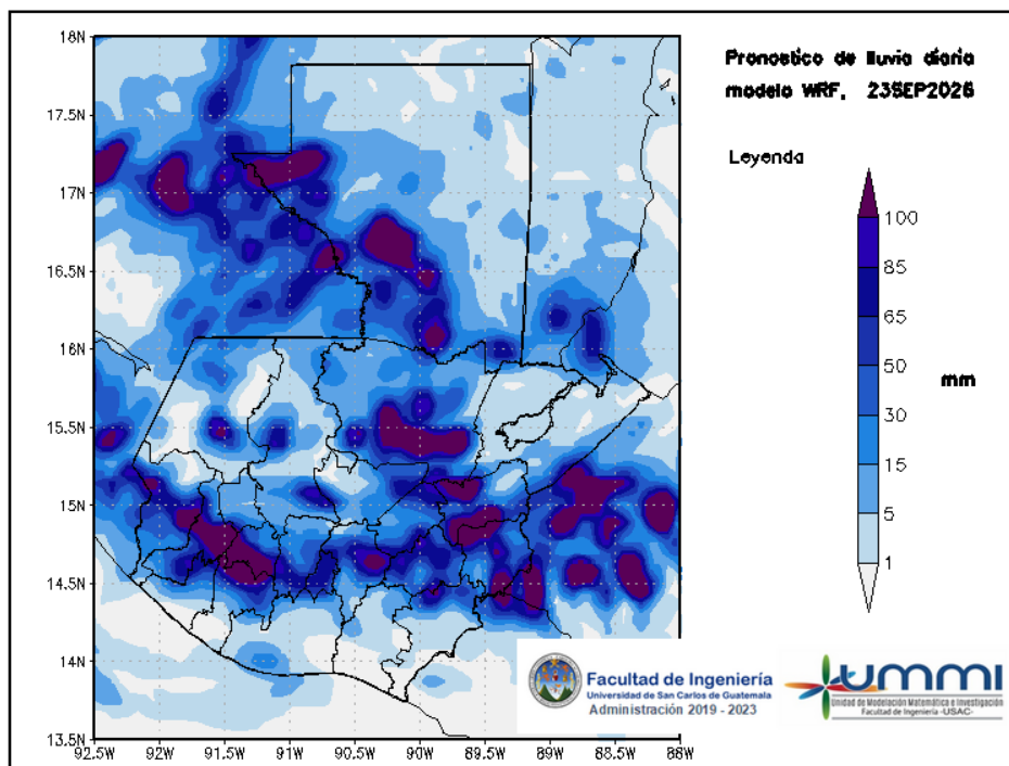
Figura 2: Pronóstico de lluvia diaria del 23 de September
