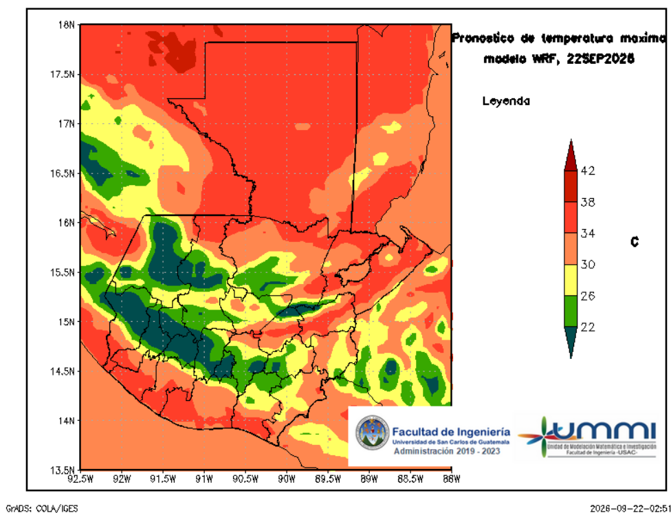
Figura 4: Pronóstico de temperatura máxima diaria del 22 de September
