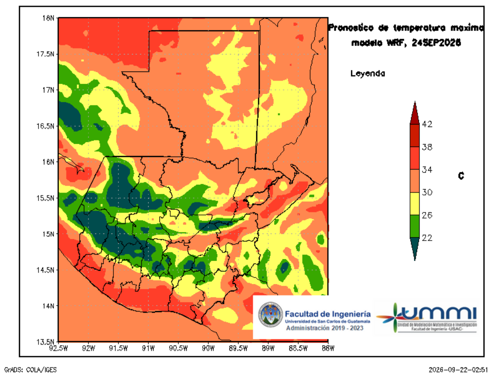
Figura 6: Pronóstico de temperatura máxima diaria del 24 de September
