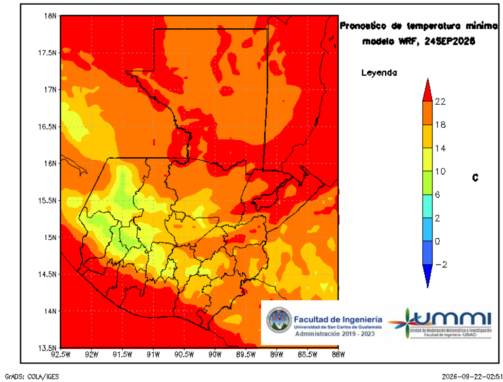
Figura 9: Pronóstico de temperatura mínima diaria del 25 de September
