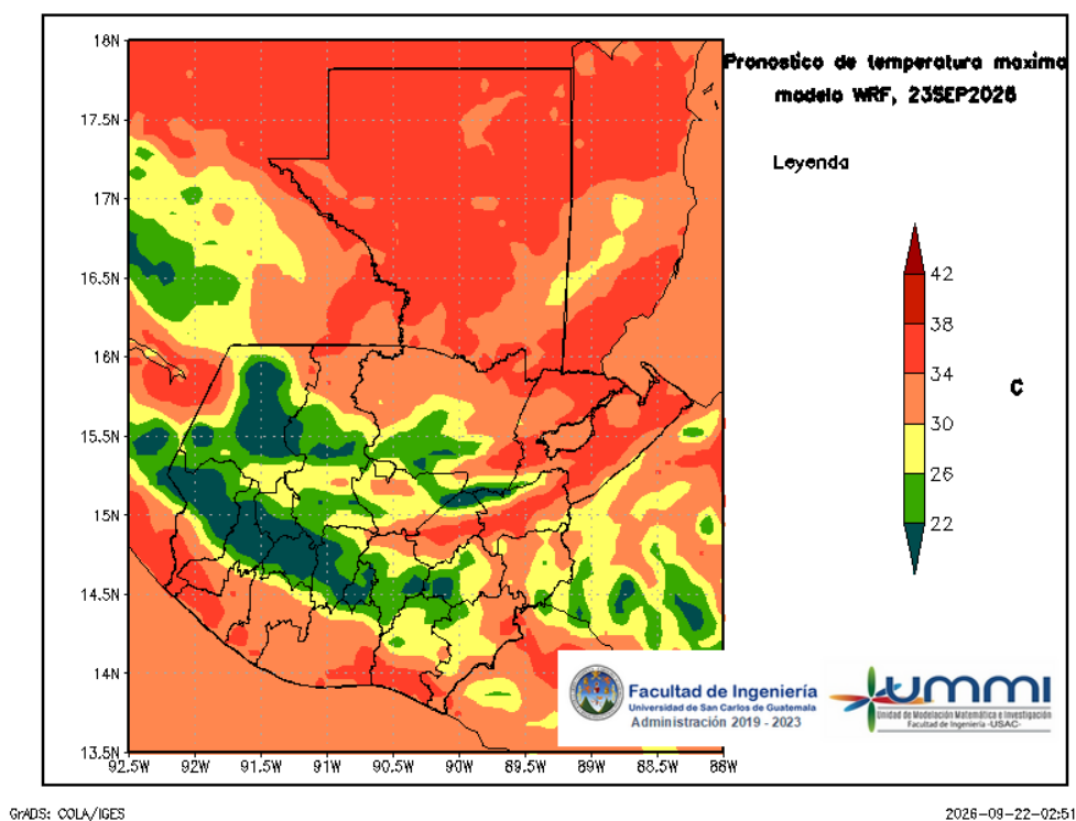
Figura 5: Pronóstico de temperatura máxima diaria del 23 de September
