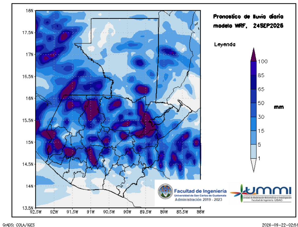
Figura 3: Pronóstico de lluvia diaria del 24 de September
