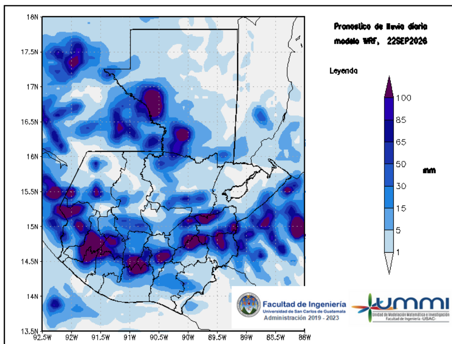
Figura 1: Pronóstico de lluvia diaria del 22 de September
