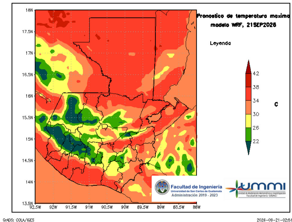
Figura 4: Pronóstico de temperatura máxima diaria del 21 de September
