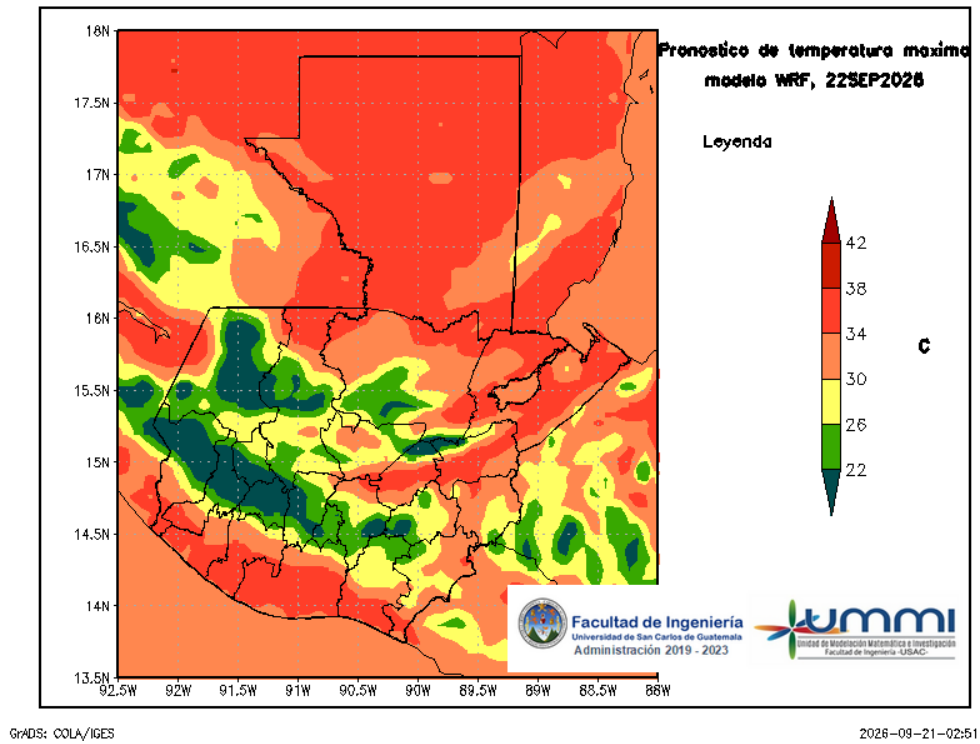
Figura 5: Pronóstico de temperatura máxima diaria del 22 de September
