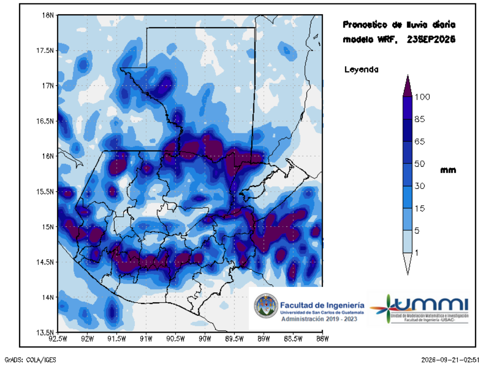
Figura 3: Pronóstico de lluvia diaria del 23 de September
