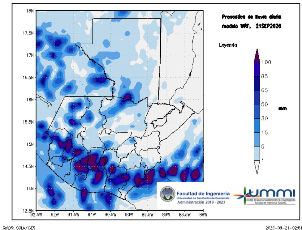
Figura 1: Pronóstico de lluvia diaria del 21 de September
