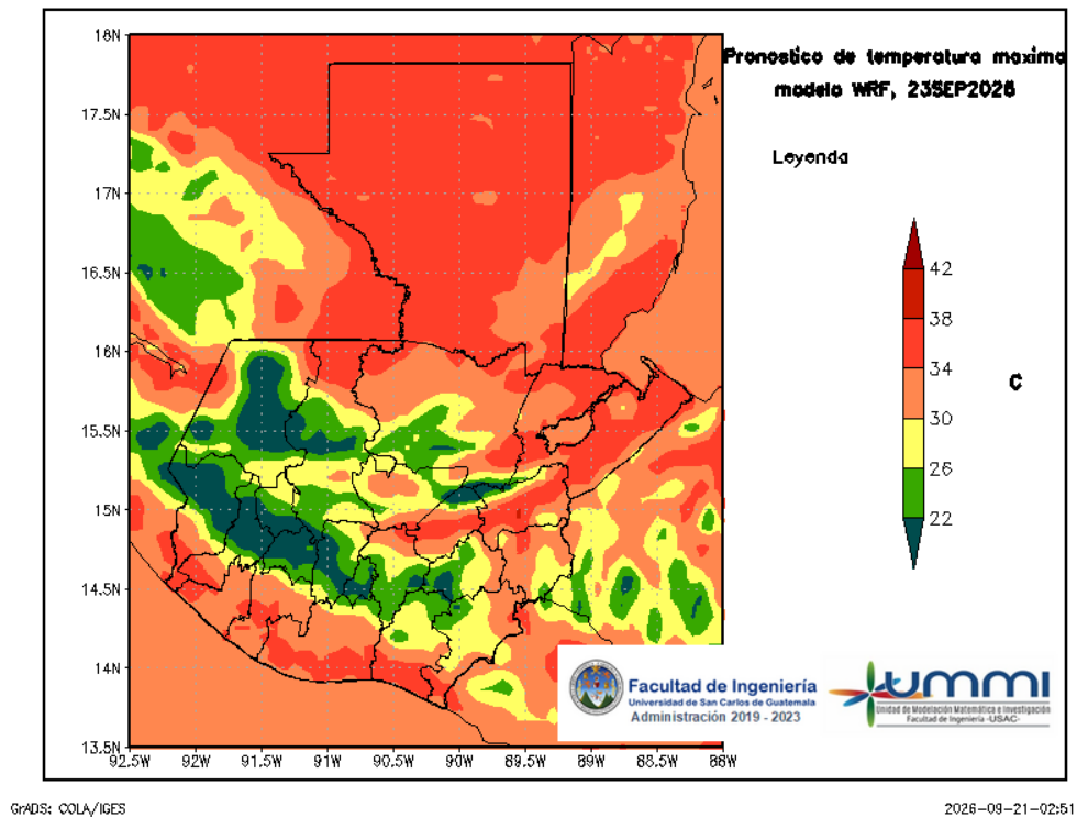
Figura 6: Pronóstico de temperatura máxima diaria del 23 de September
