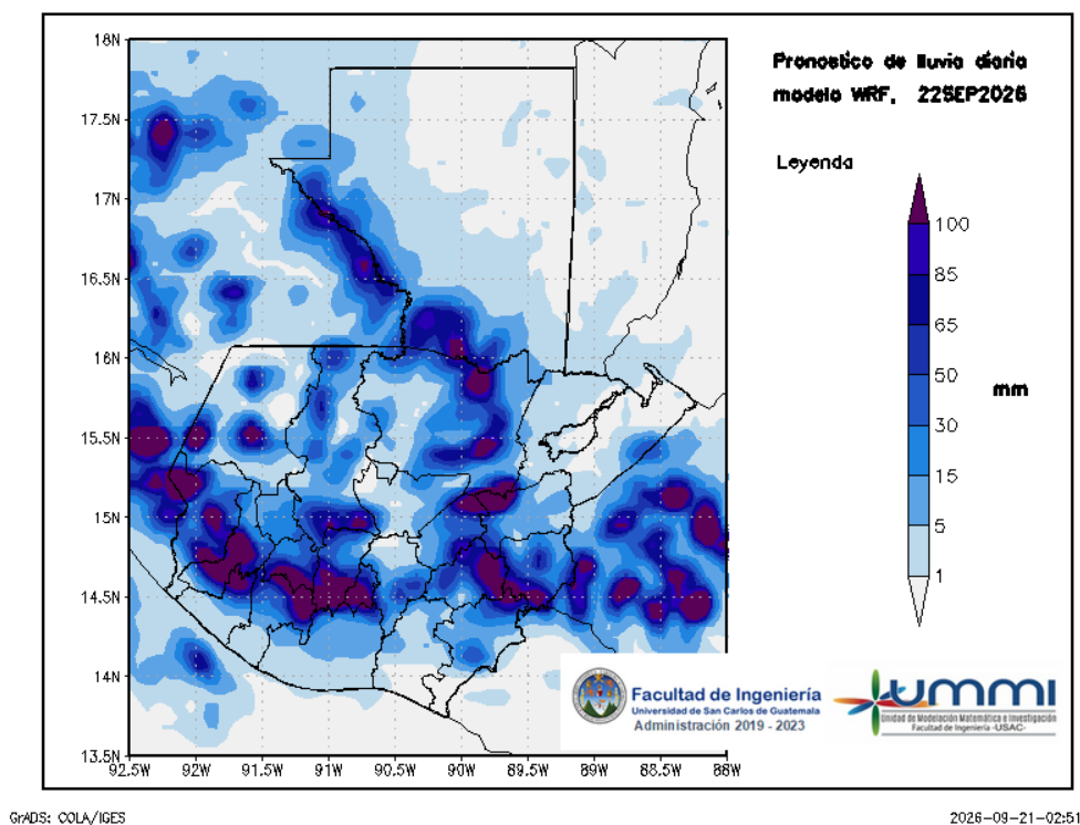
Figura 2: Pronóstico de lluvia diaria del 22 de September
