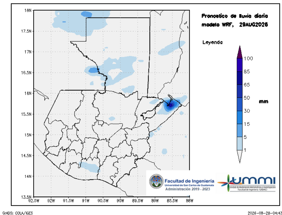
Figura 2: Pronóstico de lluvia diaria del 29 de August
