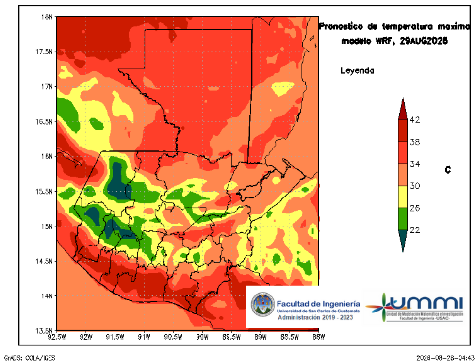
Figura 5: Pronóstico de temperatura máxima diaria del 29 de August
