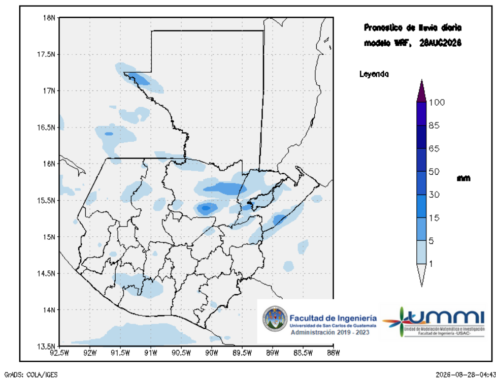
Figura 1: Pronóstico de lluvia diaria del 28 de August
