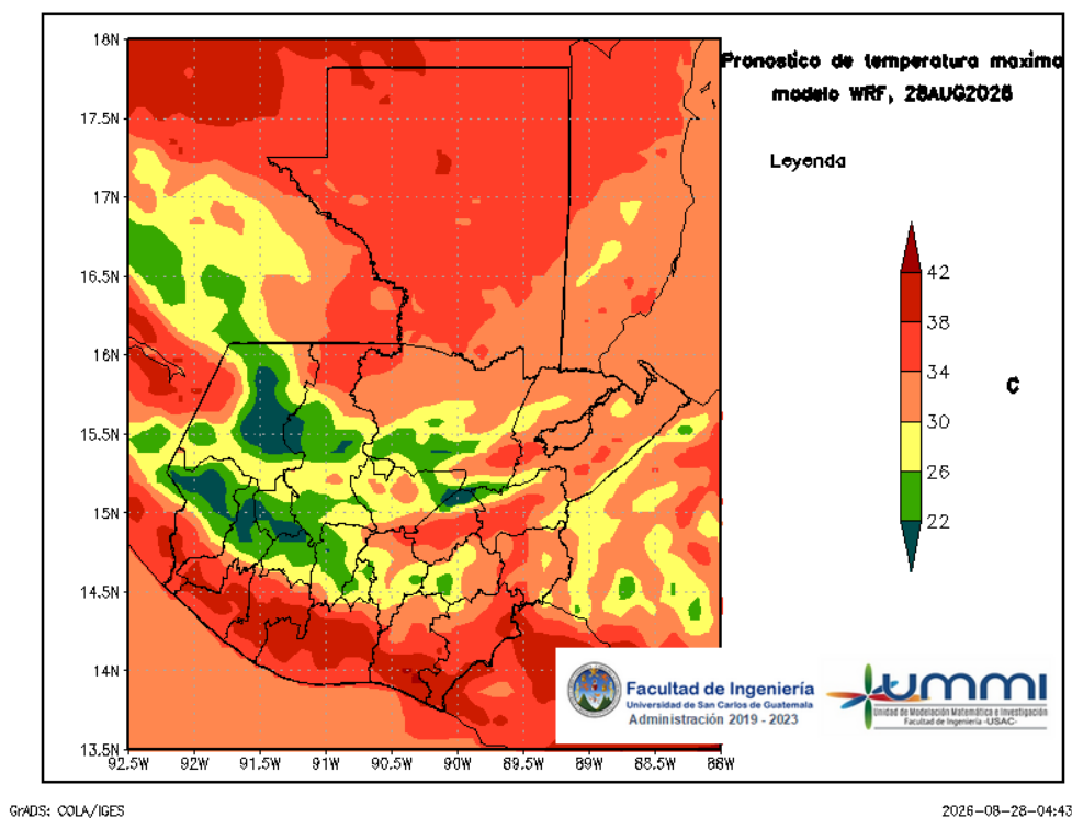
Figura 4: Pronóstico de temperatura máxima diaria del 28 de August
