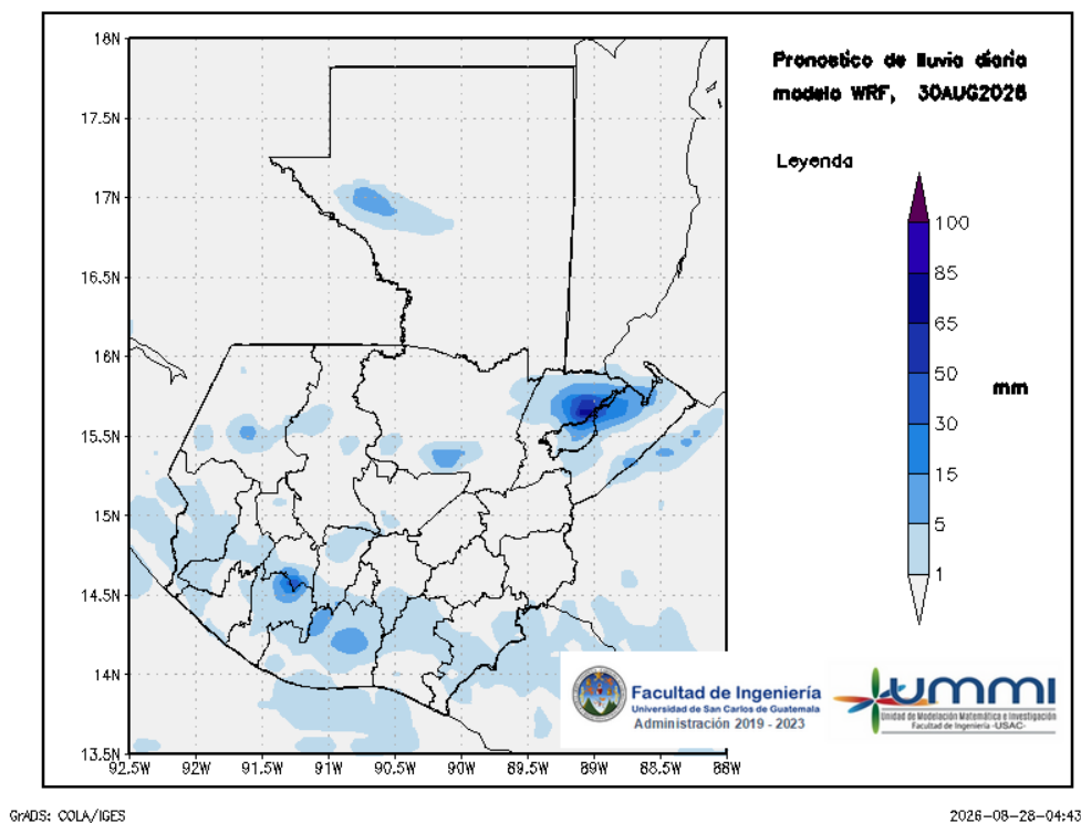
Figura 3: Pronóstico de lluvia diaria del 30 de August
