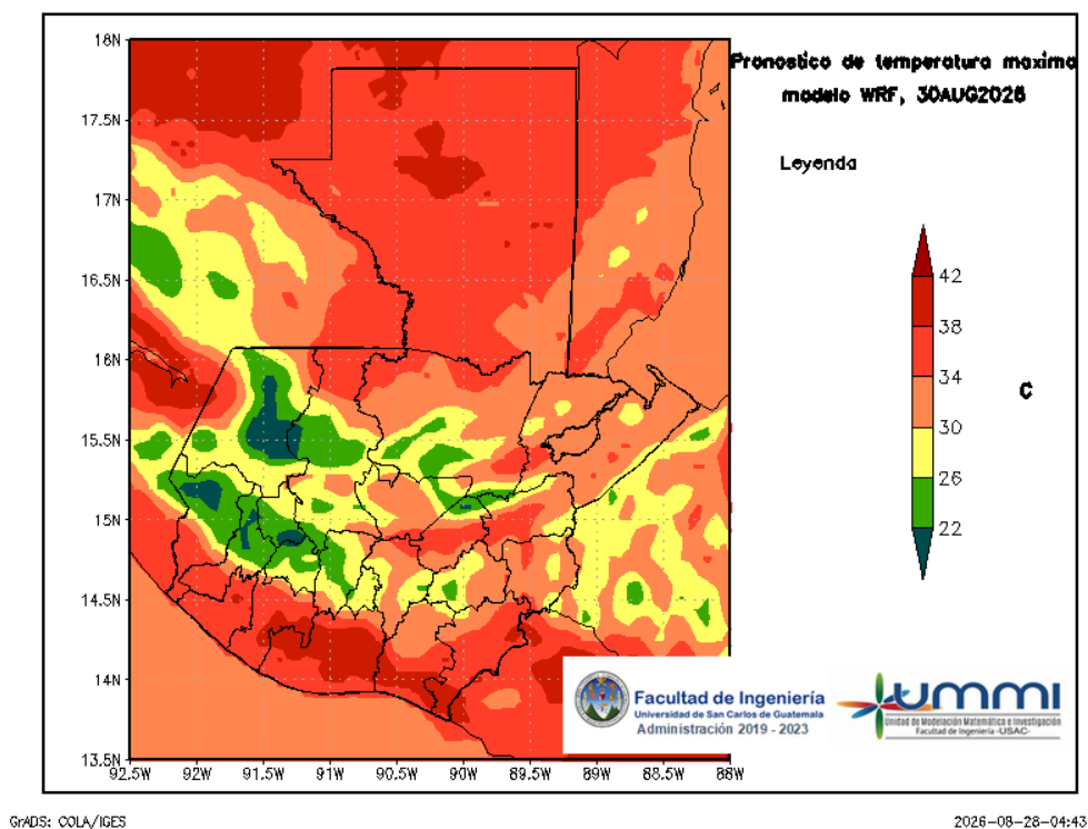
Figura 6: Pronóstico de temperatura máxima diaria del 30 de August
