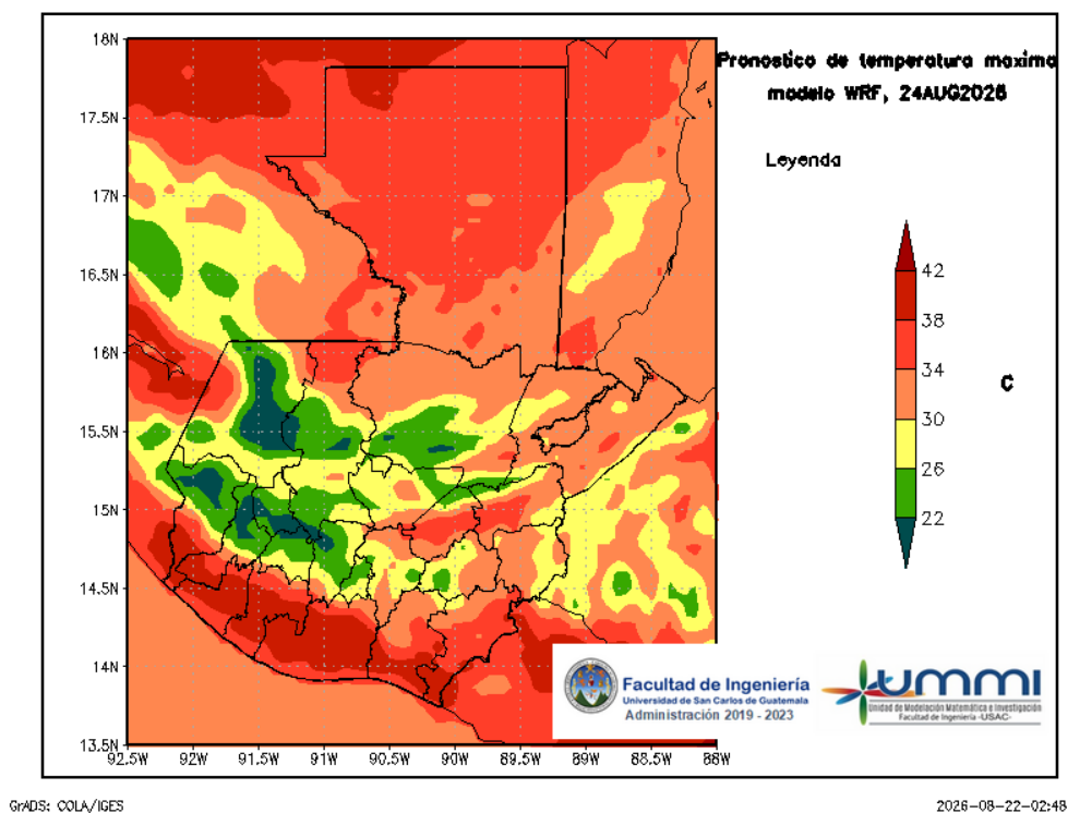
Figura 6: Pronóstico de temperatura máxima diaria del 24 de August
