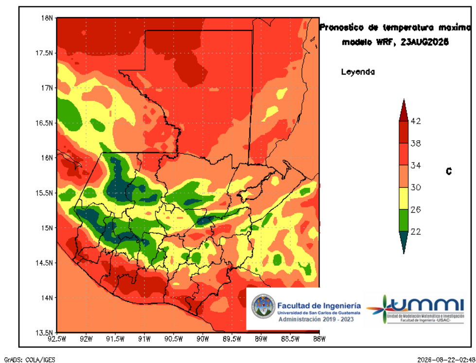
Figura 5: Pronóstico de temperatura máxima diaria del 23 de August
