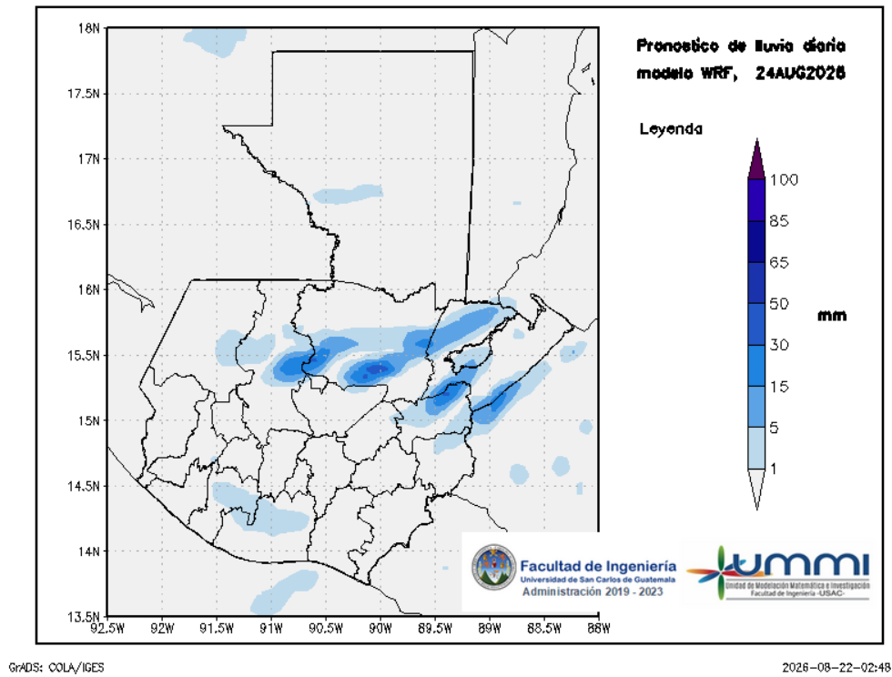
Figura 3: Pronóstico de lluvia diaria del 24 de August
