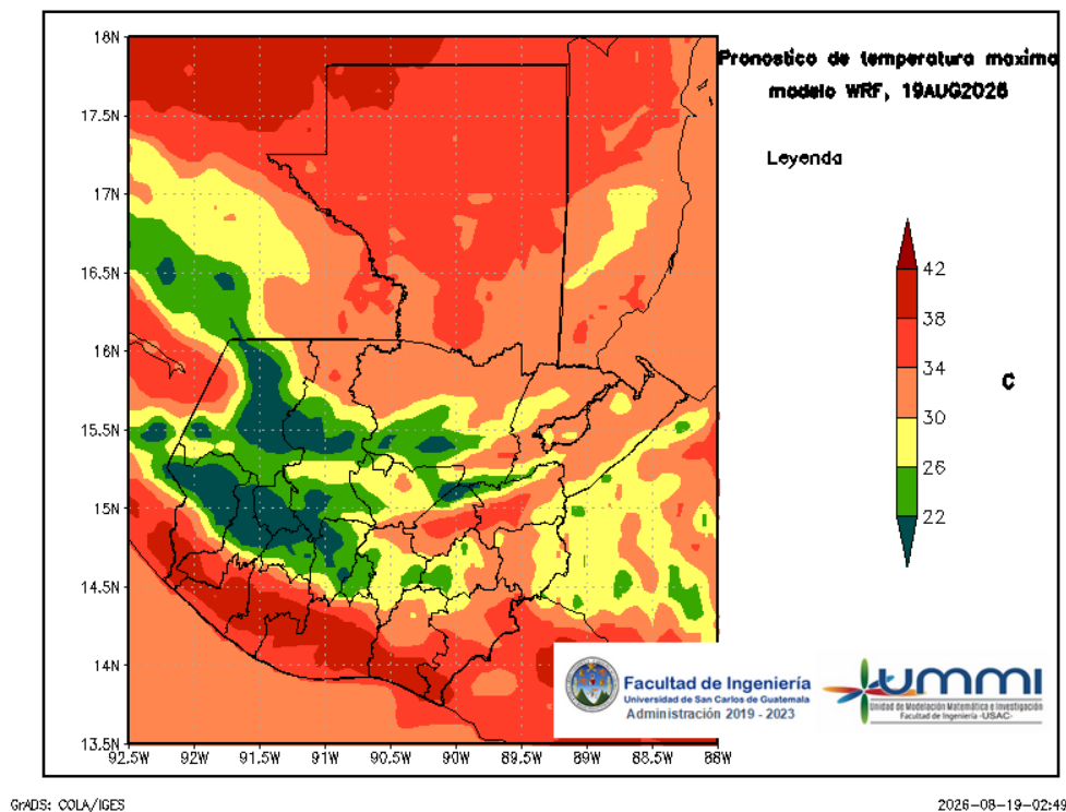
Figura 4: Pronóstico de temperatura máxima diaria del 19 de August
