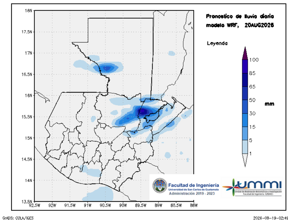
Figura 2: Pronóstico de lluvia diaria del 20 de August
