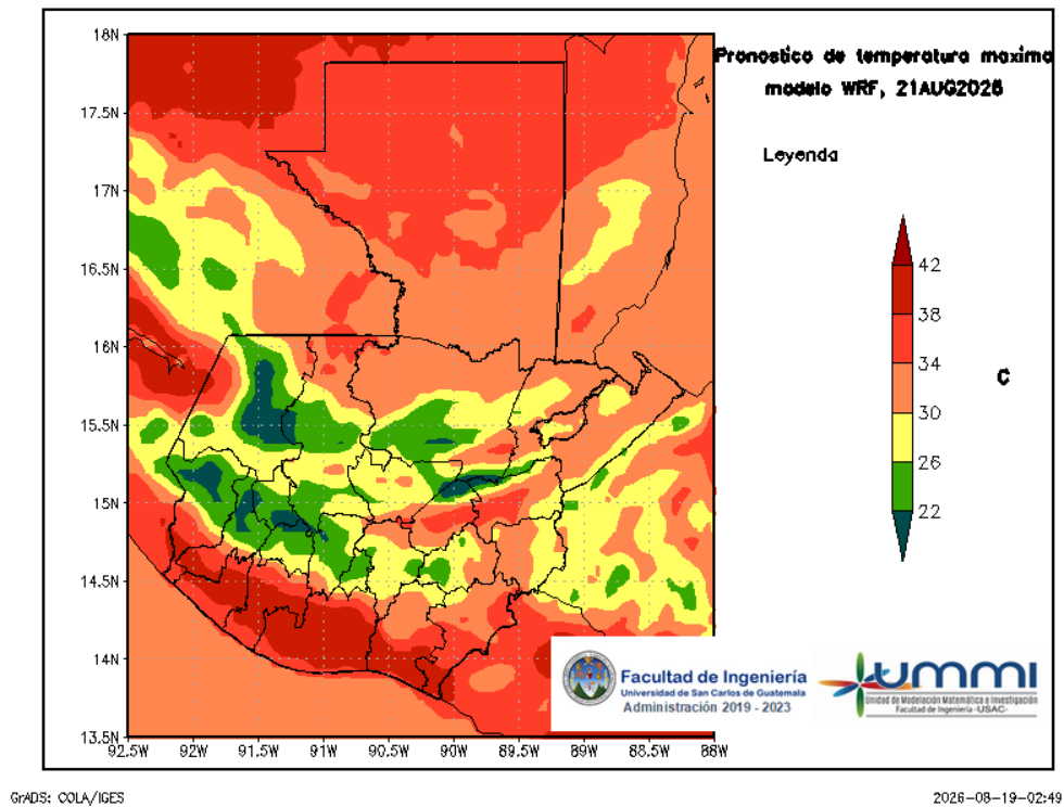
Figura 6: Pronóstico de temperatura máxima diaria del 21 de August
