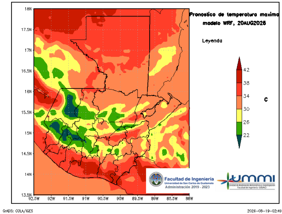
Figura 5: Pronóstico de temperatura máxima diaria del 20 de August
