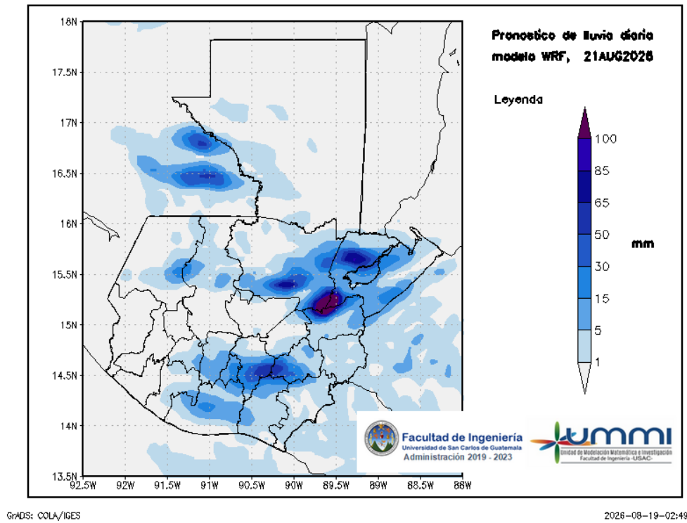
Figura 3: Pronóstico de lluvia diaria del 21 de August
