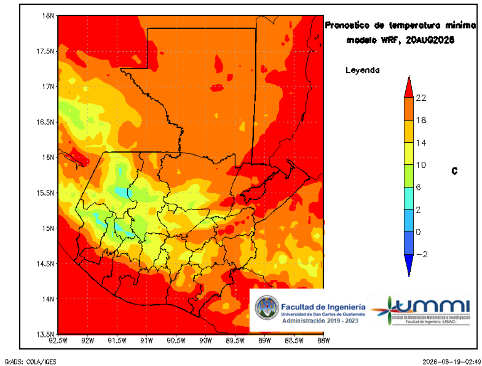
Figura 8: Pronóstico de temperatura mínima diaria del 21 de August
