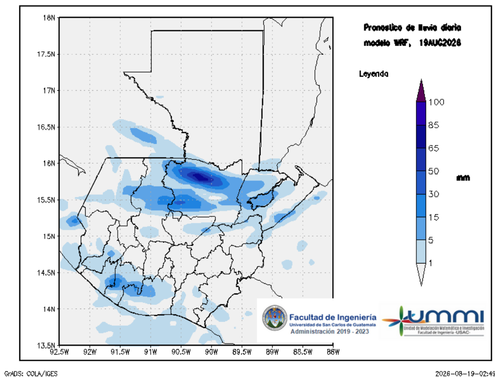
Figura 1: Pronóstico de lluvia diaria del 19 de August
