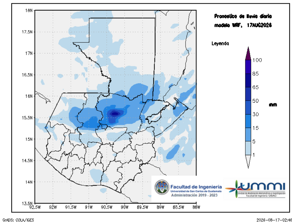
Figura 1: Pronóstico de lluvia diaria del 17 de August
