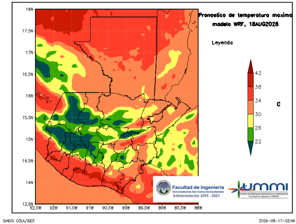
Figura 5: Pronóstico de temperatura máxima diaria del 18 de August
