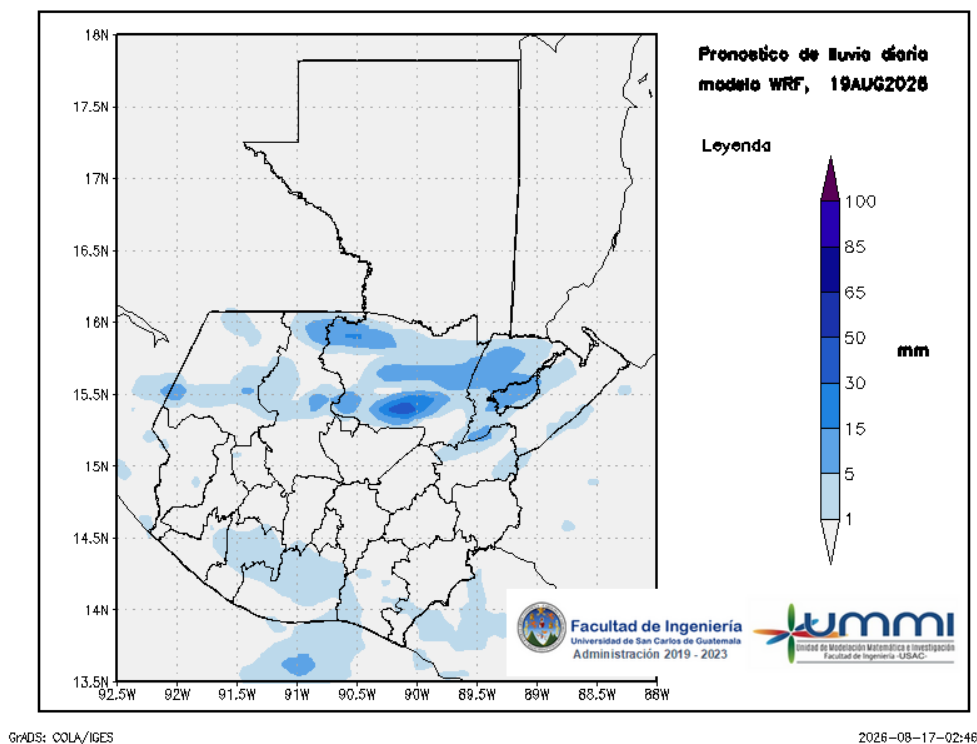
Figura 3: Pronóstico de lluvia diaria del 19 de August
