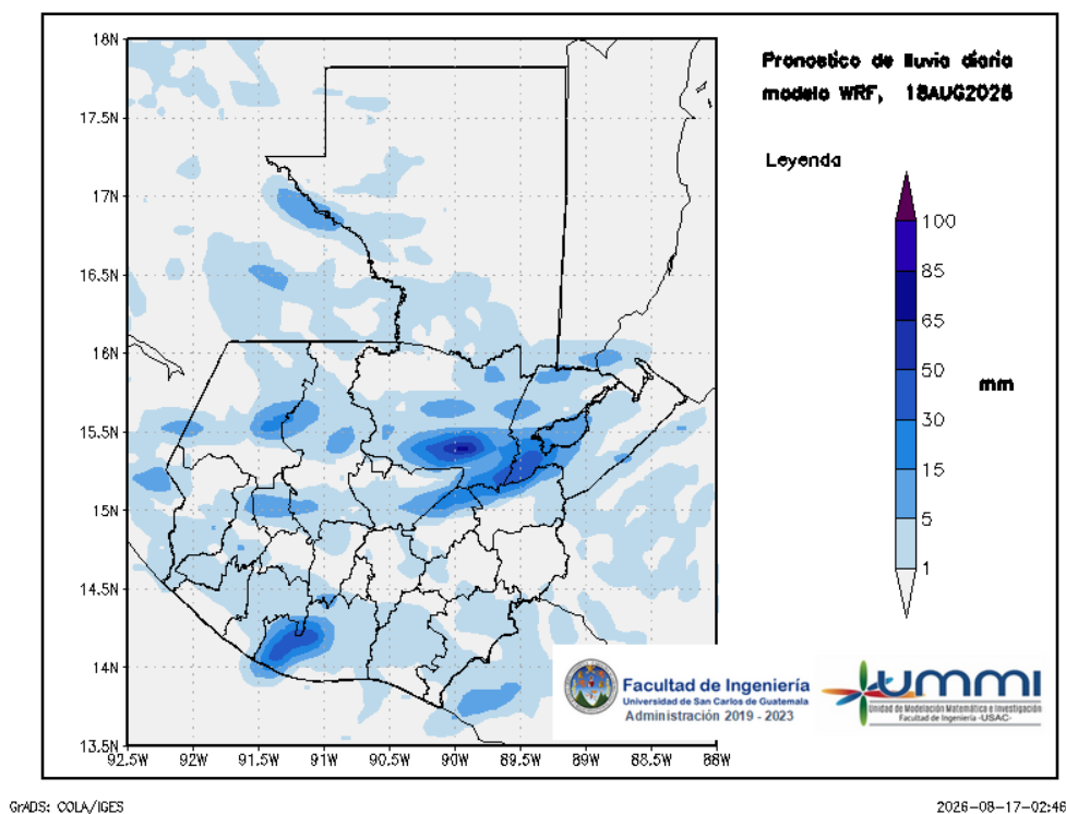
Figura 2: Pronóstico de lluvia diaria del 18 de August
