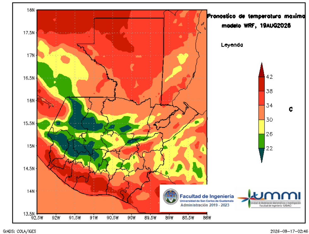
Figura 6: Pronóstico de temperatura máxima diaria del 19 de August
