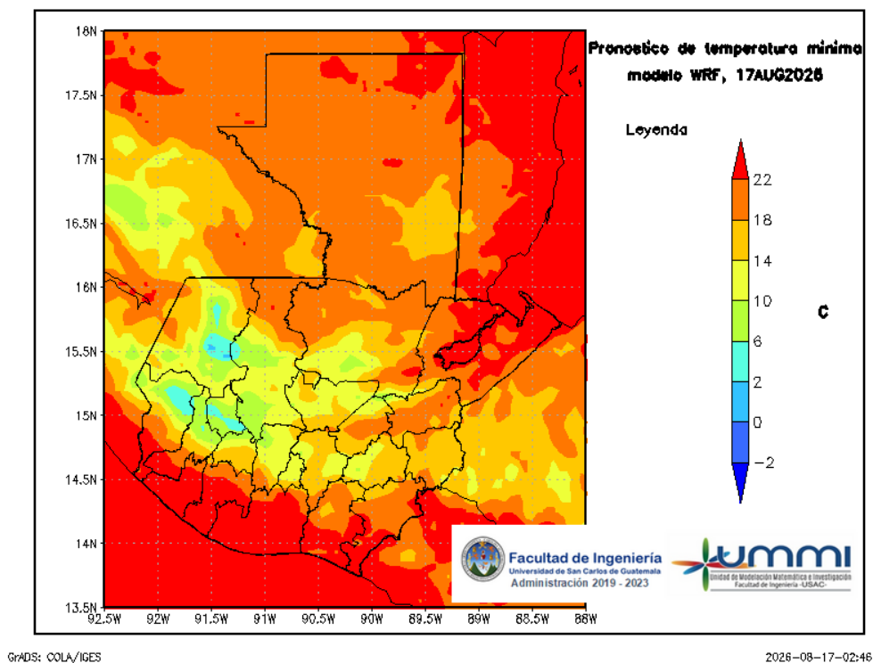
Figura 7: Pronóstico de temperatura mínima diaria del 18 de August
