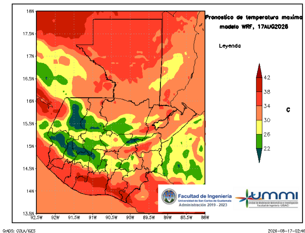
Figura 4: Pronóstico de temperatura máxima diaria del 17 de August
