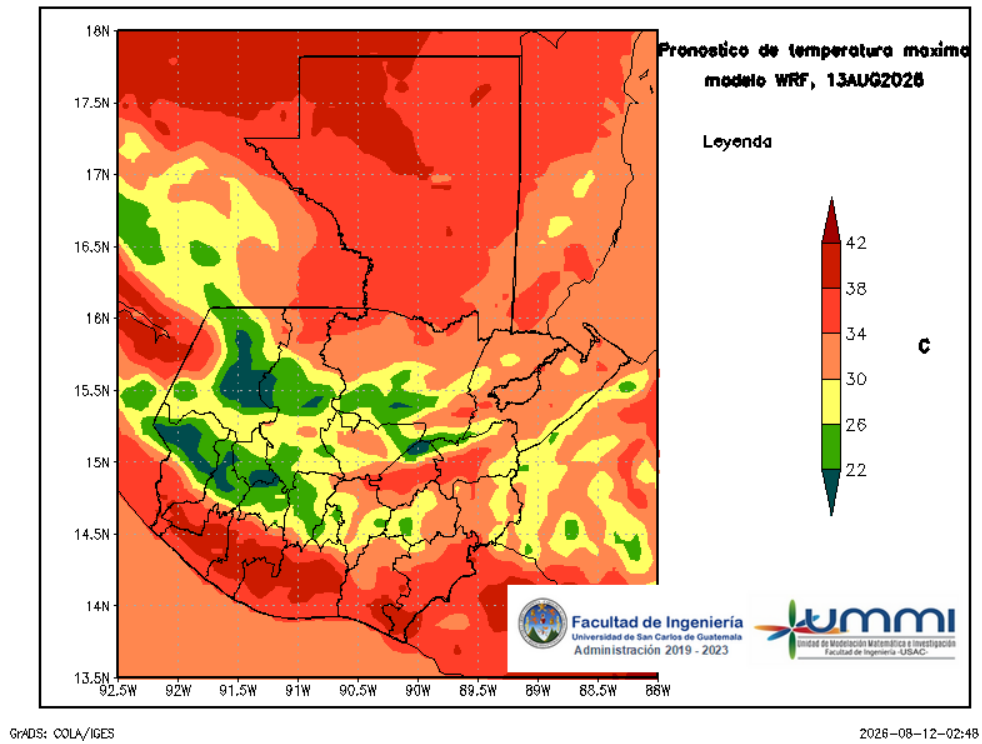
Figura 5: Pronóstico de temperatura máxima diaria del 13 de August
