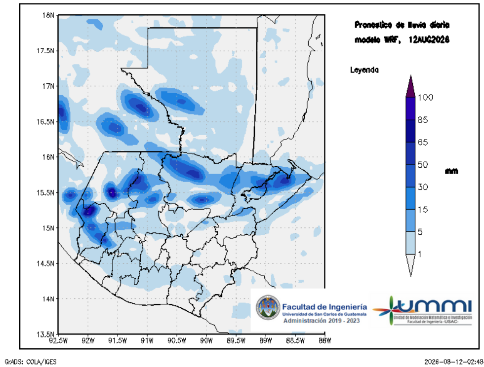
Figura 1: Pronóstico de lluvia diaria del 12 de August
