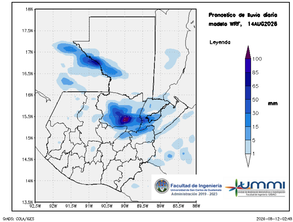
Figura 3: Pronóstico de lluvia diaria del 14 de August
