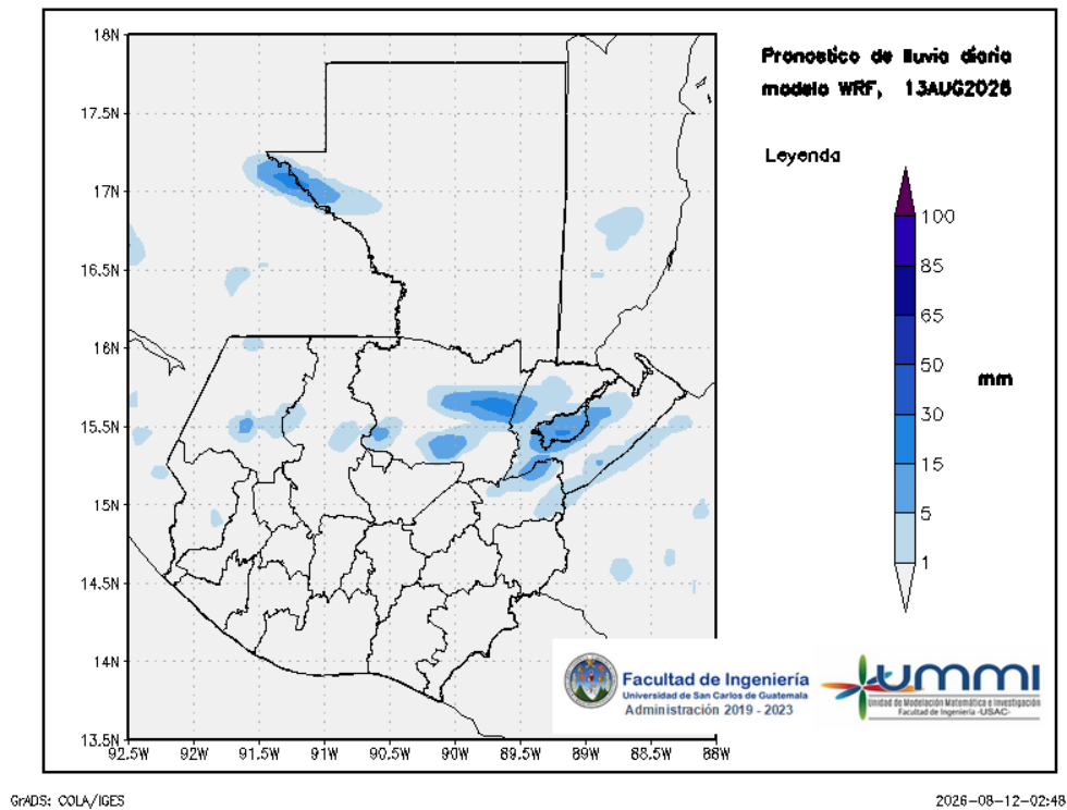
Figura 2: Pronóstico de lluvia diaria del 13 de August
