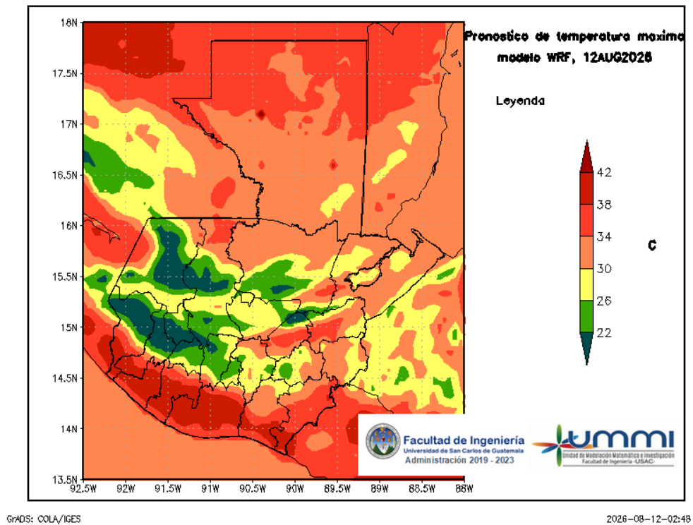
Figura 4: Pronóstico de temperatura máxima diaria del 12 de August
