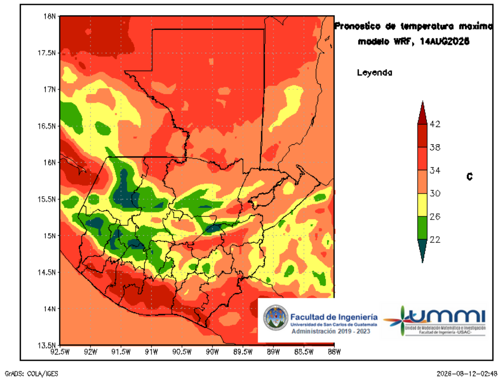
Figura 6: Pronóstico de temperatura máxima diaria del 14 de August
