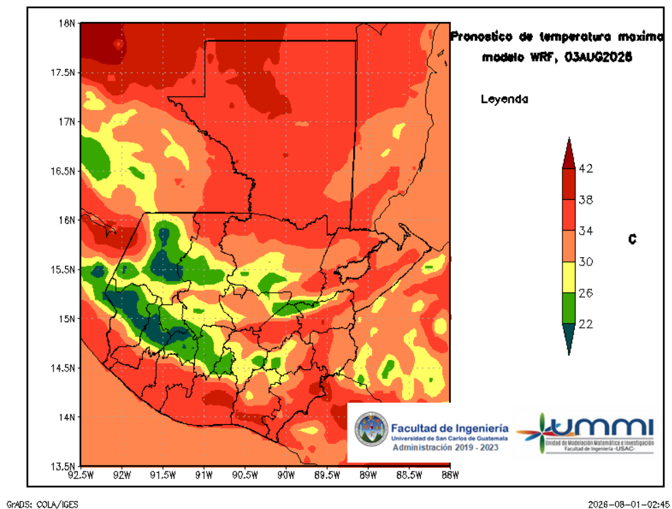
Figura 6: Pronóstico de temperatura máxima diaria del 03 de August
