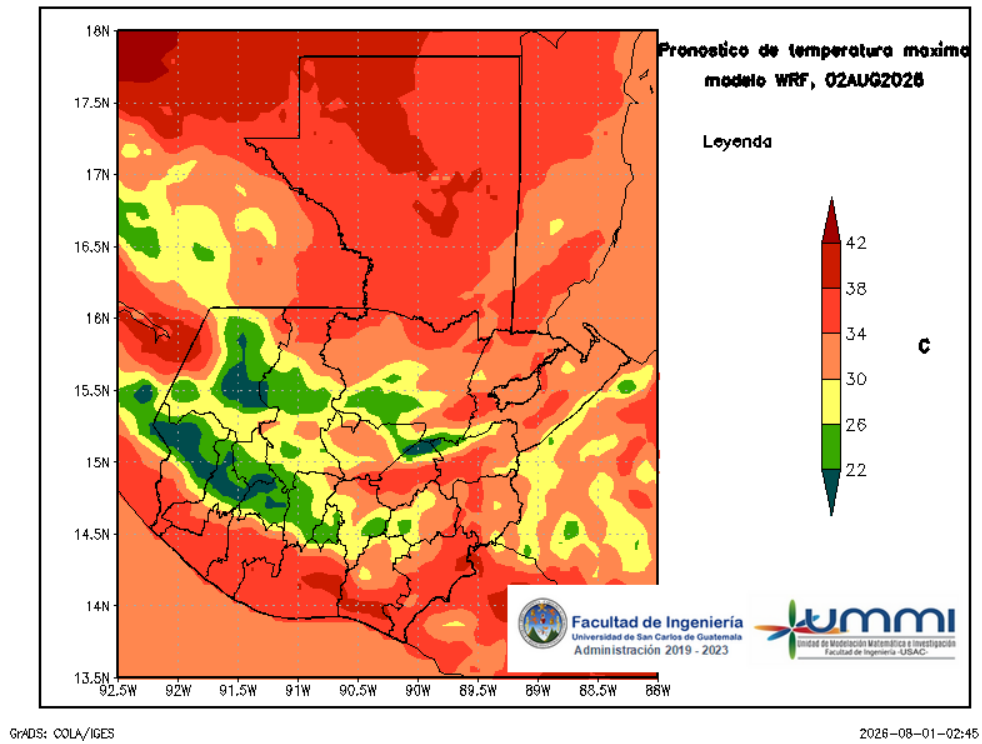
Figura 5: Pronóstico de temperatura máxima diaria del 02 de August
