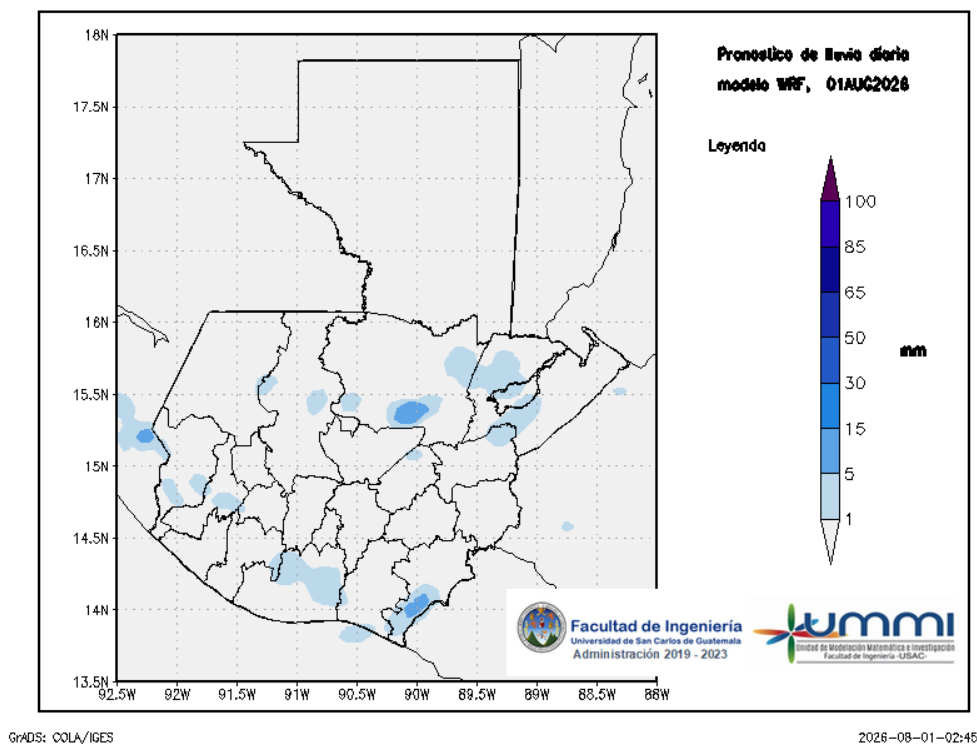
Figura 1: Pronóstico de lluvia diaria del 01 de August
