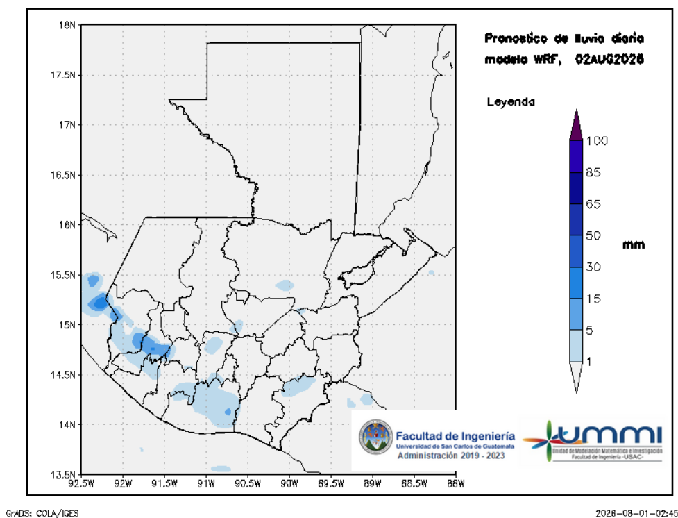
Figura 2: Pronóstico de lluvia diaria del 02 de August
