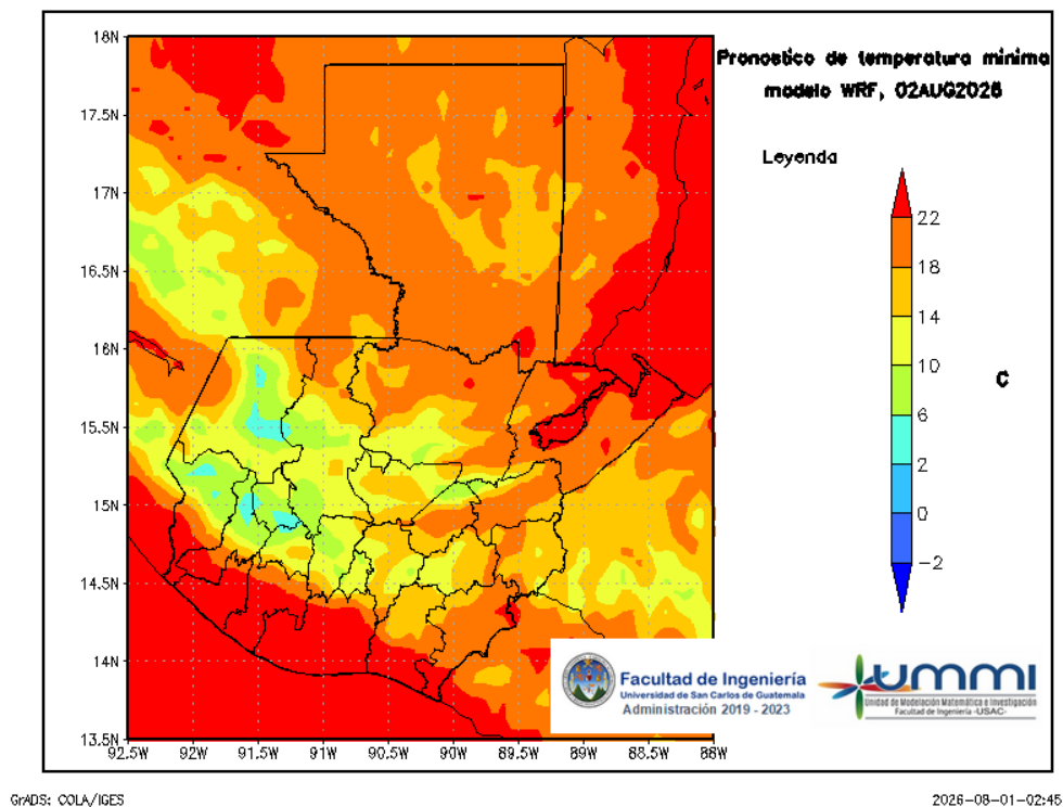
Figura 8: Pronóstico de temperatura mínima diaria del 03 de August
