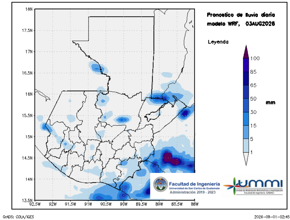
Figura 3: Pronóstico de lluvia diaria del 03 de August
