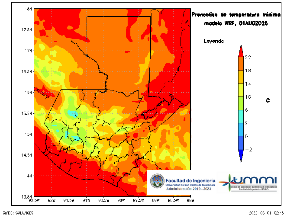
Figura 7: Pronóstico de temperatura mínima diaria del 02 de August
