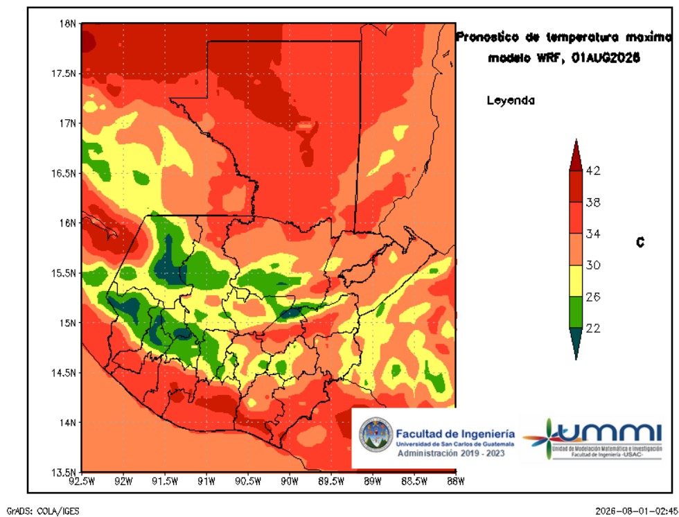
Figura 4: Pronóstico de temperatura máxima diaria del 01 de August
