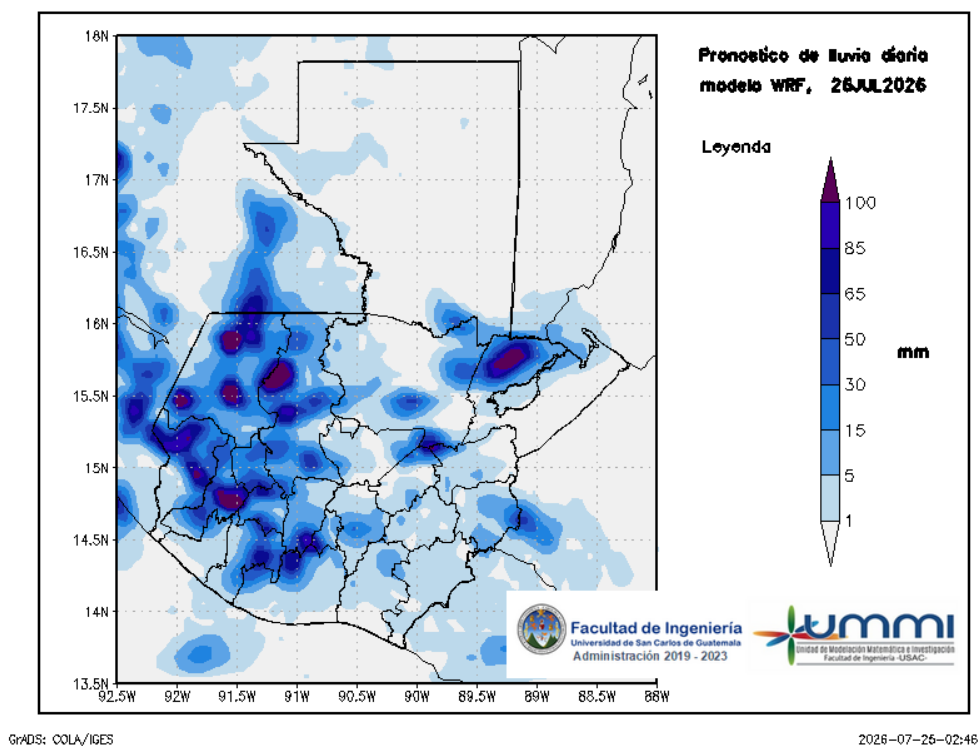
Figura 2: Pronóstico de lluvia diaria del 26 de July
