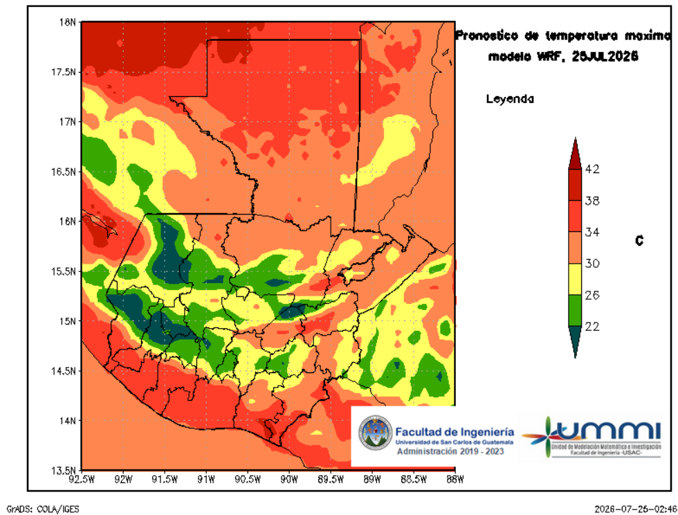
Figura 4: Pronóstico de temperatura máxima diaria del 25 de July
