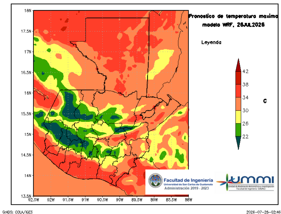
Figura 5: Pronóstico de temperatura máxima diaria del 26 de July
