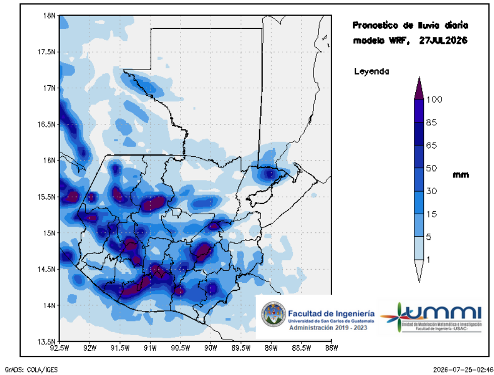
Figura 3: Pronóstico de lluvia diaria del 27 de July
