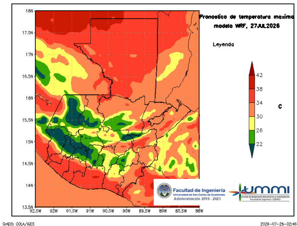
Figura 6: Pronóstico de temperatura máxima diaria del 27 de July
