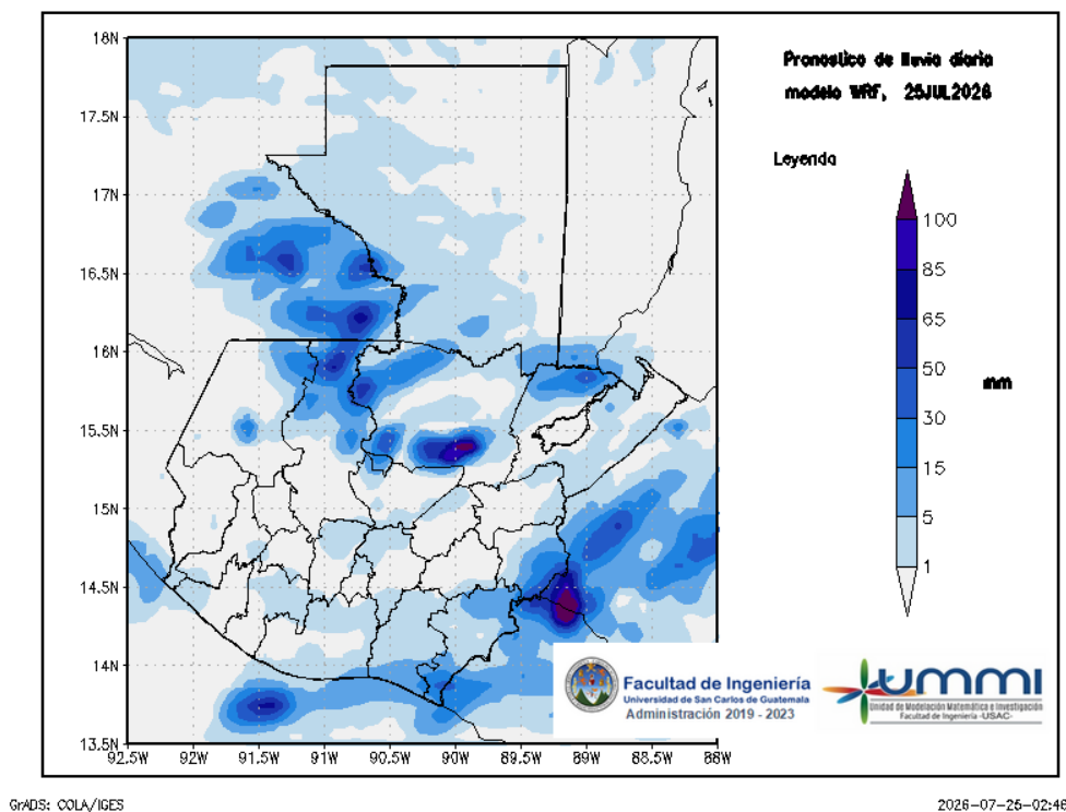
Figura 1: Pronóstico de lluvia diaria del 25 de July
