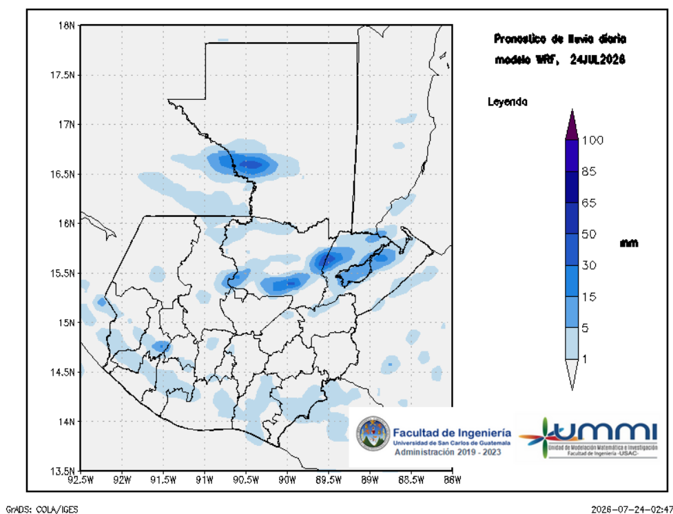
Figura 1: Pronóstico de lluvia diaria del 24 de July
