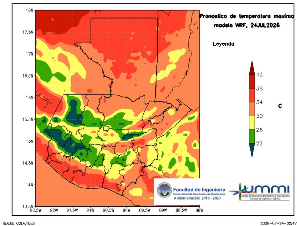
Figura 4: Pronóstico de temperatura máxima diaria del 24 de July
