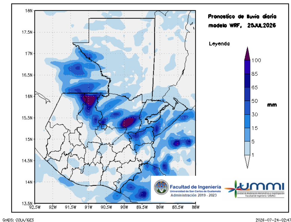
Figura 2: Pronóstico de lluvia diaria del 25 de July
