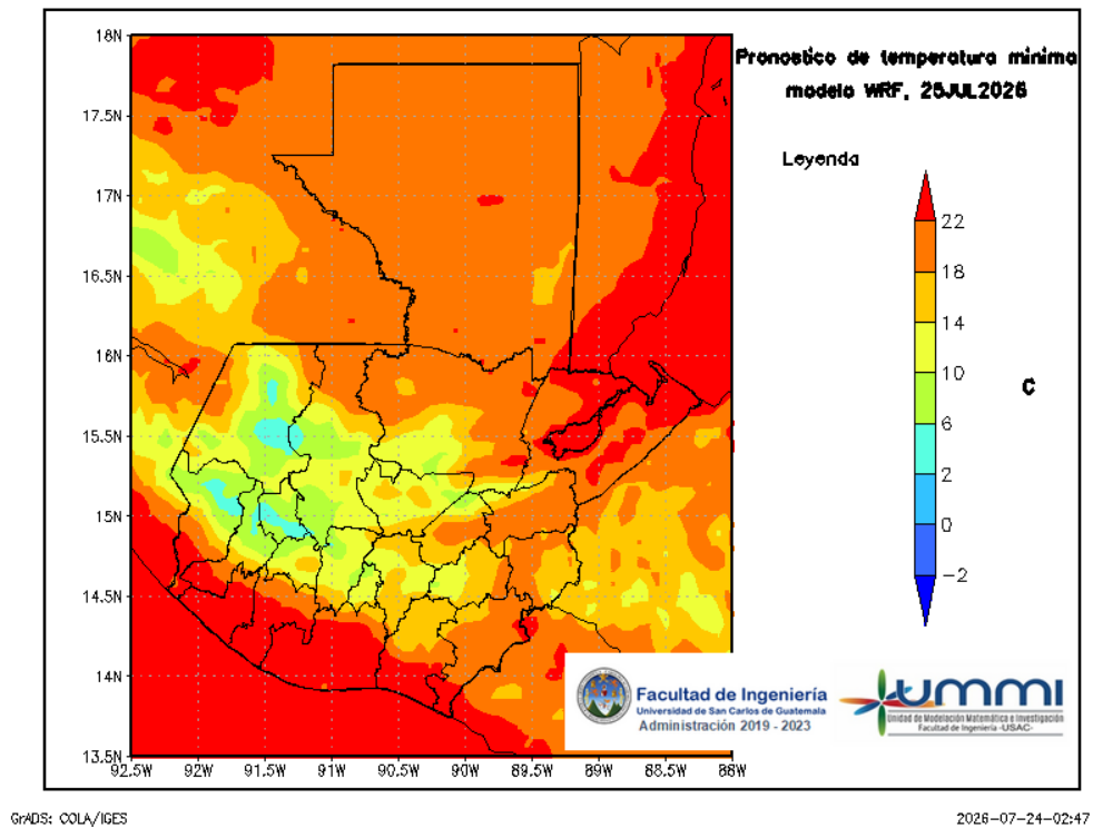
Figura 8: Pronóstico de temperatura mínima diaria del 26 de July
