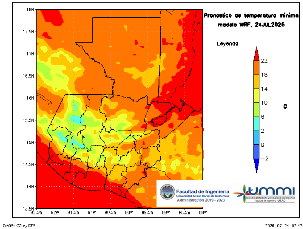
Figura 7: Pronóstico de temperatura mínima diaria del 25 de July
