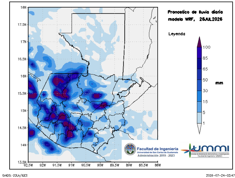
Figura 3: Pronóstico de lluvia diaria del 26 de July
