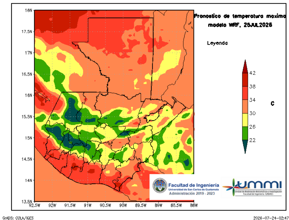
Figura 5: Pronóstico de temperatura máxima diaria del 25 de July
