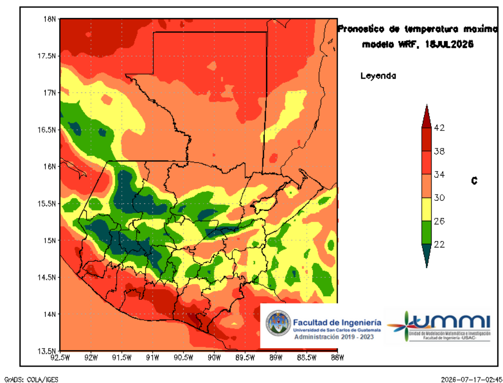
Figura 5: Pronóstico de temperatura máxima diaria del 18 de July
