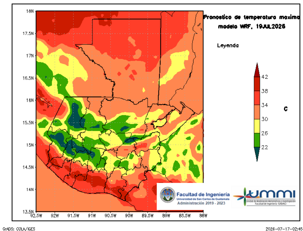
Figura 6: Pronóstico de temperatura máxima diaria del 19 de July
