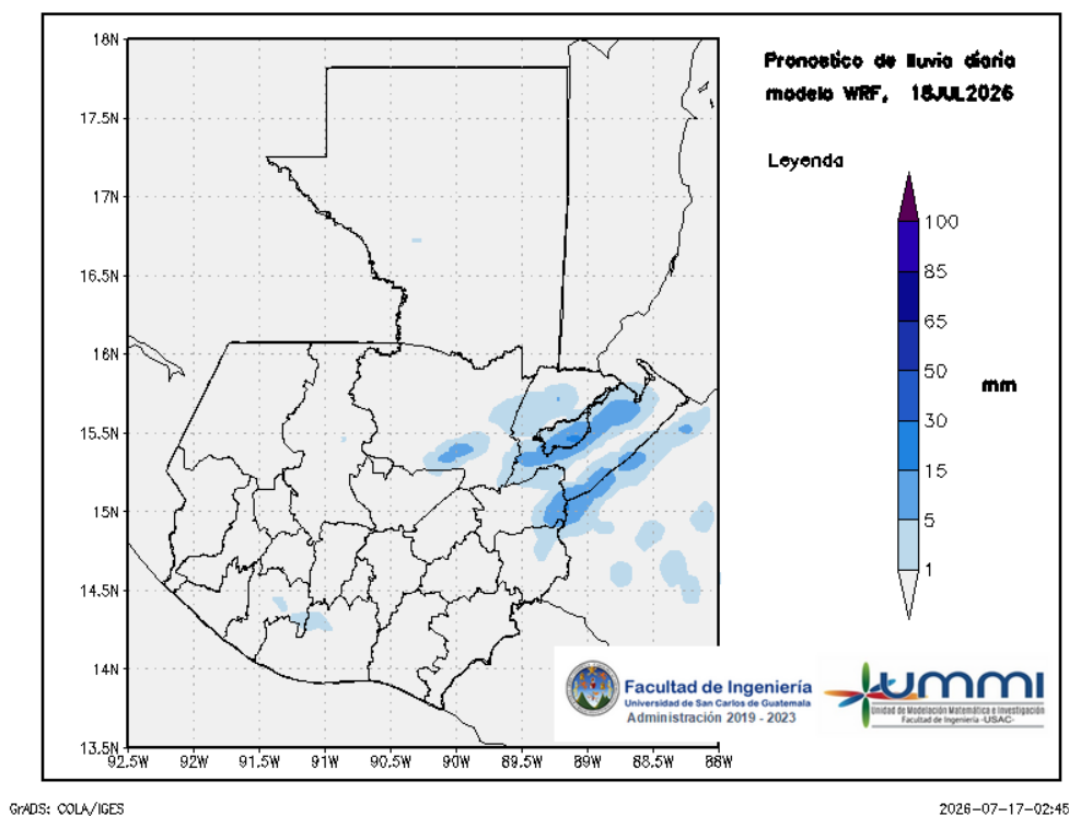
Figura 2: Pronóstico de lluvia diaria del 18 de July
