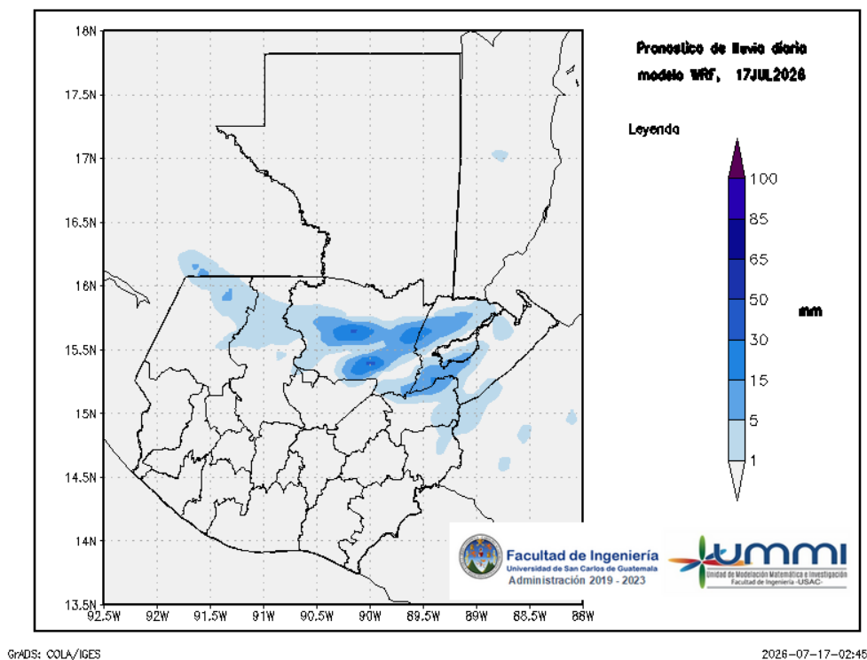
Figura 1: Pronóstico de lluvia diaria del 17 de July
