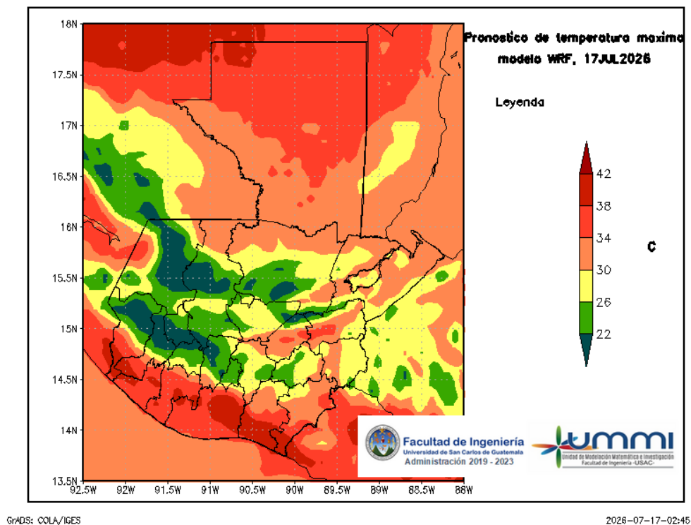
Figura 4: Pronóstico de temperatura máxima diaria del 17 de July
