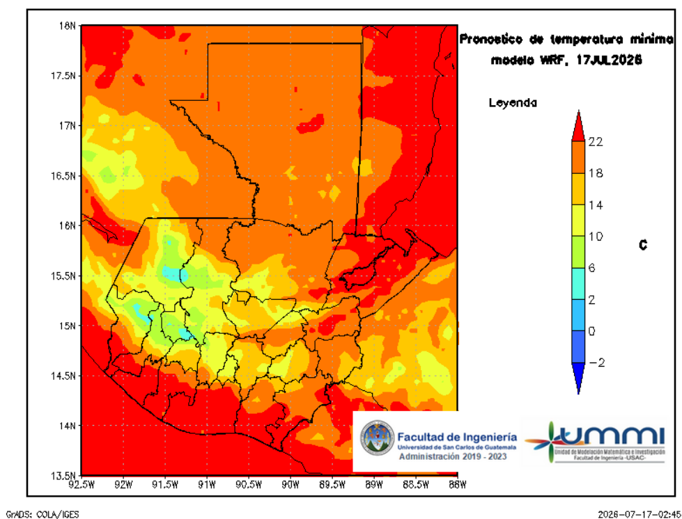
Figura 7: Pronóstico de temperatura mínima diaria del 18 de July
