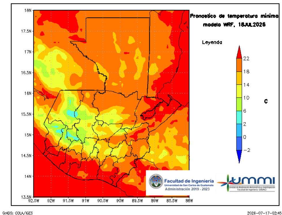
Figura 8: Pronóstico de temperatura mínima diaria del 19 de July
