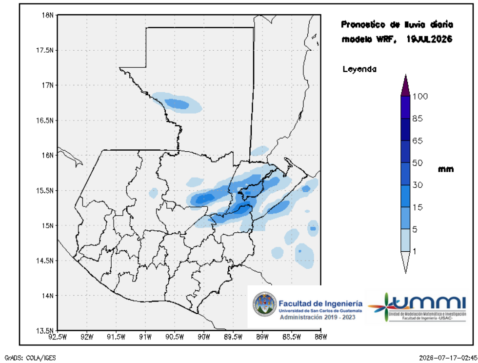
Figura 3: Pronóstico de lluvia diaria del 19 de July
