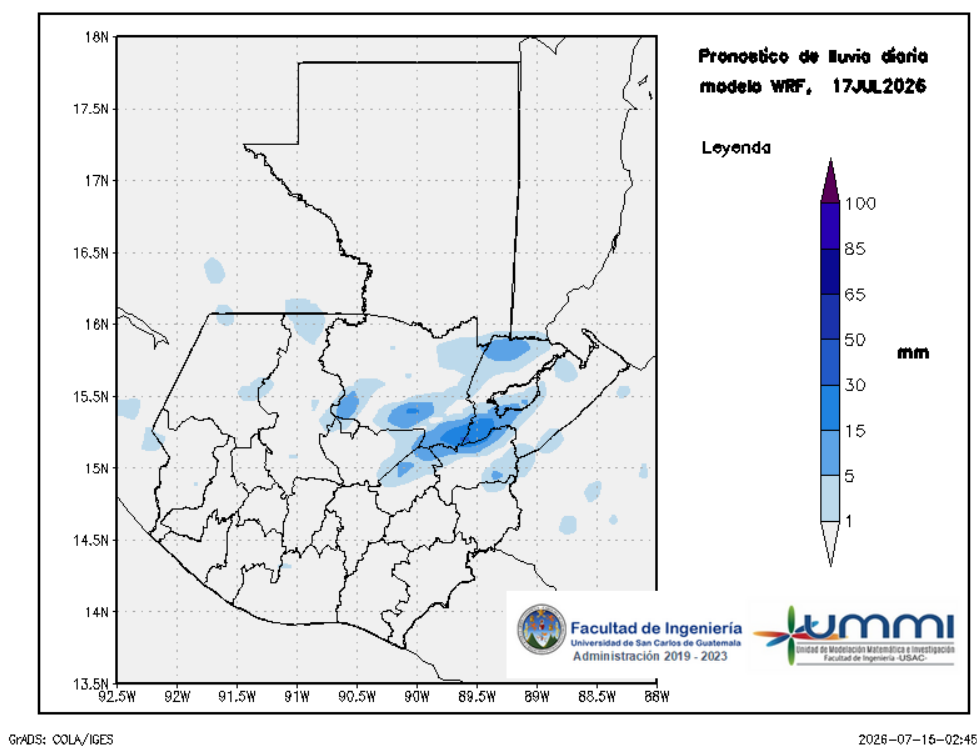
Figura 3: Pronóstico de lluvia diaria del 17 de July
