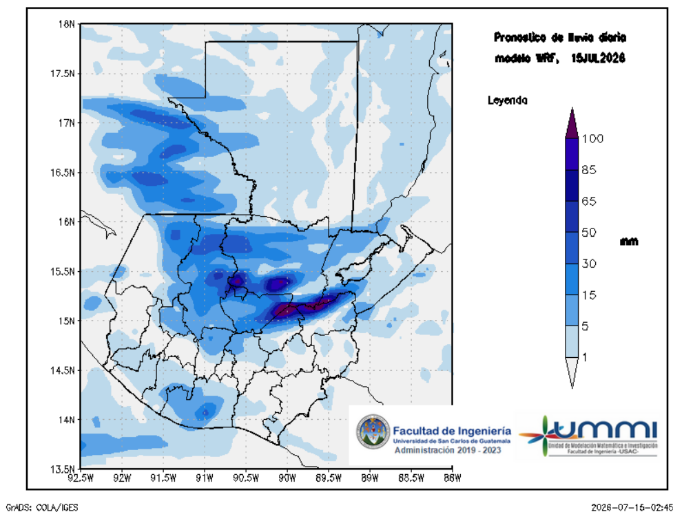
Figura 1: Pronóstico de lluvia diaria del 15 de July
