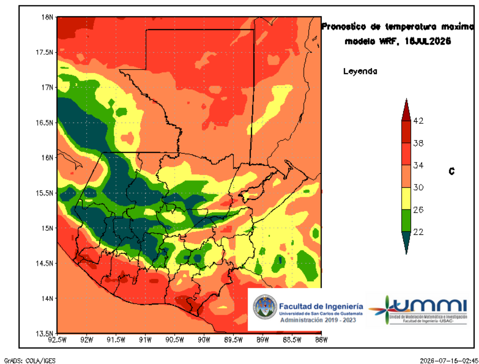
Figura 5: Pronóstico de temperatura máxima diaria del 16 de July
