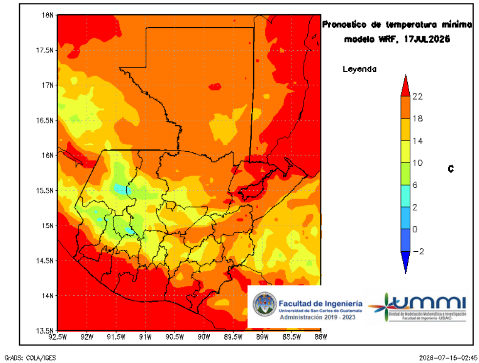
Figura 9: Pronóstico de temperatura mínima diaria del 18 de July
