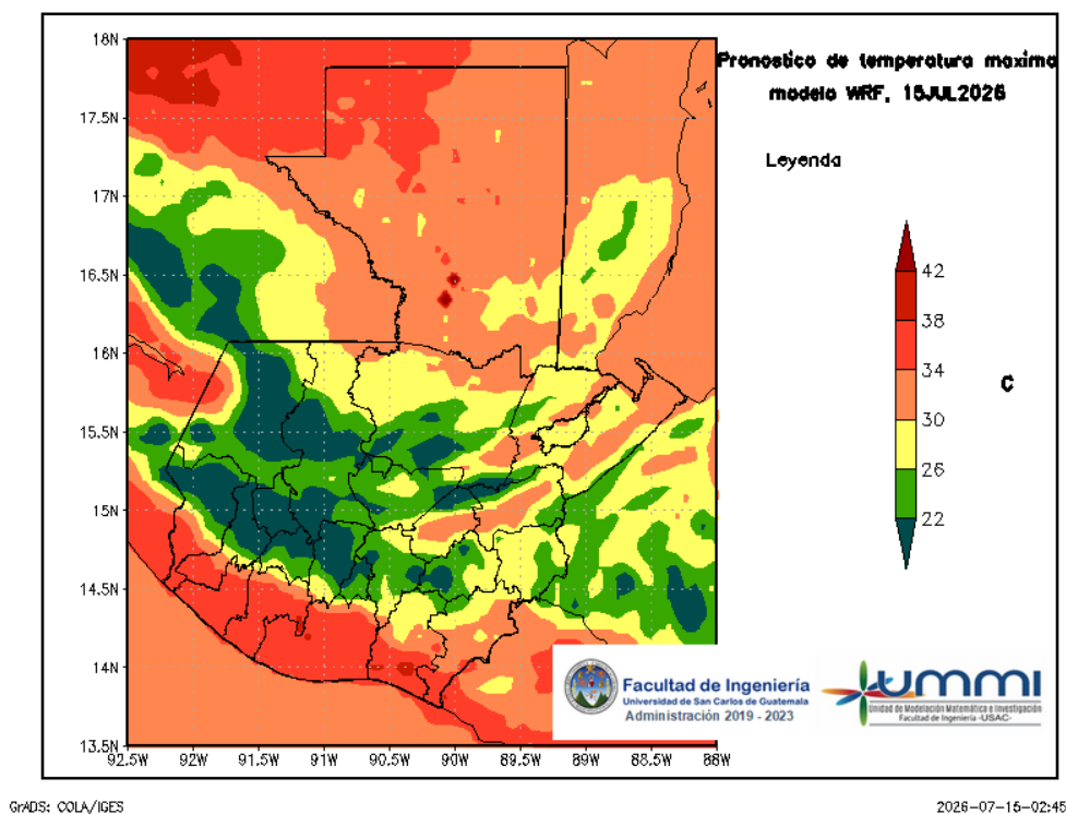
Figura 4: Pronóstico de temperatura máxima diaria del 15 de July
