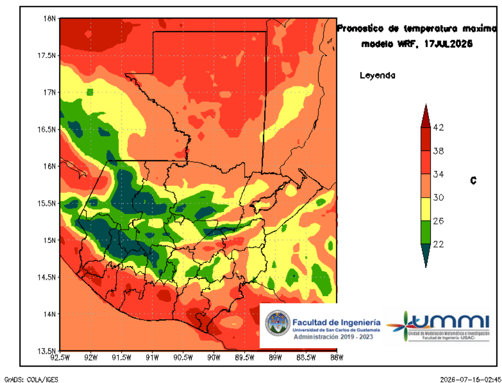
Figura 6: Pronóstico de temperatura máxima diaria del 17 de July
