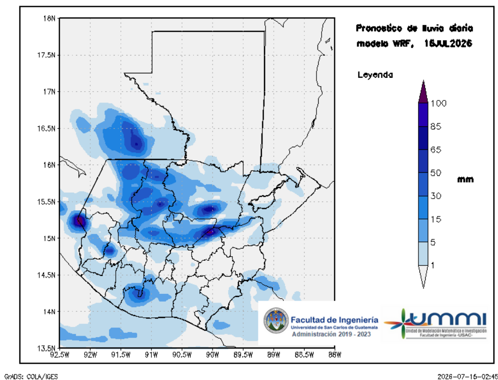
Figura 2: Pronóstico de lluvia diaria del 16 de July
