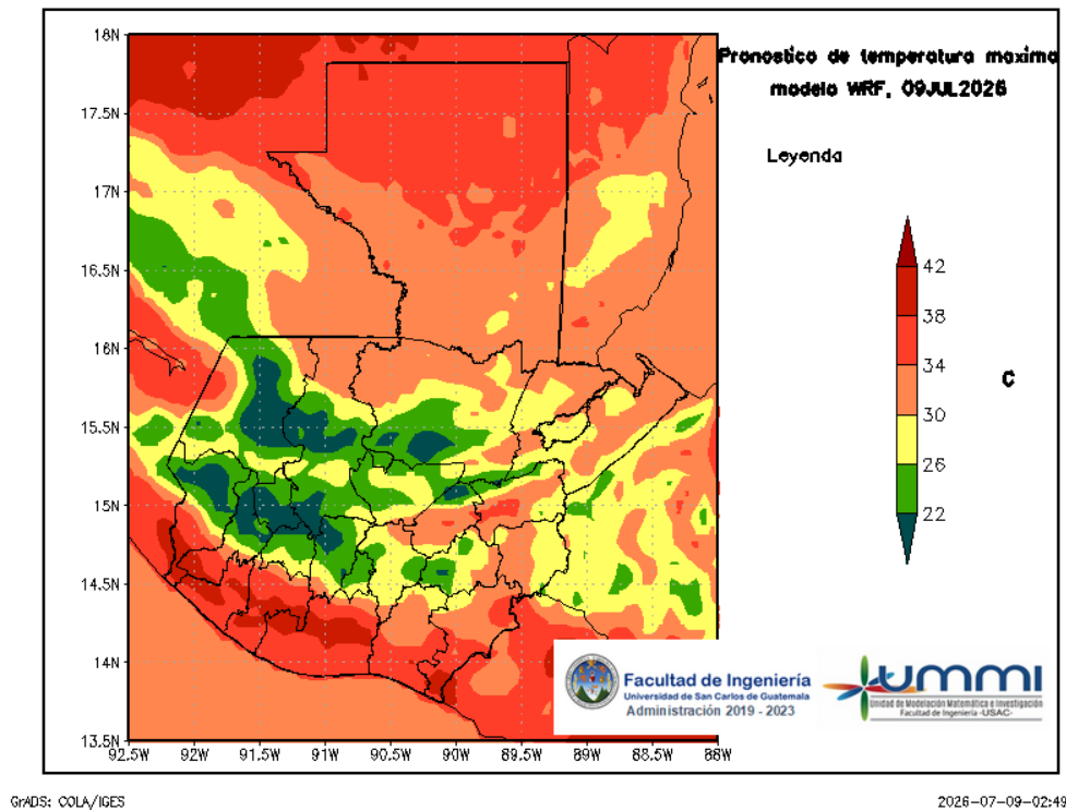
Figura 4: Pronóstico de temperatura máxima diaria del 09 de July
