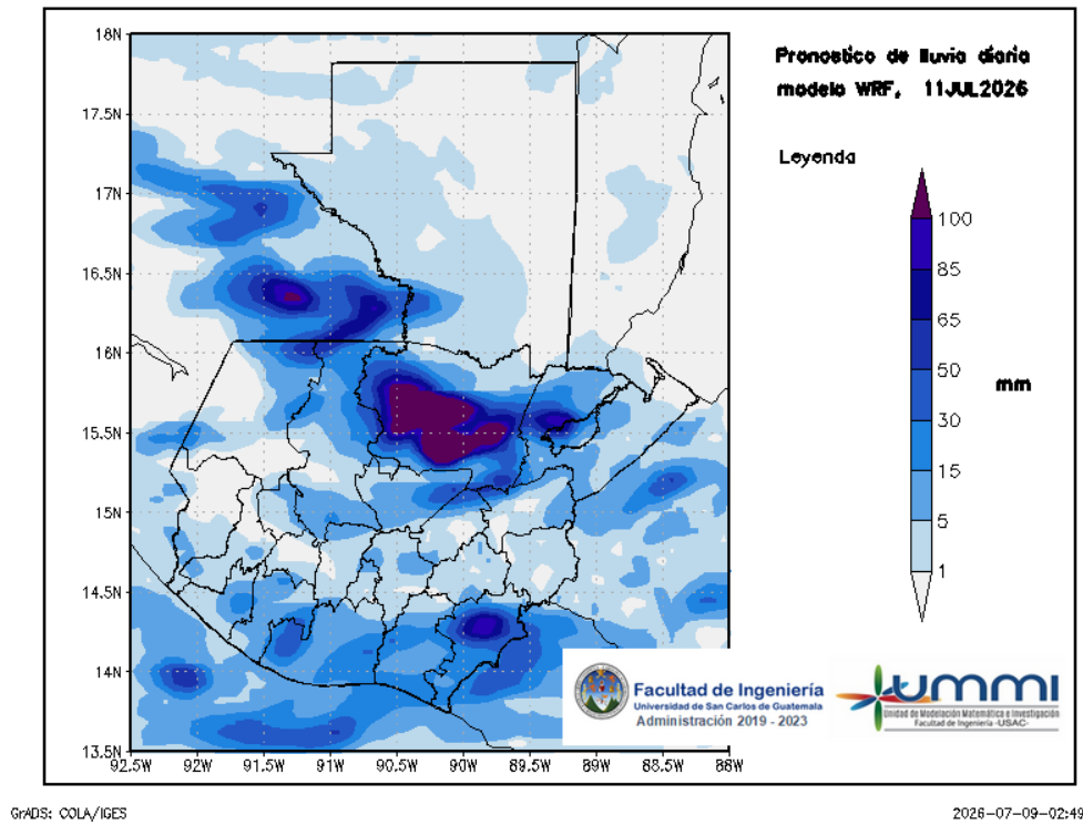
Figura 3: Pronóstico de lluvia diaria del 11 de July
