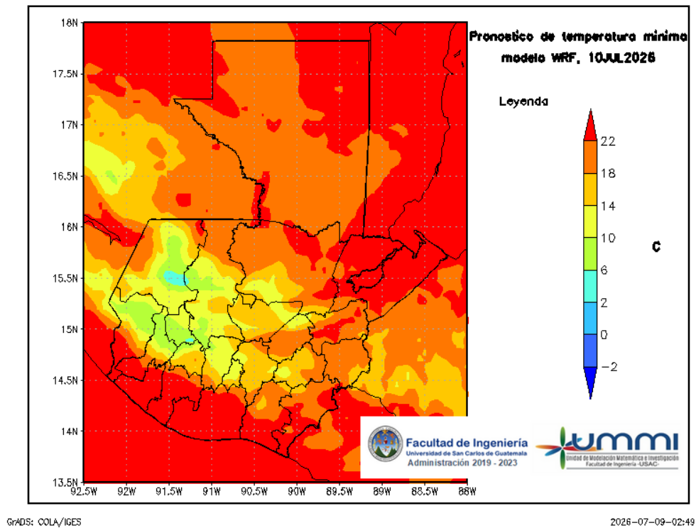
Figura 8: Pronóstico de temperatura mínima diaria del 11 de July
