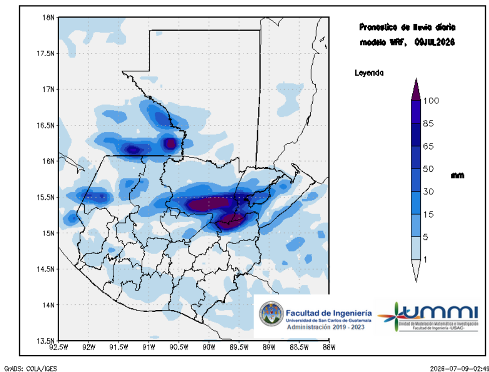
Figura 1: Pronóstico de lluvia diaria del 09 de July
