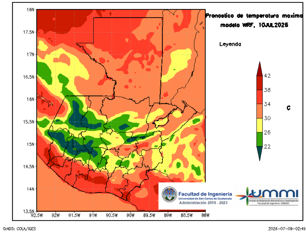
Figura 5: Pronóstico de temperatura máxima diaria del 10 de July
