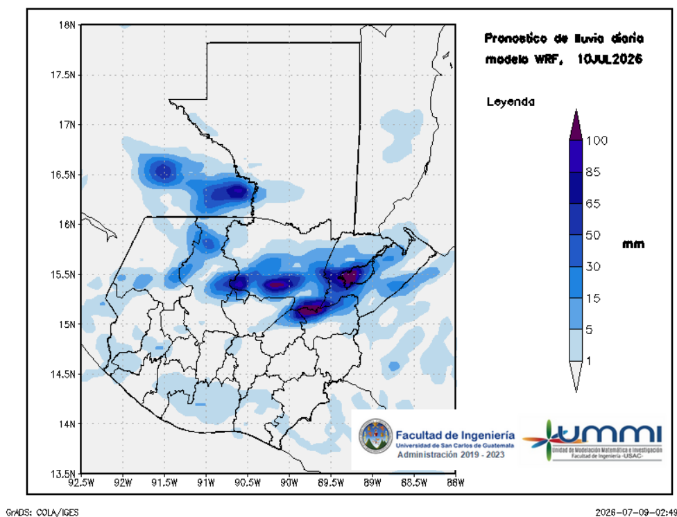
Figura 2: Pronóstico de lluvia diaria del 10 de July
