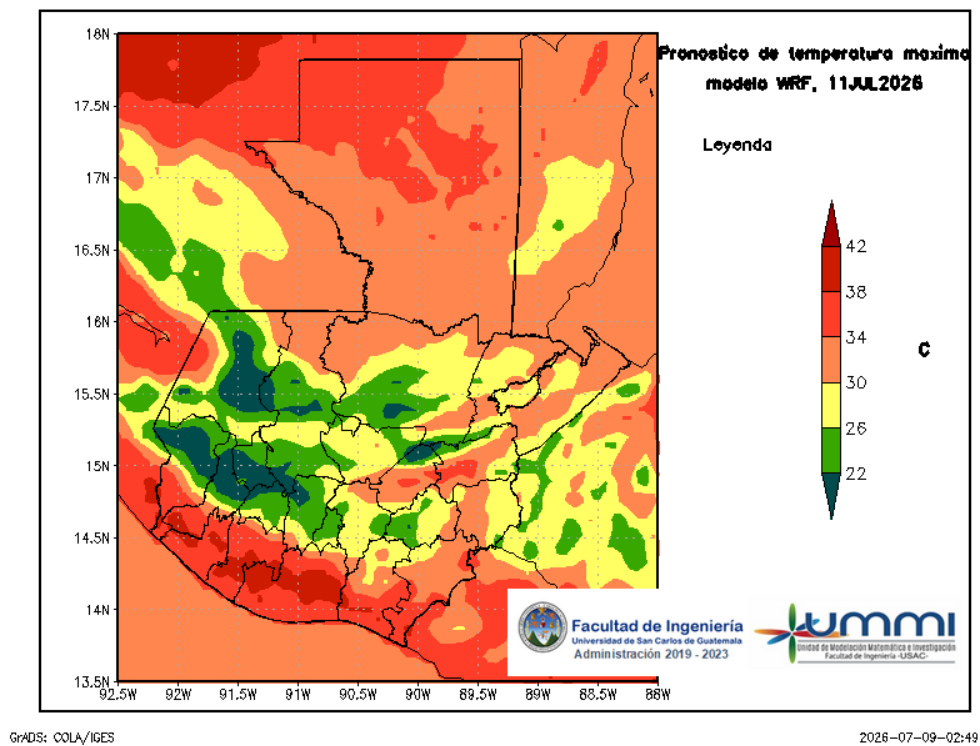
Figura 6: Pronóstico de temperatura máxima diaria del 11 de July
