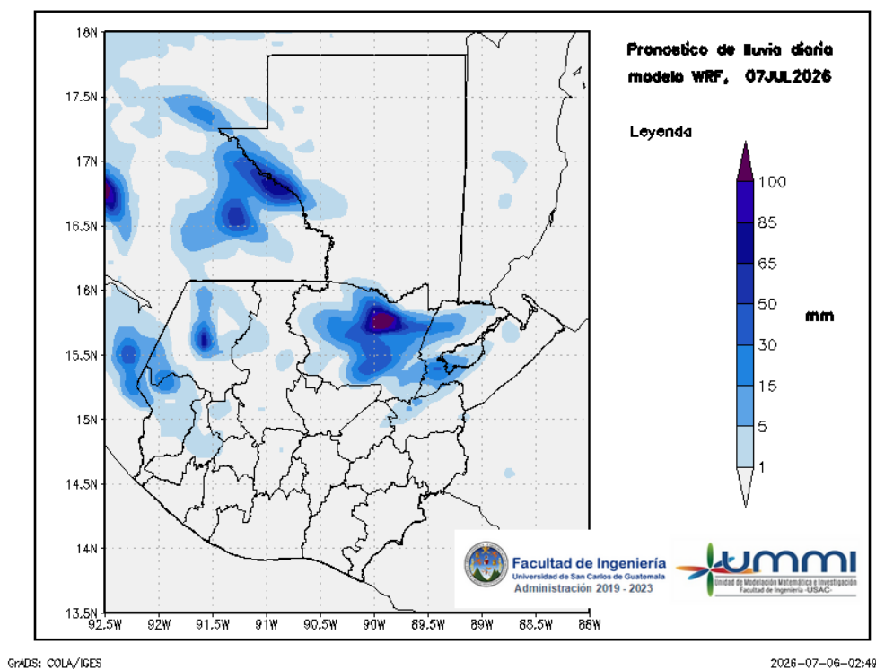
Figura 2: Pronóstico de lluvia diaria del 07 de July
