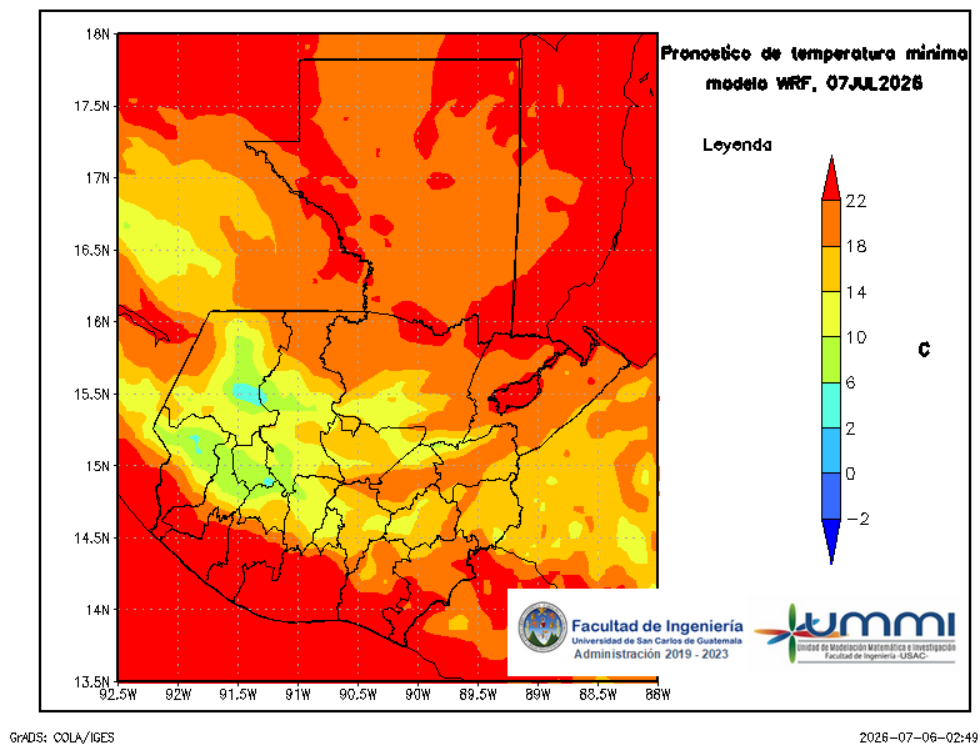
Figura 8: Pronóstico de temperatura mínima diaria del 08 de July
