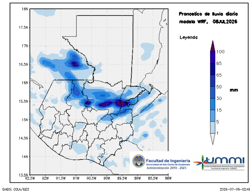
Figura 3: Pronóstico de lluvia diaria del 08 de July
