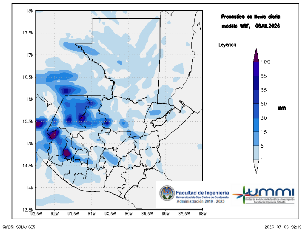
Figura 1: Pronóstico de lluvia diaria del 06 de July
