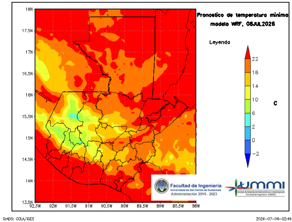
Figura 9: Pronóstico de temperatura mínima diaria del 09 de July
