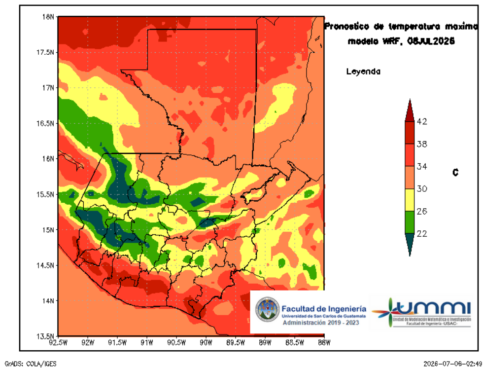
Figura 6: Pronóstico de temperatura máxima diaria del 08 de July
