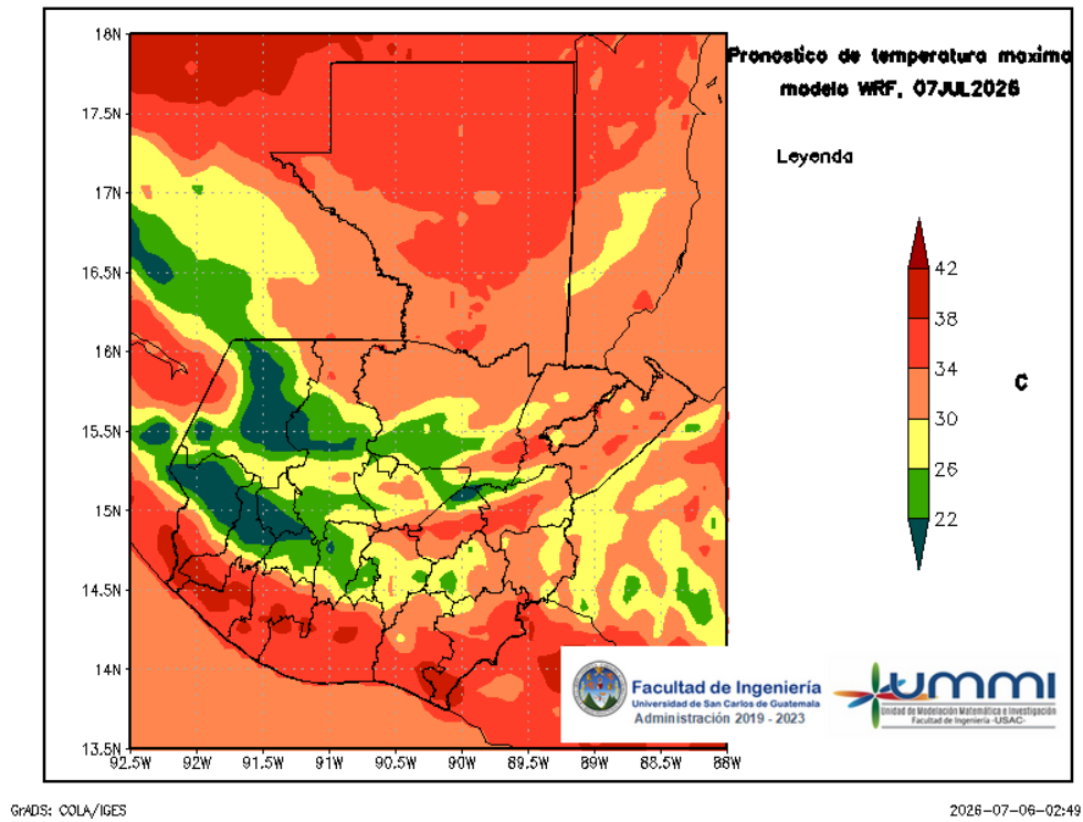
Figura 5: Pronóstico de temperatura máxima diaria del 07 de July
