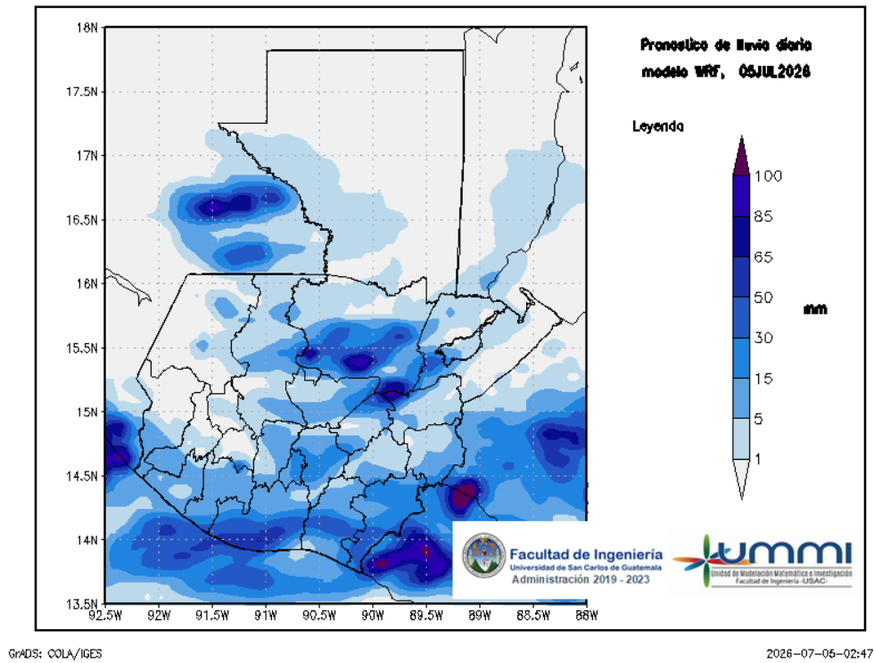
Figura 1: Pronóstico de lluvia diaria del 05 de July
