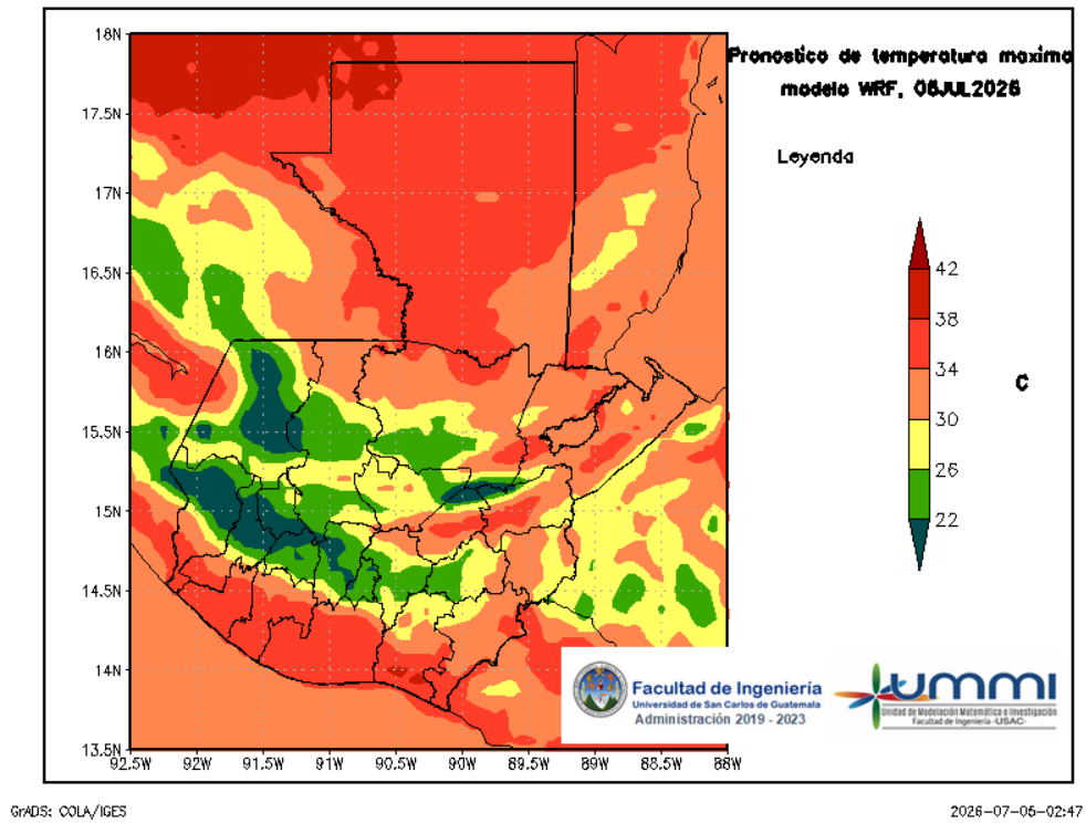
Figura 5: Pronóstico de temperatura máxima diaria del 06 de July
