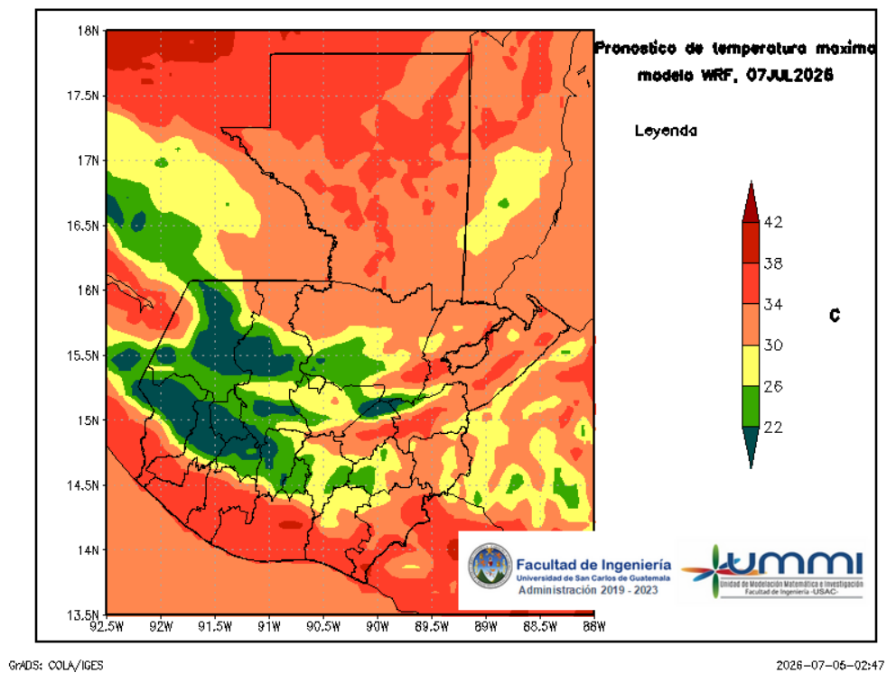
Figura 6: Pronóstico de temperatura máxima diaria del 07 de July
