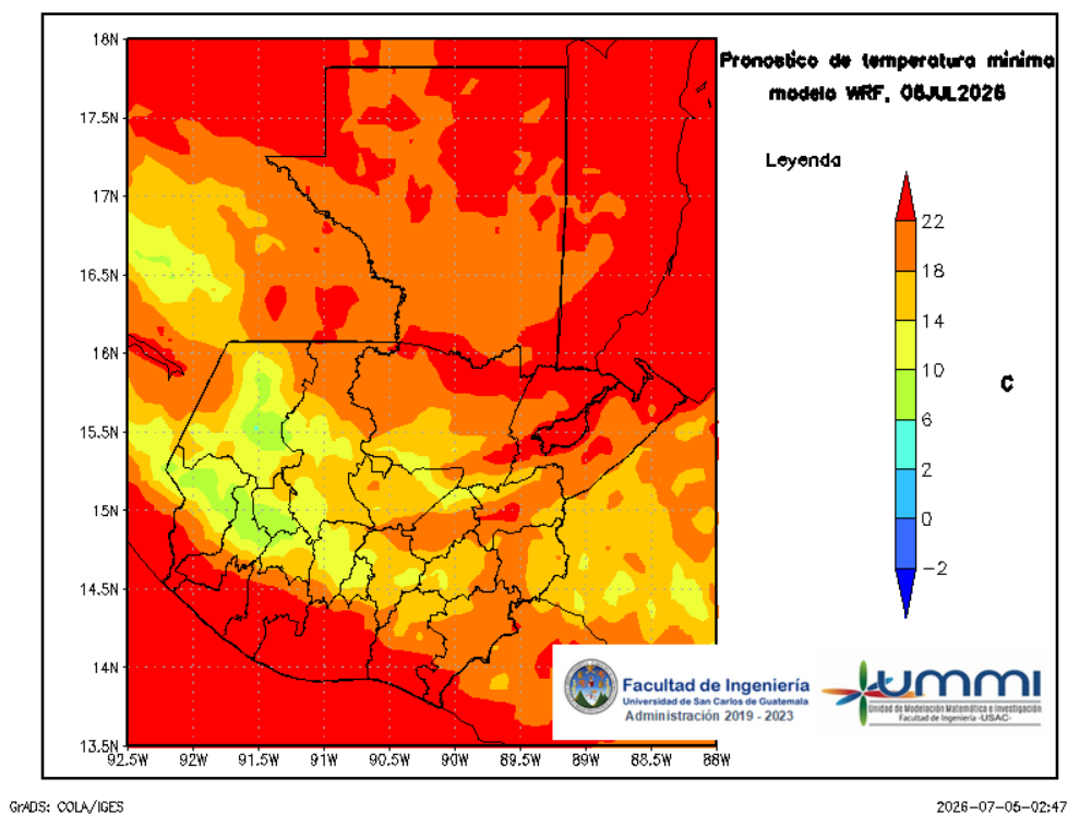
Figura 8: Pronóstico de temperatura mínima diaria del 07 de July
