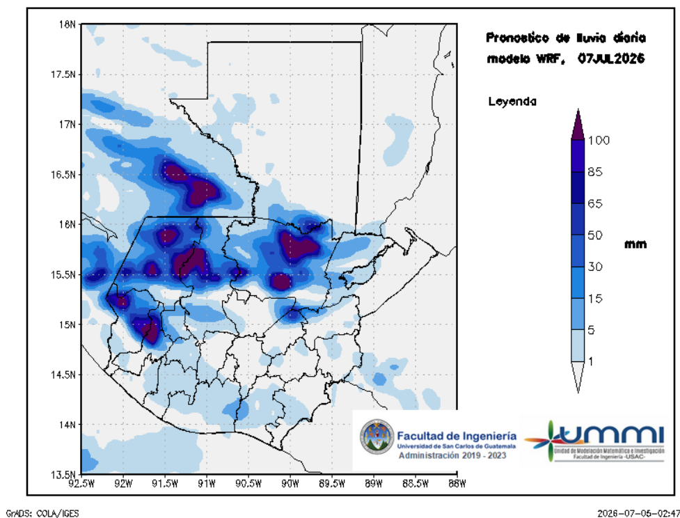
Figura 3: Pronóstico de lluvia diaria del 07 de July
