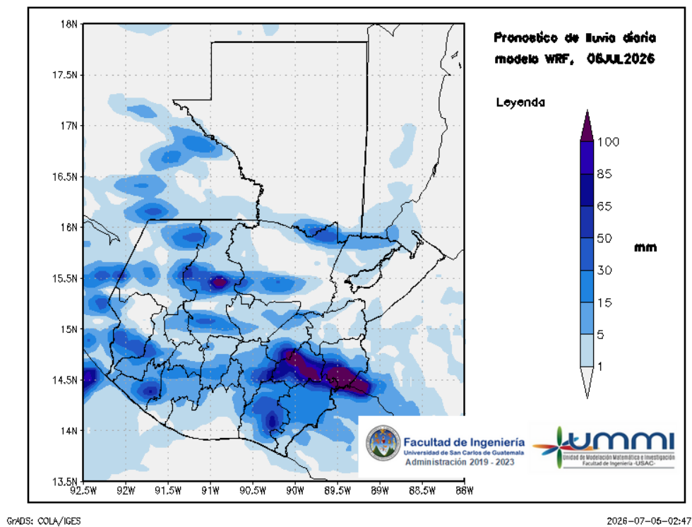
Figura 2: Pronóstico de lluvia diaria del 06 de July
