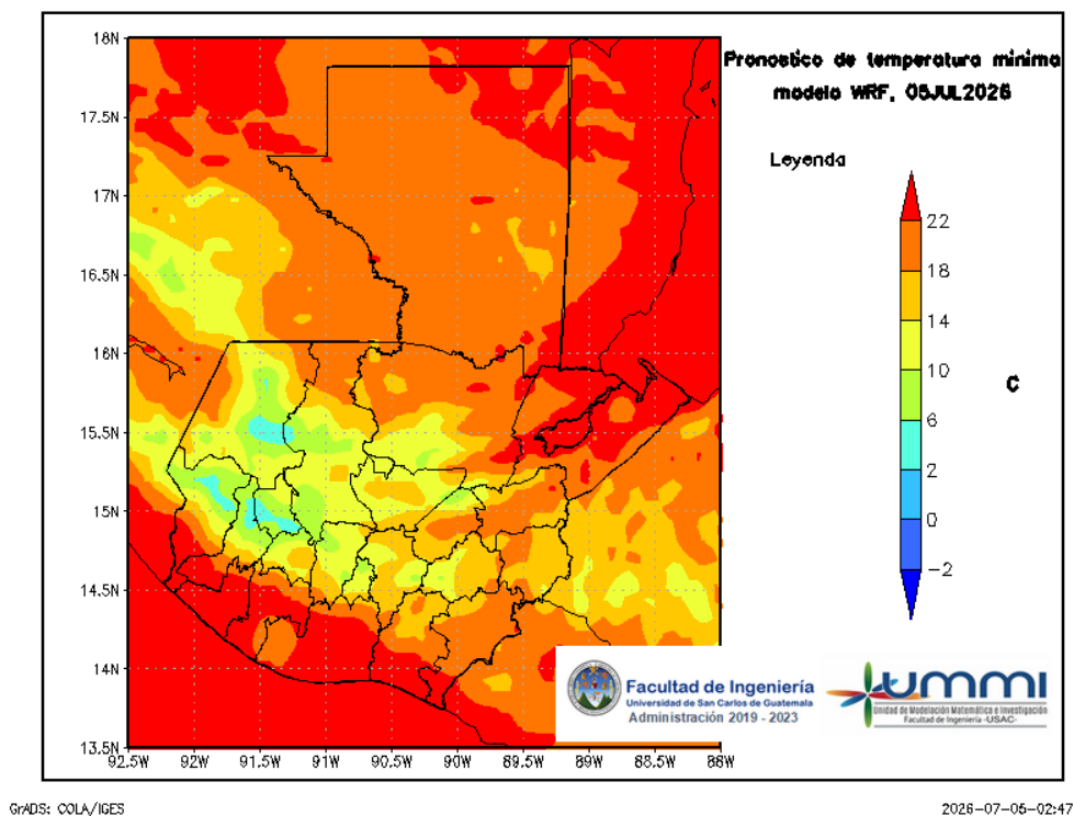
Figura 7: Pronóstico de temperatura mínima diaria del 06 de July
