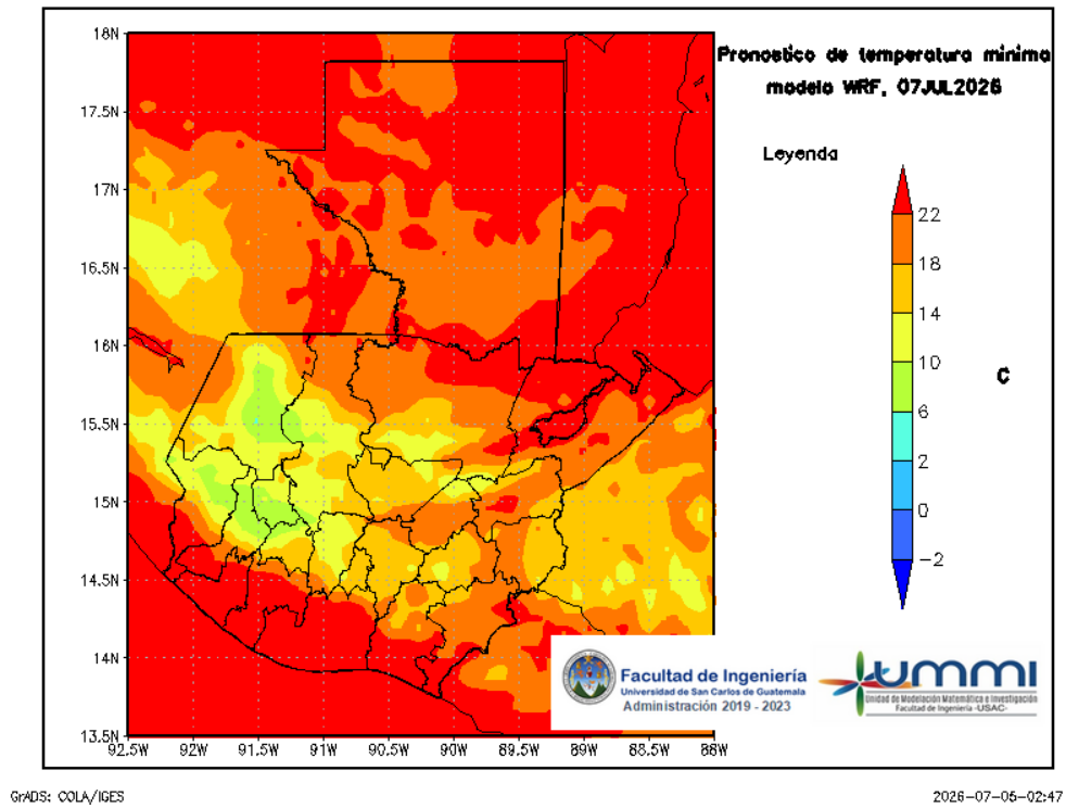
Figura 9: Pronóstico de temperatura mínima diaria del 08 de July
