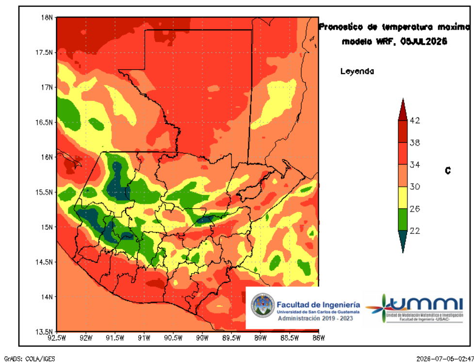
Figura 4: Pronóstico de temperatura máxima diaria del 05 de July
