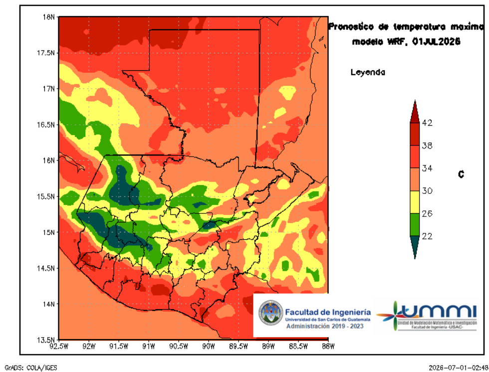
Figura 4: Pronóstico de temperatura máxima diaria del 01 de July
