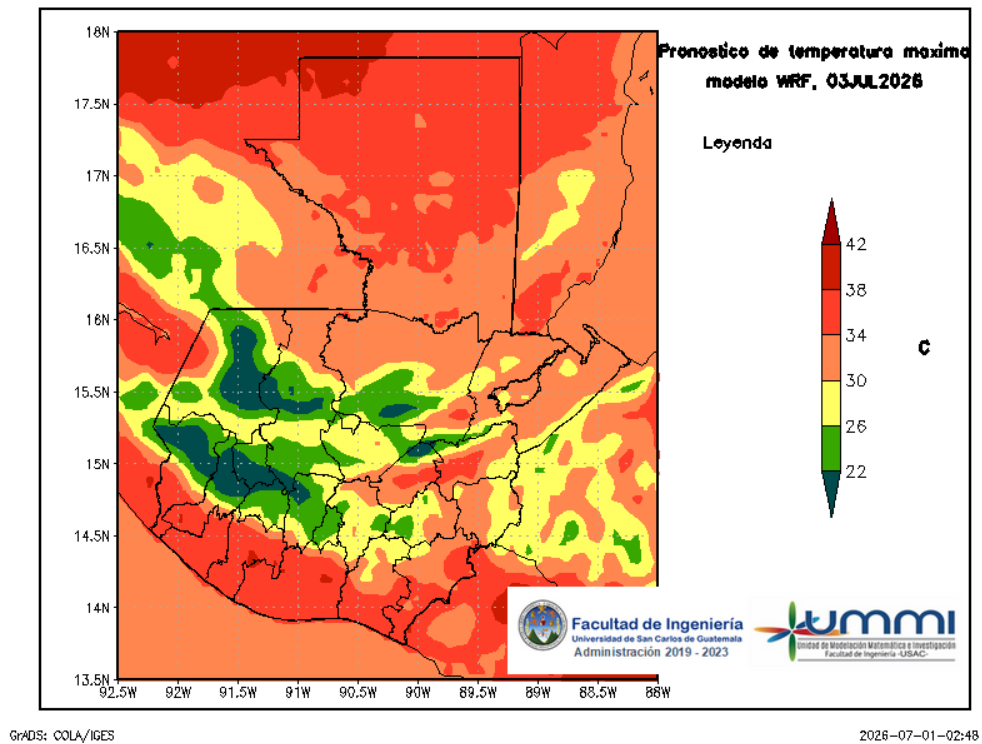
Figura 6: Pronóstico de temperatura máxima diaria del 03 de July
