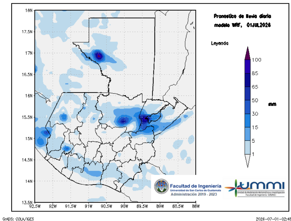
Figura 1: Pronóstico de lluvia diaria del 01 de July
