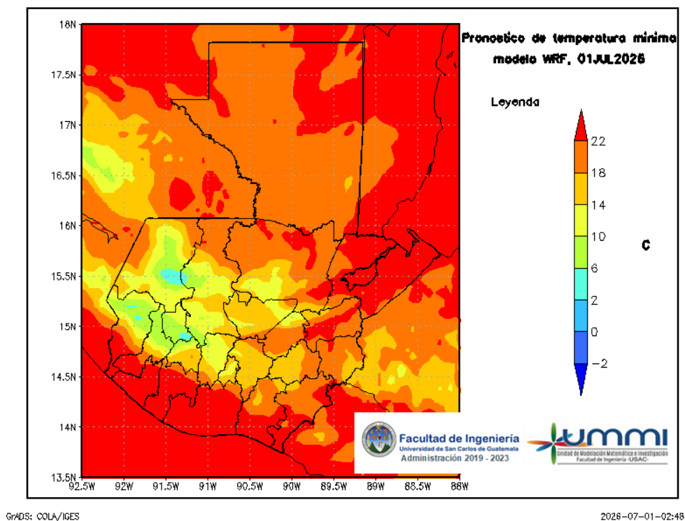
Figura 7: Pronóstico de temperatura mínima diaria del 02 de July
