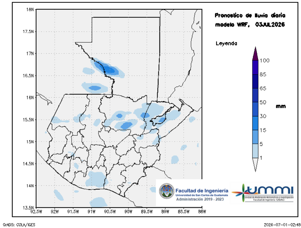
Figura 3: Pronóstico de lluvia diaria del 03 de July
