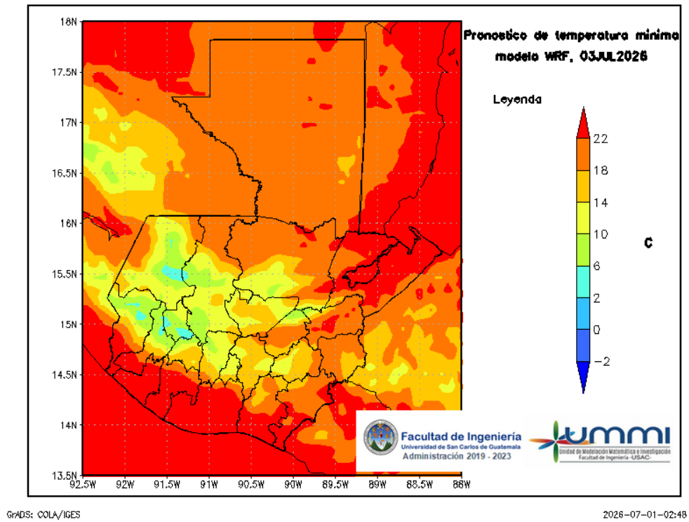
Figura 9: Pronóstico de temperatura mínima diaria del 04 de July
