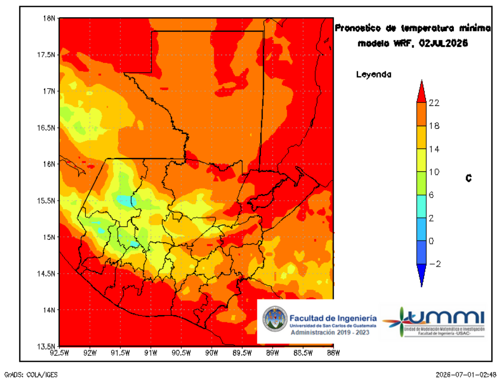
Figura 8: Pronóstico de temperatura mínima diaria del 03 de July
