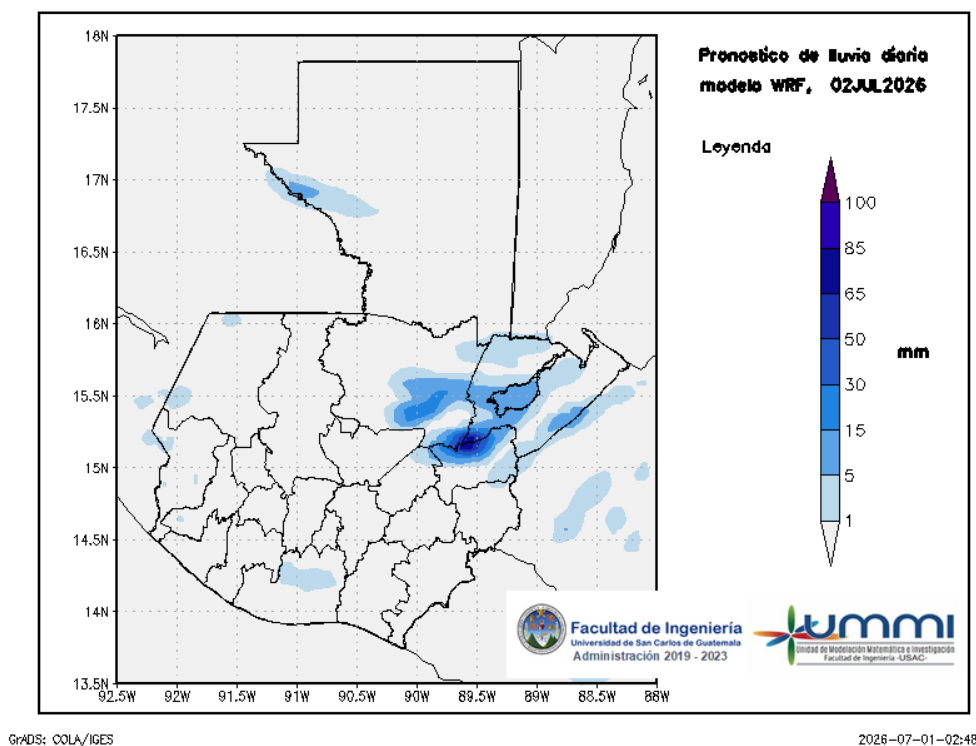
Figura 2: Pronóstico de lluvia diaria del 02 de July
