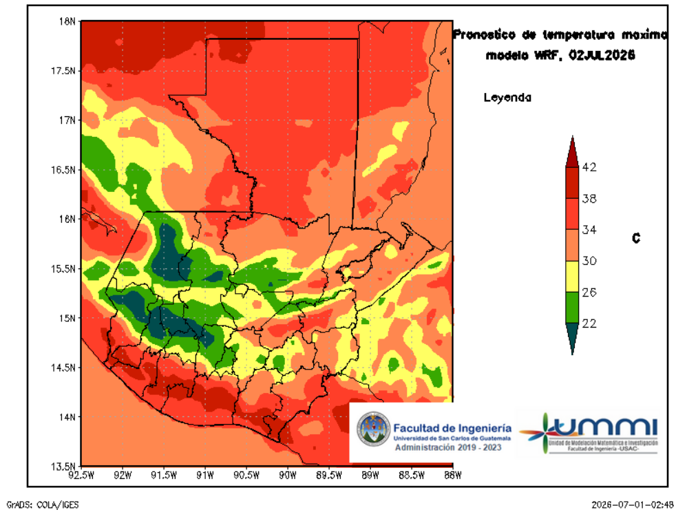
Figura 5: Pronóstico de temperatura máxima diaria del 02 de July
