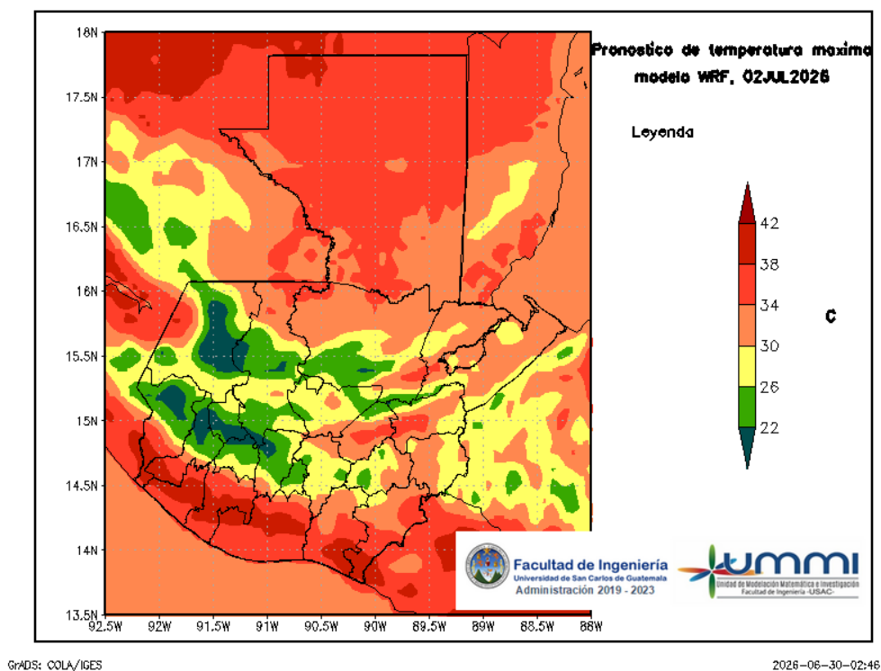
Figura 6: Pronóstico de temperatura máxima diaria del 02 de July
