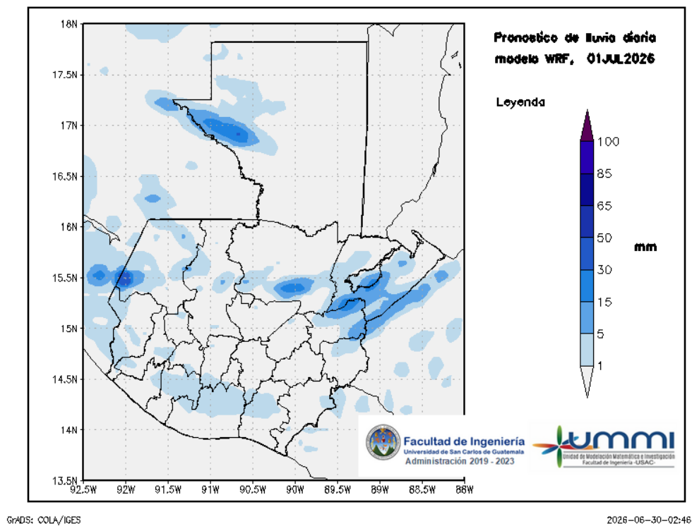
Figura 2: Pronóstico de lluvia diaria del 01 de July
