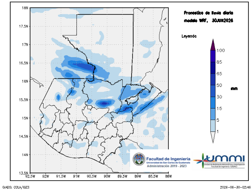
Figura 1: Pronóstico de lluvia diaria del 30 de June
