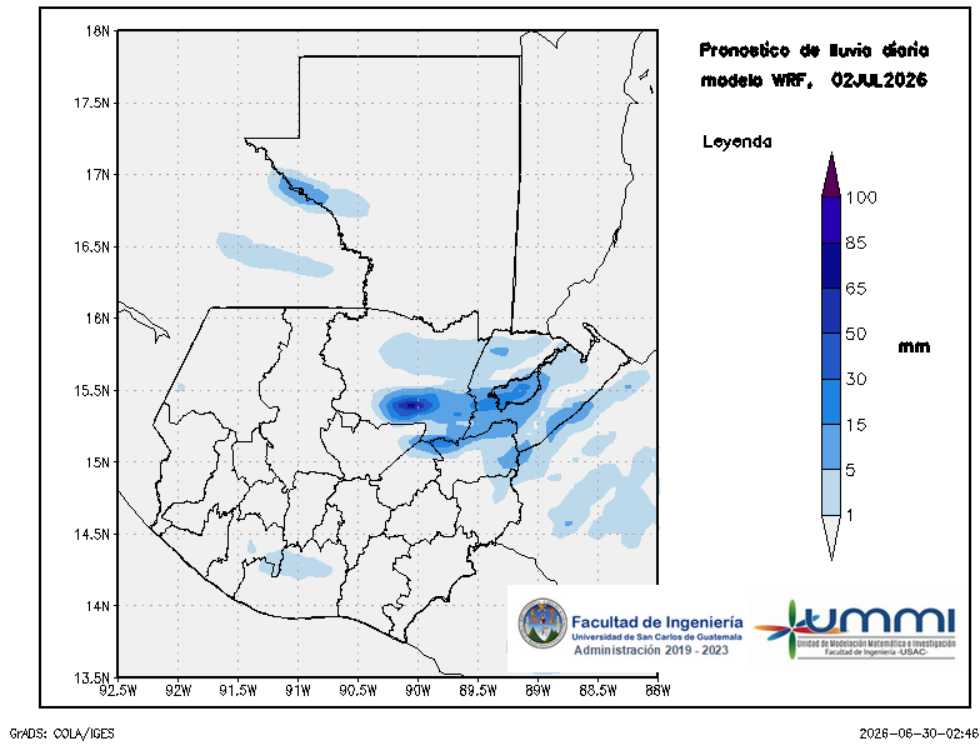
Figura 3: Pronóstico de lluvia diaria del 02 de July
