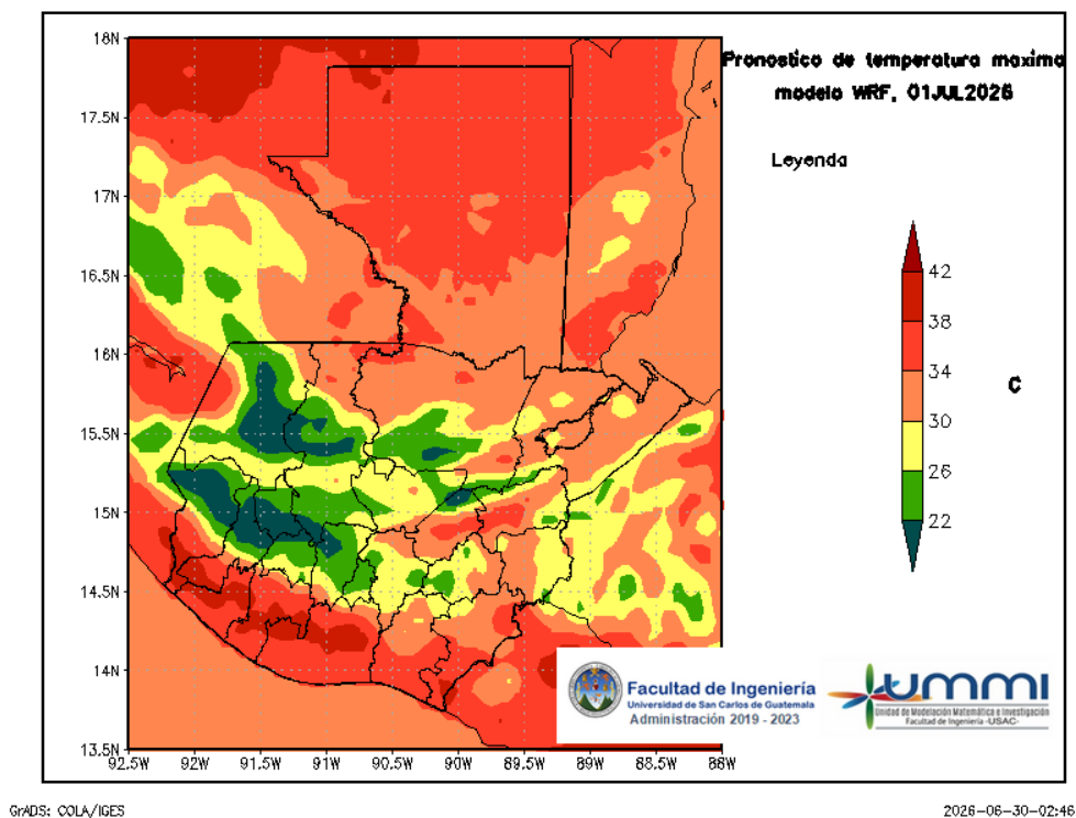
Figura 5: Pronóstico de temperatura máxima diaria del 01 de July
