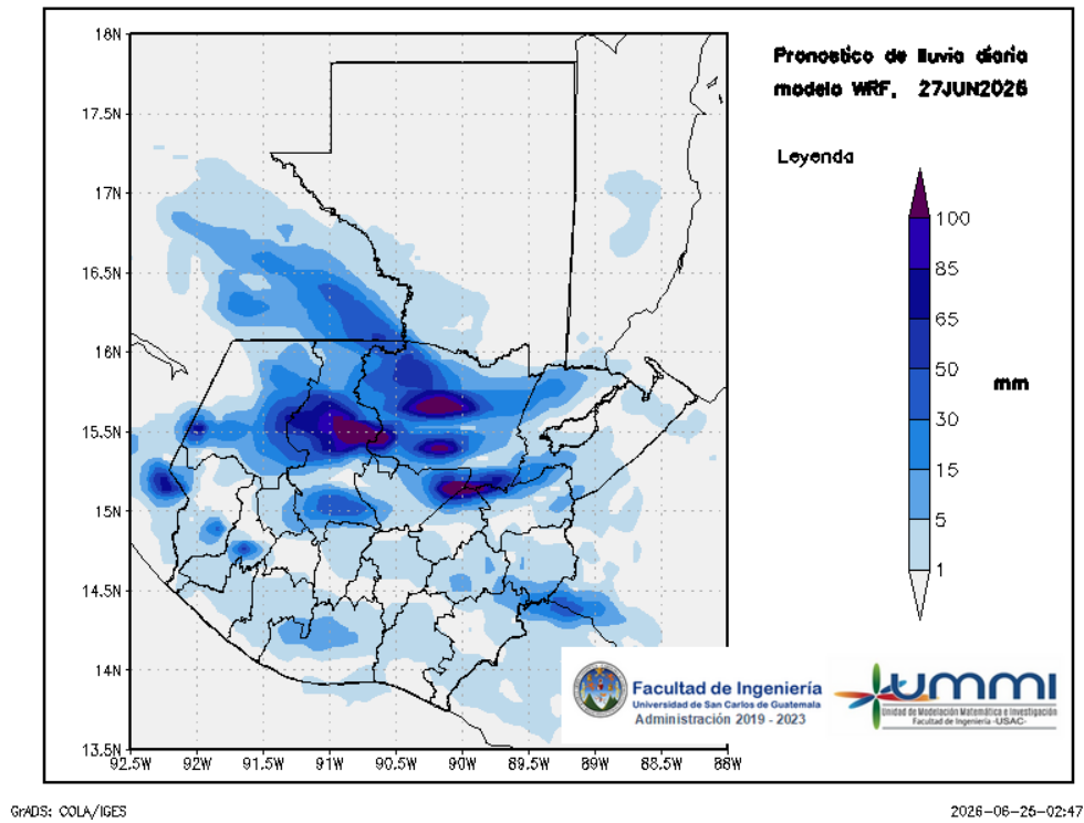
Figura 3: Pronóstico de lluvia diaria del 27 de June
