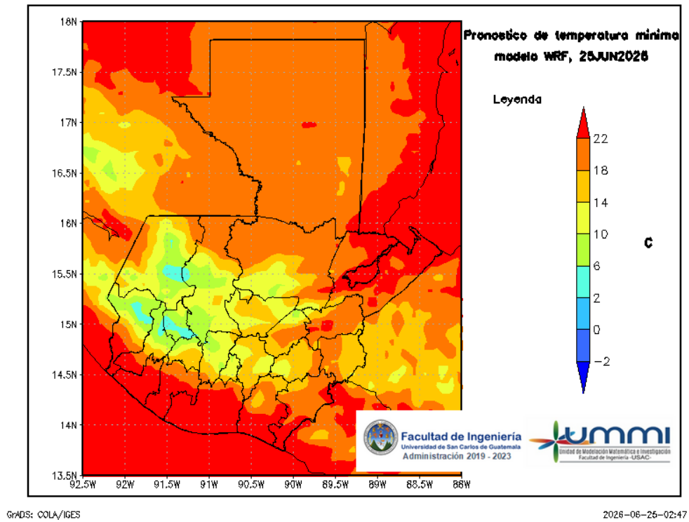
Figura 7: Pronóstico de temperatura mínima diaria del 26 de June
