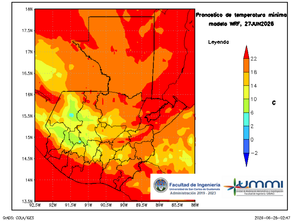
Figura 9: Pronóstico de temperatura mínima diaria del 28 de June
