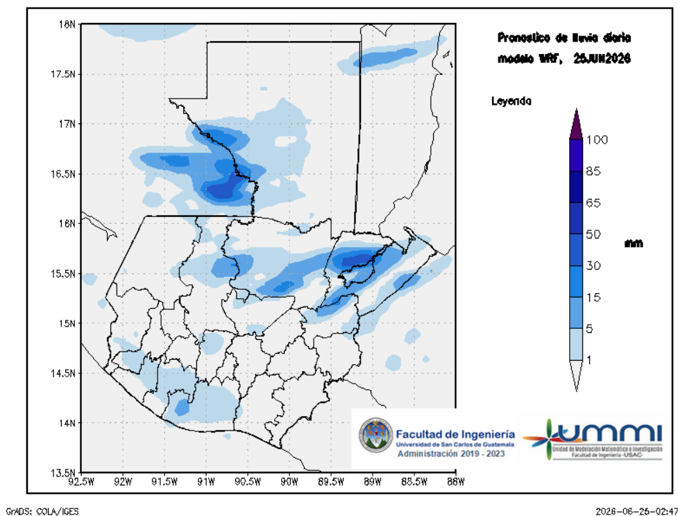
Figura 1: Pronóstico de lluvia diaria del 25 de June
