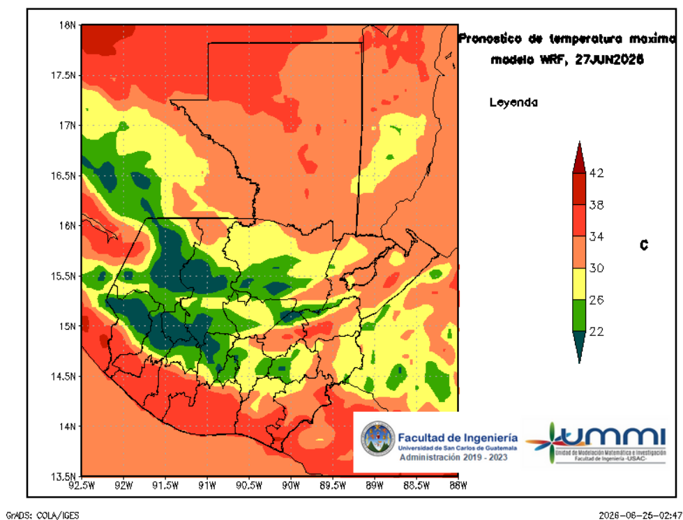
Figura 6: Pronóstico de temperatura máxima diaria del 27 de June
