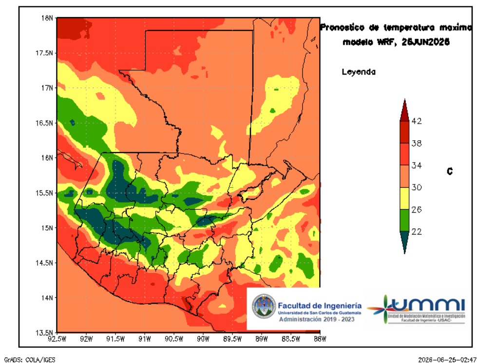
Figura 5: Pronóstico de temperatura máxima diaria del 26 de June
