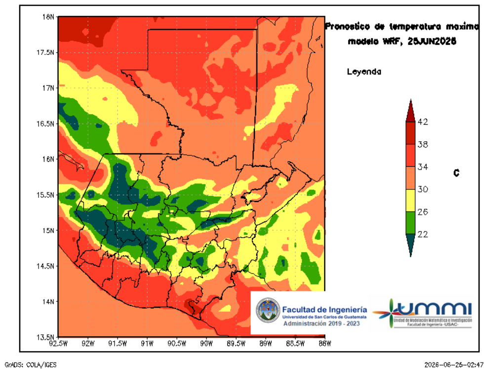
Figura 4: Pronóstico de temperatura máxima diaria del 25 de June
