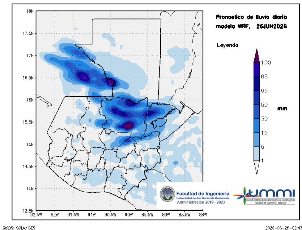
Figura 2: Pronóstico de lluvia diaria del 26 de June
