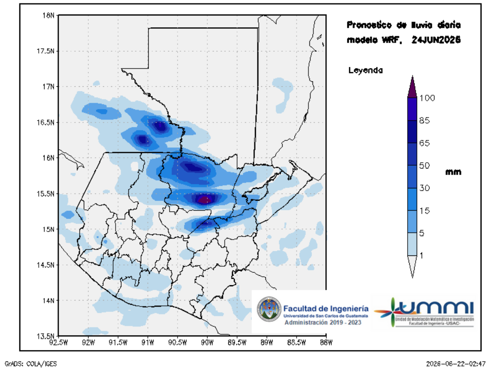
Figura 3: Pronóstico de lluvia diaria del 24 de June
