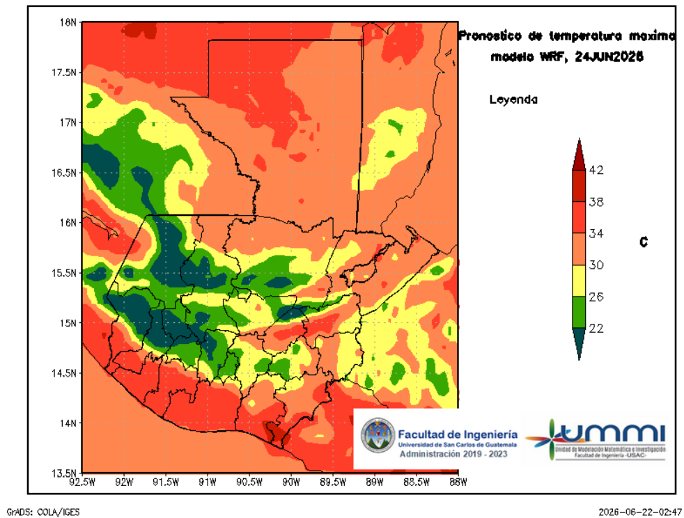
Figura 6: Pronóstico de temperatura máxima diaria del 24 de June
