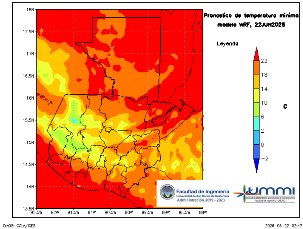
Figura 7: Pronóstico de temperatura mínima diaria del 23 de June
