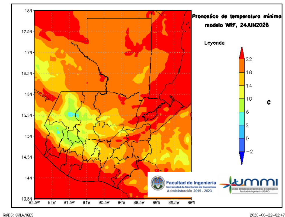
Figura 9: Pronóstico de temperatura mínima diaria del 25 de June
