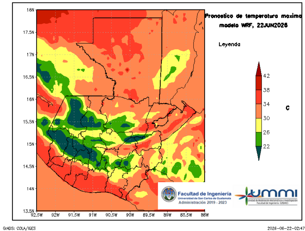
Figura 4: Pronóstico de temperatura máxima diaria del 22 de June
