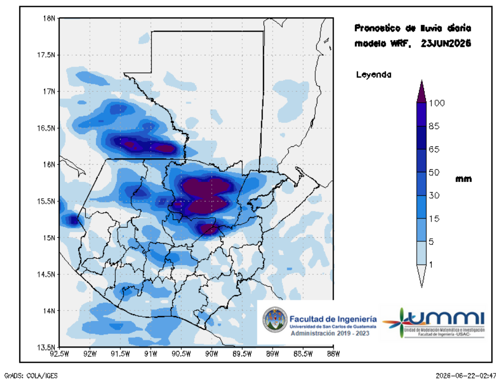
Figura 2: Pronóstico de lluvia diaria del 23 de June
