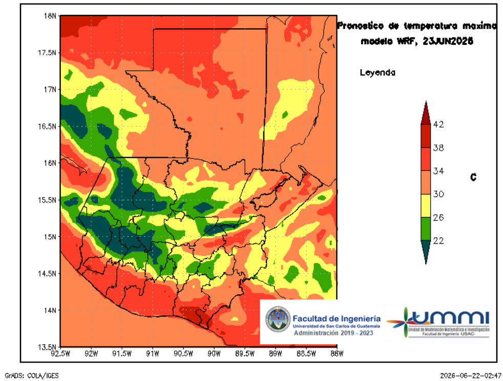
Figura 5: Pronóstico de temperatura máxima diaria del 23 de June
