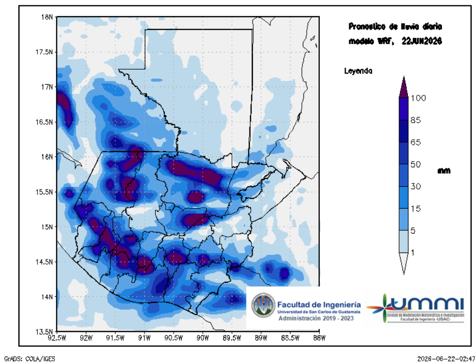
Figura 1: Pronóstico de lluvia diaria del 22 de June
