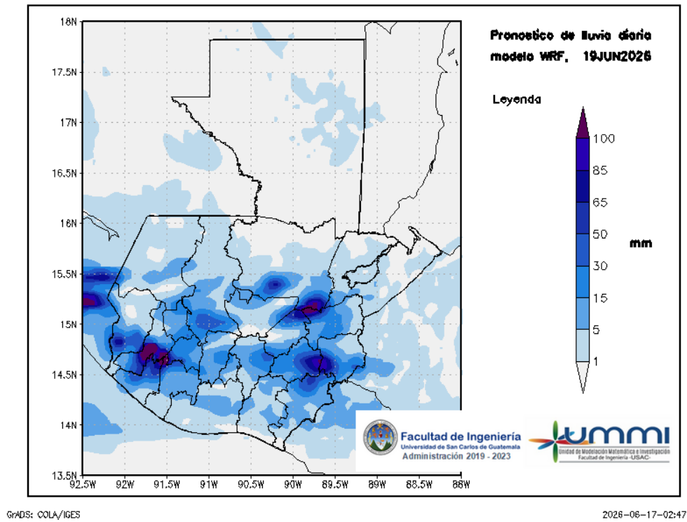
Figura 3: Pronóstico de lluvia diaria del 19 de June
