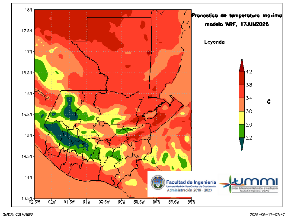
Figura 4: Pronóstico de temperatura máxima diaria del 17 de June
