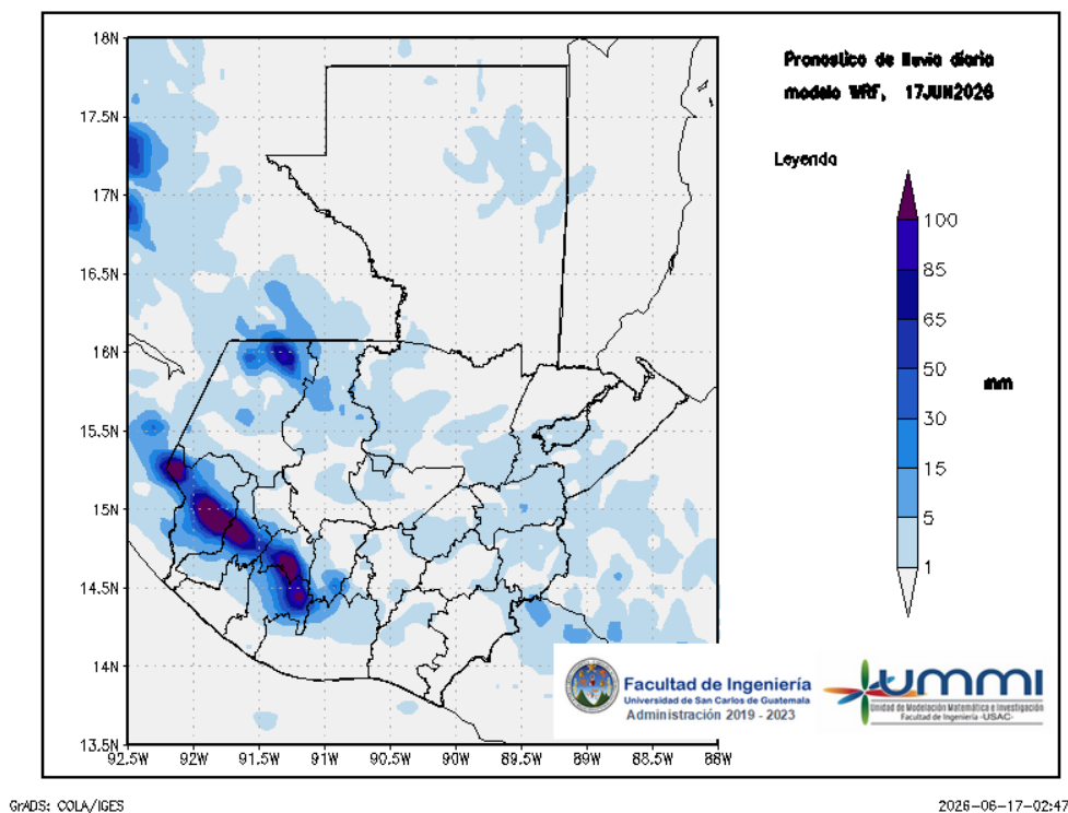
Figura 1: Pronóstico de lluvia diaria del 17 de June
