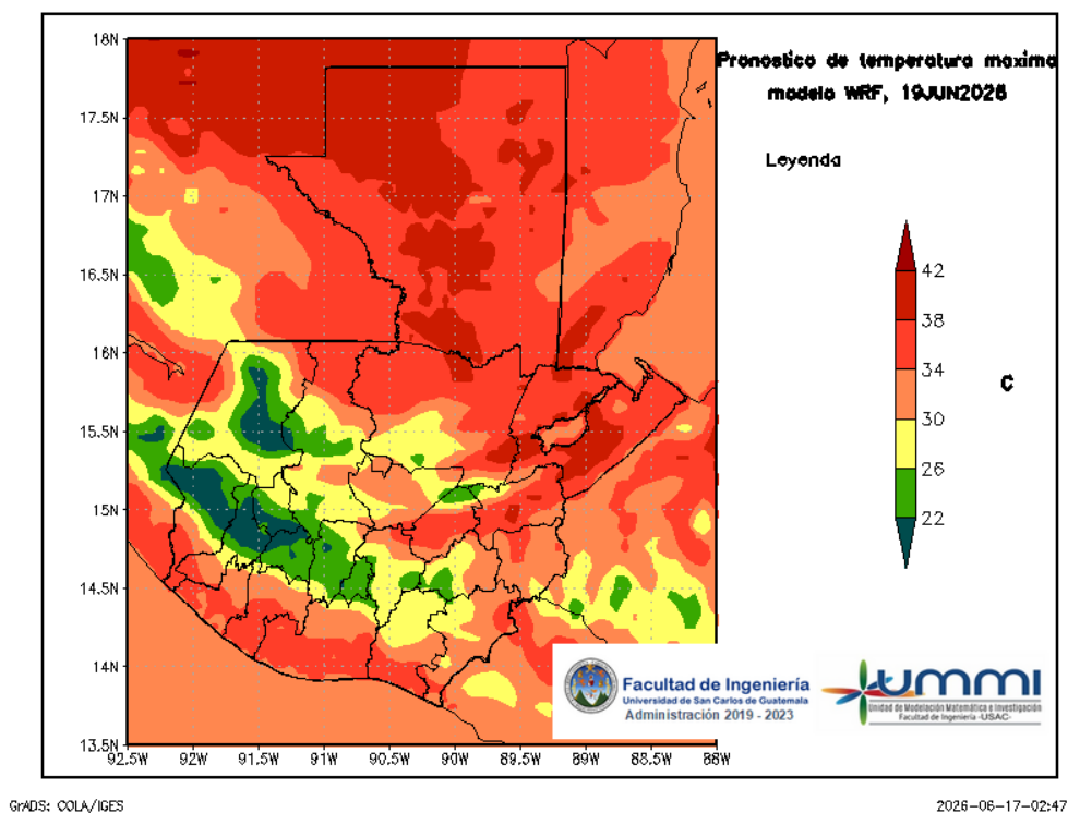
Figura 6: Pronóstico de temperatura máxima diaria del 19 de June
