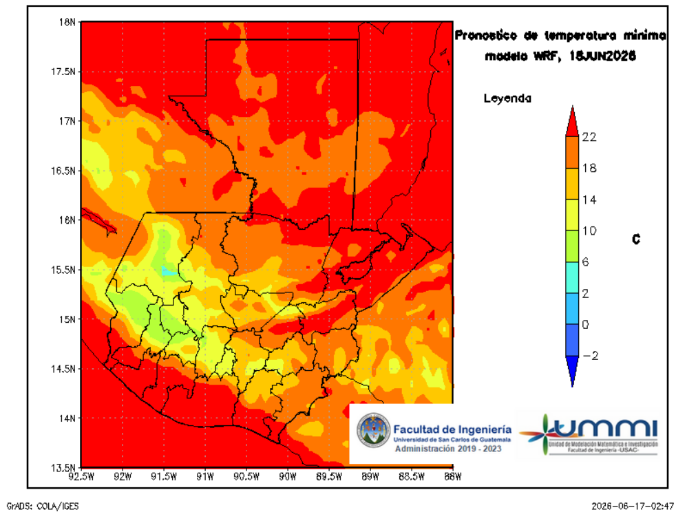
Figura 8: Pronóstico de temperatura mínima diaria del 19 de June
