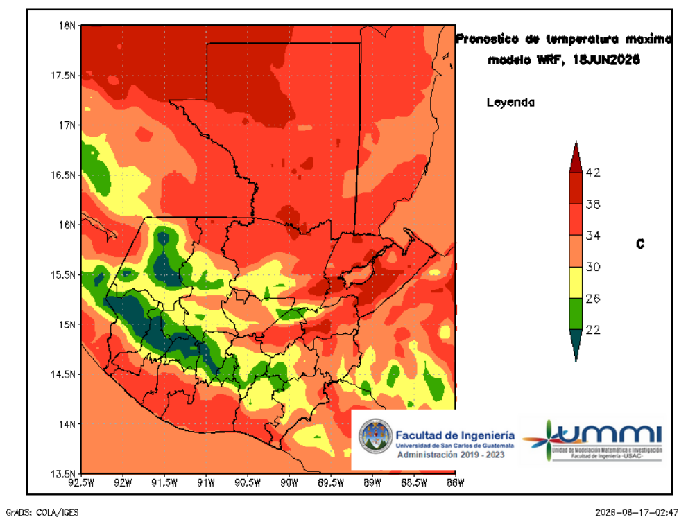
Figura 5: Pronóstico de temperatura máxima diaria del 18 de June
