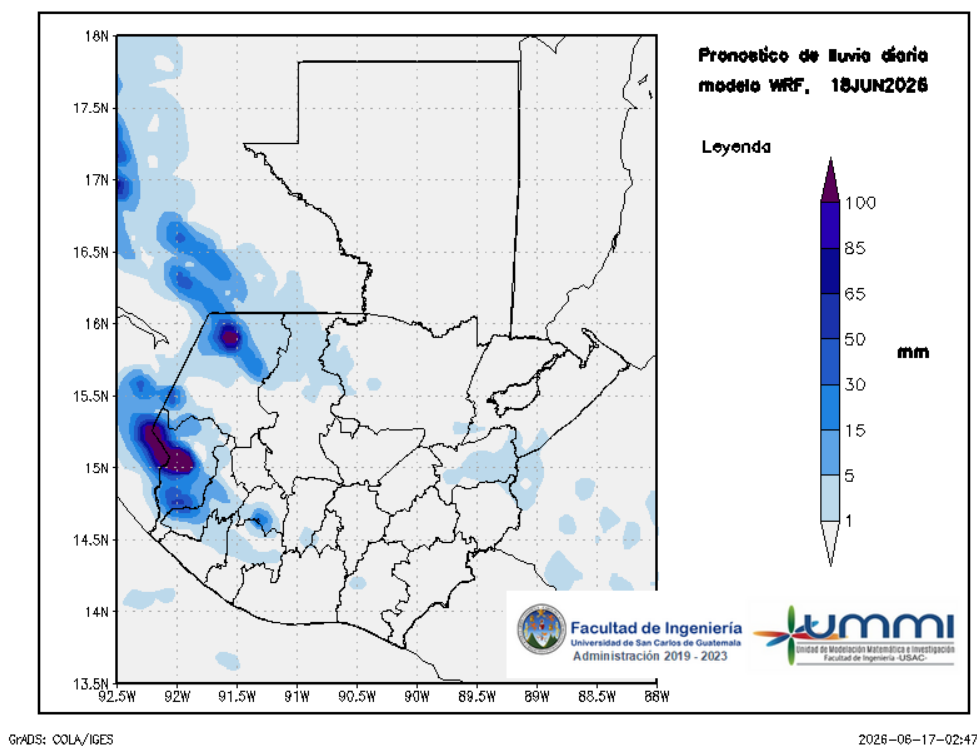
Figura 2: Pronóstico de lluvia diaria del 18 de June
