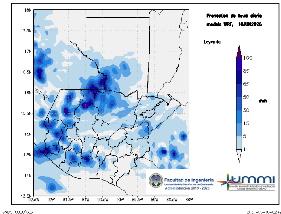
Figura 1: Pronóstico de lluvia diaria del 16 de June
