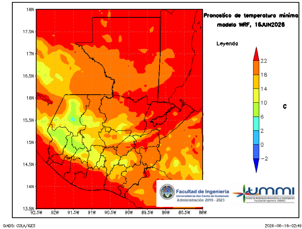
Figura 7: Pronóstico de temperatura mínima diaria del 17 de June
