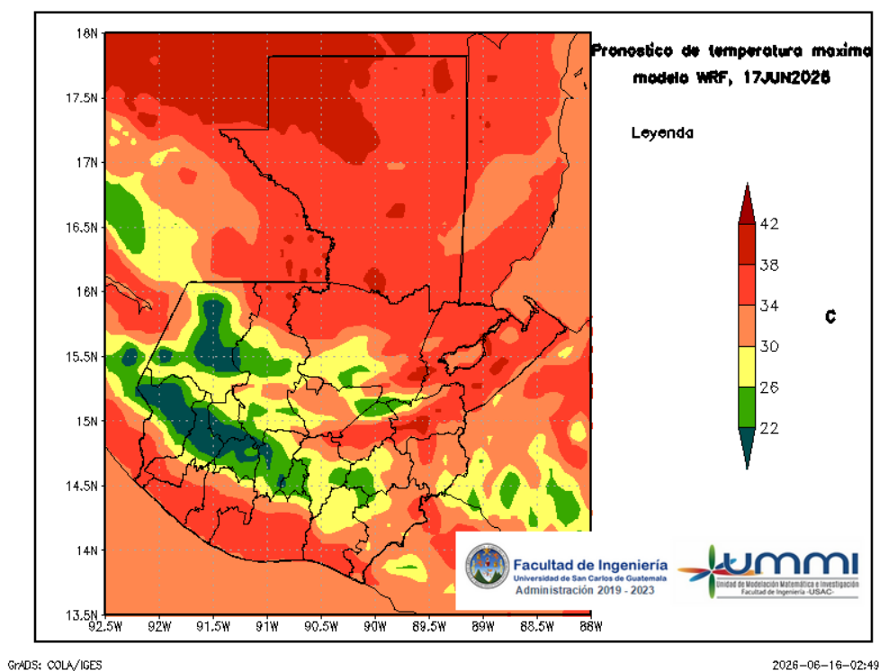
Figura 5: Pronóstico de temperatura máxima diaria del 17 de June
