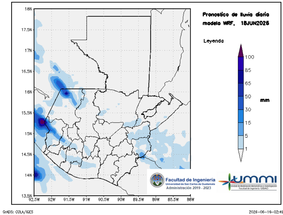
Figura 3: Pronóstico de lluvia diaria del 18 de June
