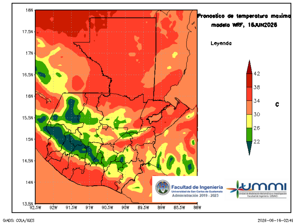
Figura 4: Pronóstico de temperatura máxima diaria del 16 de June
