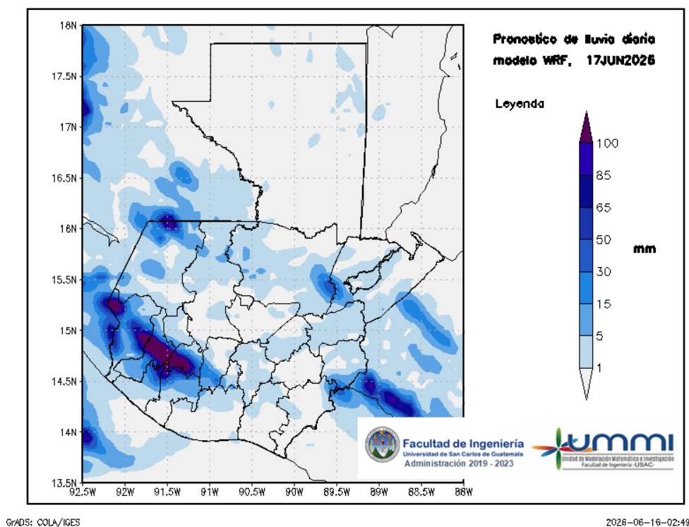
Figura 2: Pronóstico de lluvia diaria del 17 de June
