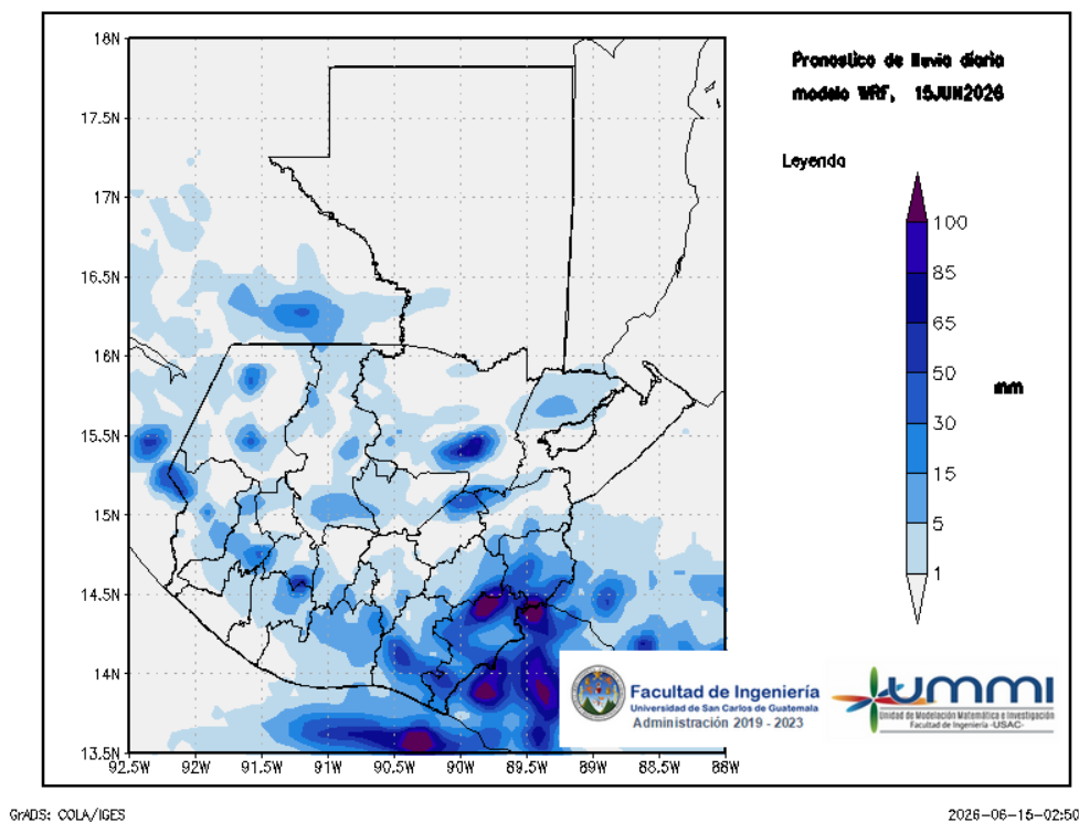
Figura 1: Pronóstico de lluvia diaria del 15 de June
