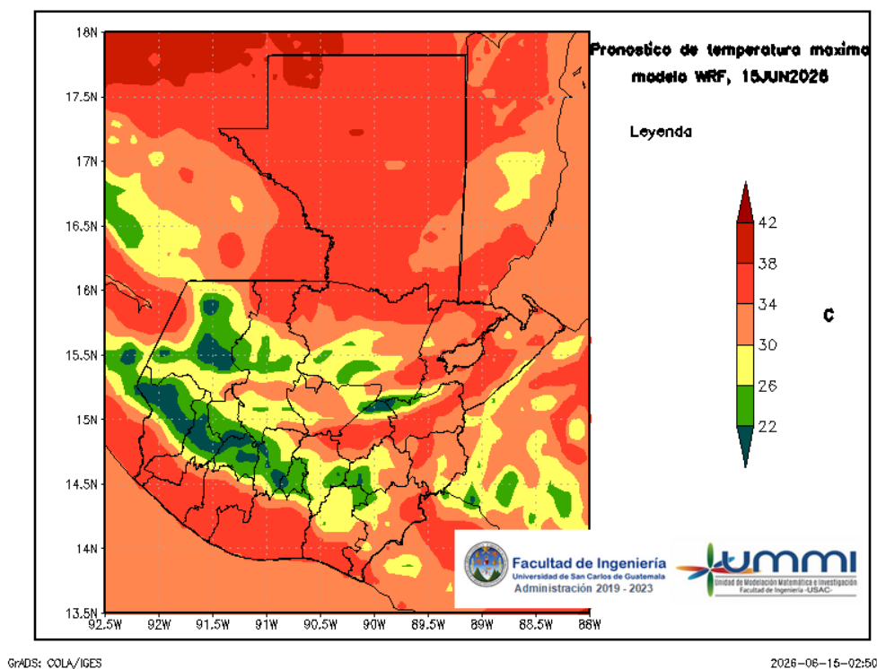
Figura 4: Pronóstico de temperatura máxima diaria del 15 de June
