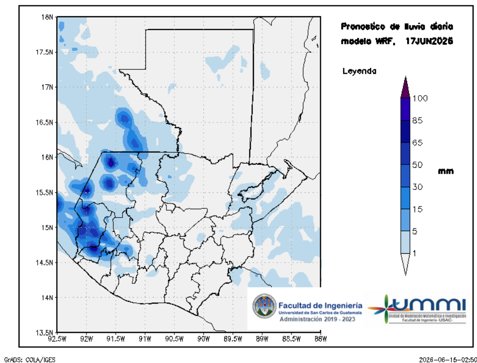
Figura 3: Pronóstico de lluvia diaria del 17 de June
