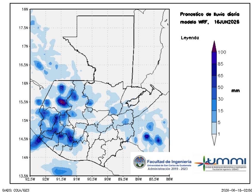
Figura 2: Pronóstico de lluvia diaria del 16 de June
