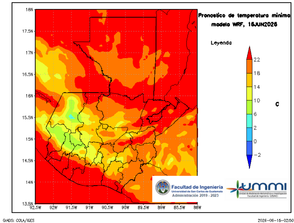
Figura 8: Pronóstico de temperatura mínima diaria del 17 de June
