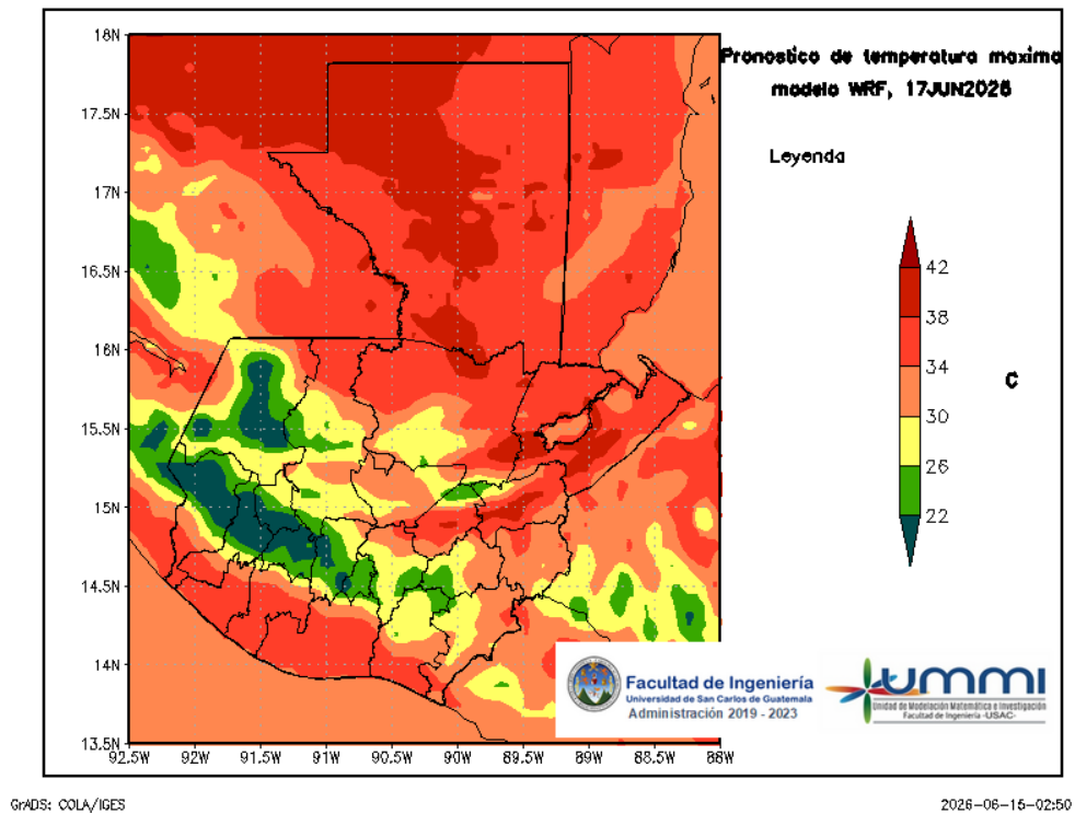
Figura 6: Pronóstico de temperatura máxima diaria del 17 de June
