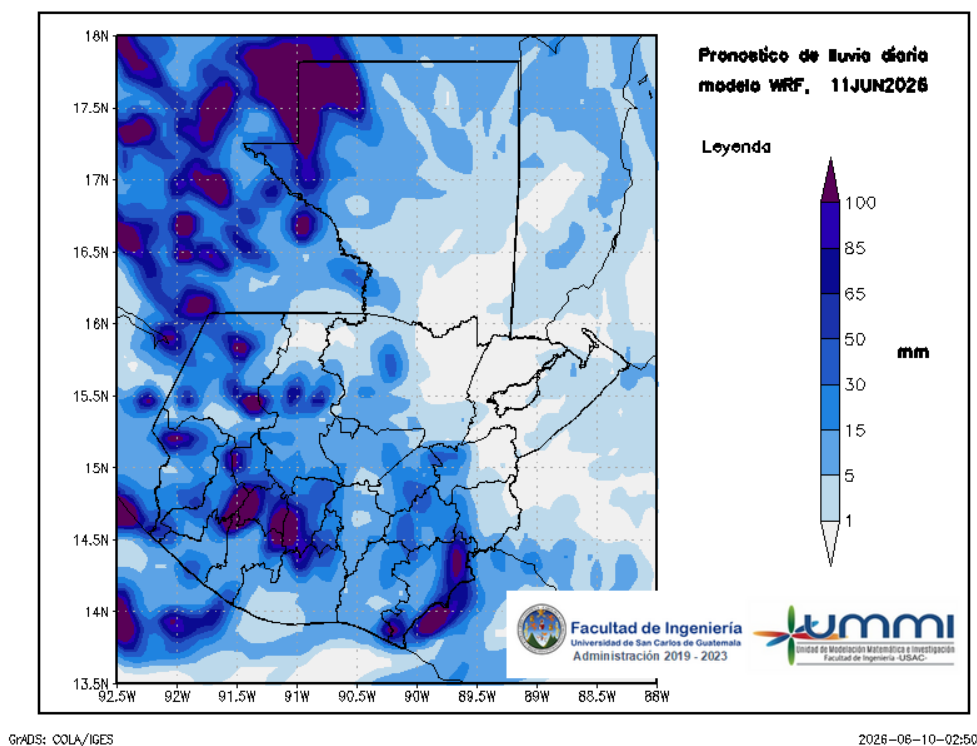
Figura 2: Pronóstico de lluvia diaria del 11 de June
