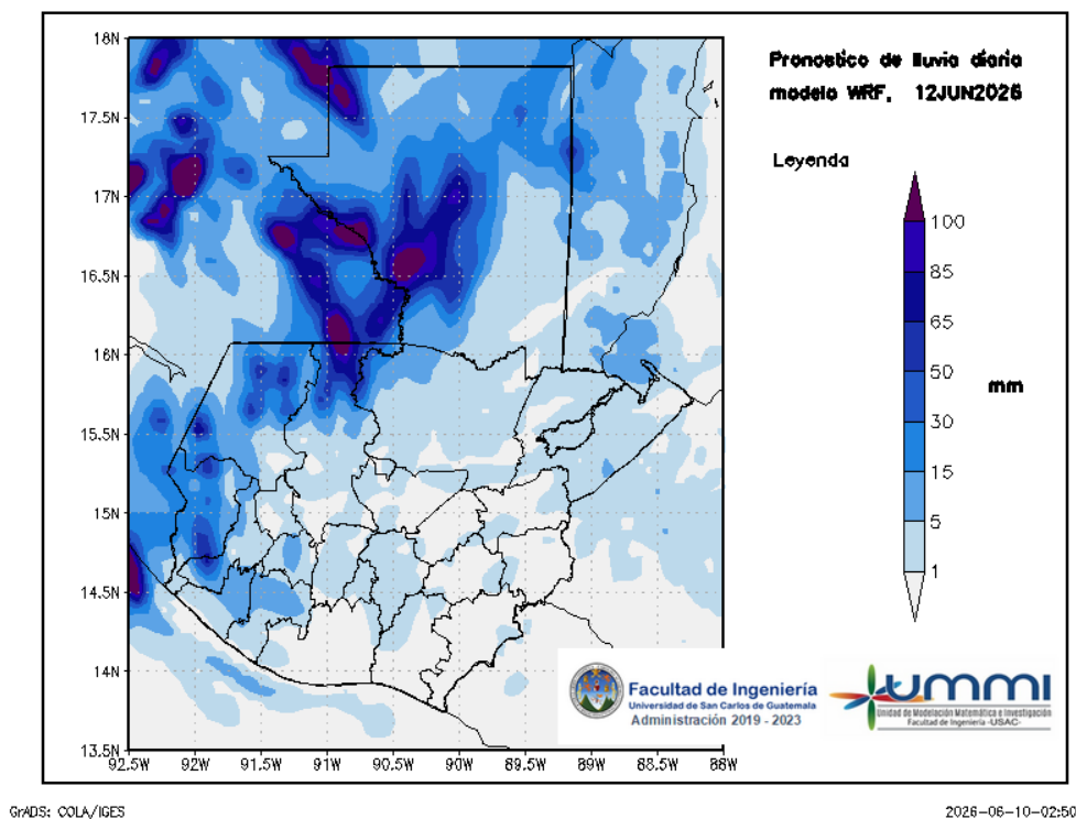
Figura 3: Pronóstico de lluvia diaria del 12 de June
