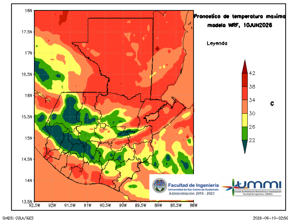
Figura 4: Pronóstico de temperatura máxima diaria del 10 de June
