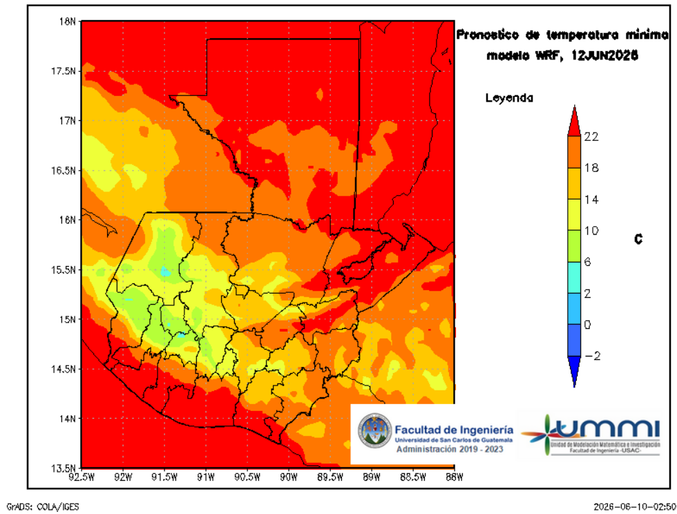
Figura 9: Pronóstico de temperatura mínima diaria del 13 de June
