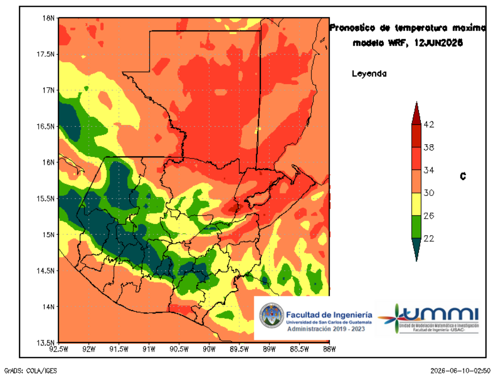
Figura 6: Pronóstico de temperatura máxima diaria del 12 de June
