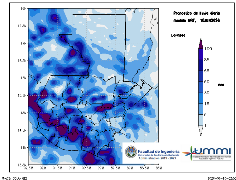
Figura 1: Pronóstico de lluvia diaria del 10 de June
