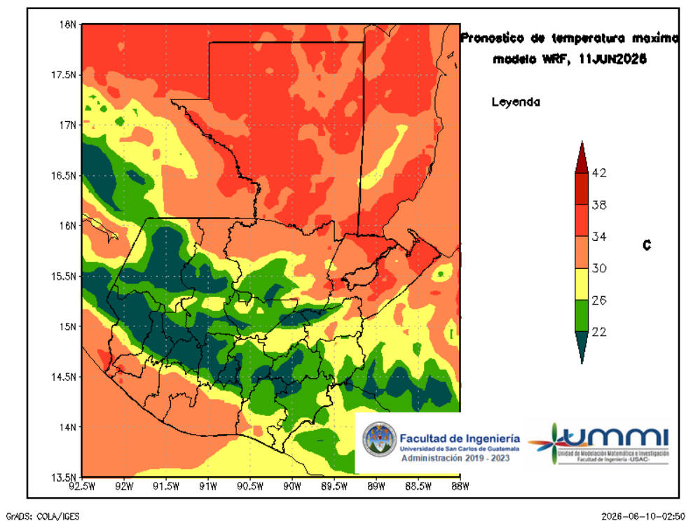
Figura 5: Pronóstico de temperatura máxima diaria del 11 de June
