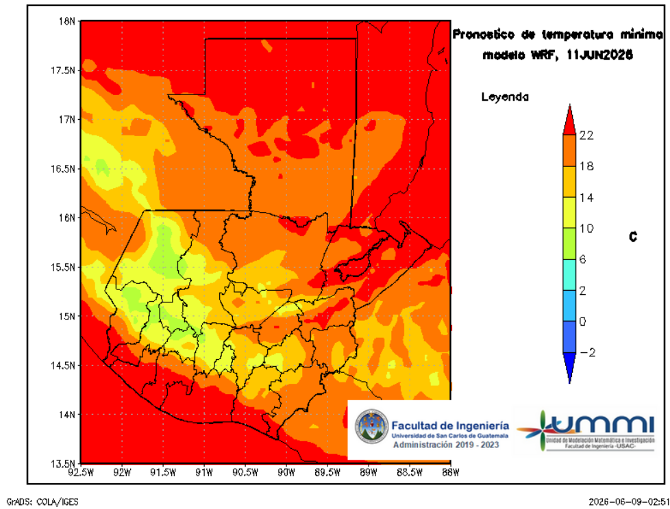
Figura 9: Pronóstico de temperatura mínima diaria del 12 de June
