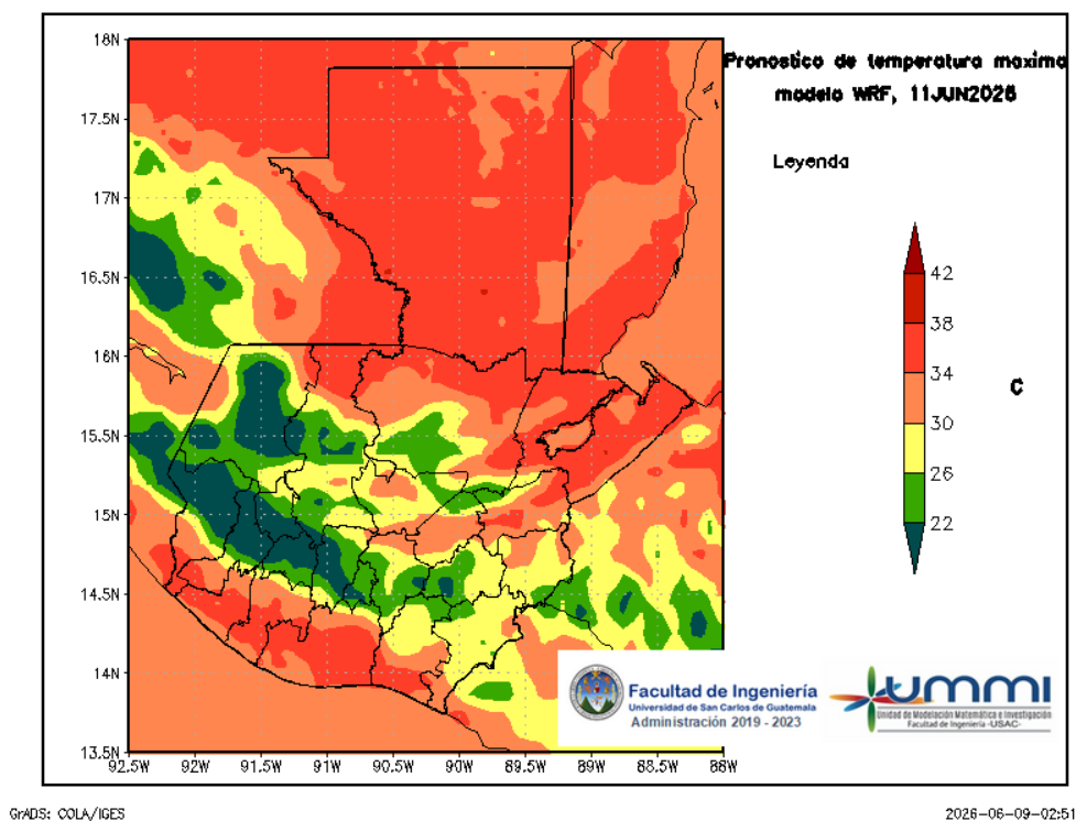
Figura 6: Pronóstico de temperatura máxima diaria del 11 de June
