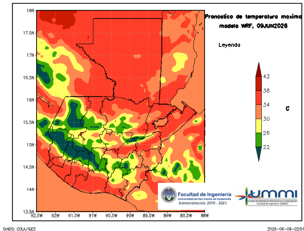
Figura 4: Pronóstico de temperatura máxima diaria del 09 de June
