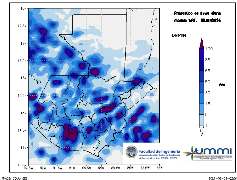
Figura 1: Pronóstico de lluvia diaria del 09 de June
