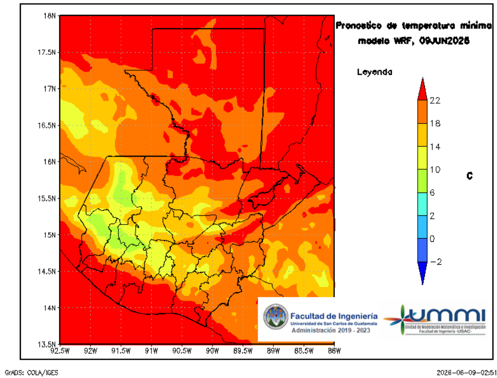
Figura 7: Pronóstico de temperatura mínima diaria del 10 de June
