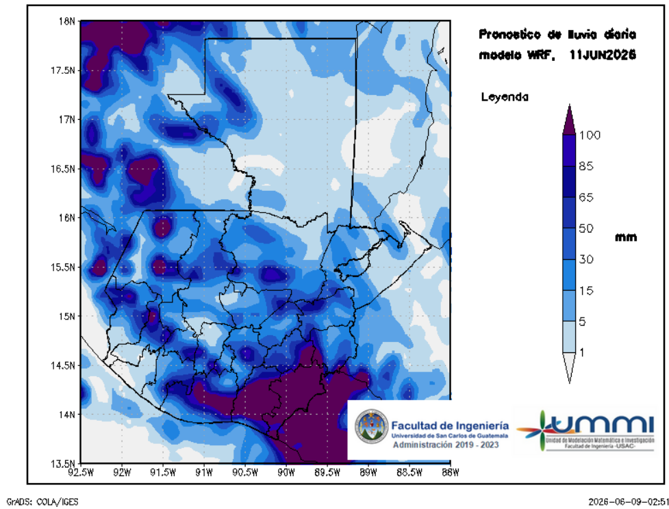
Figura 3: Pronóstico de lluvia diaria del 11 de June
