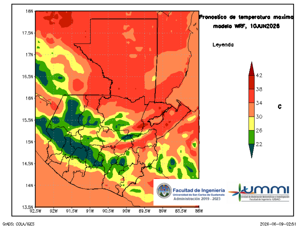
Figura 5: Pronóstico de temperatura máxima diaria del 10 de June
