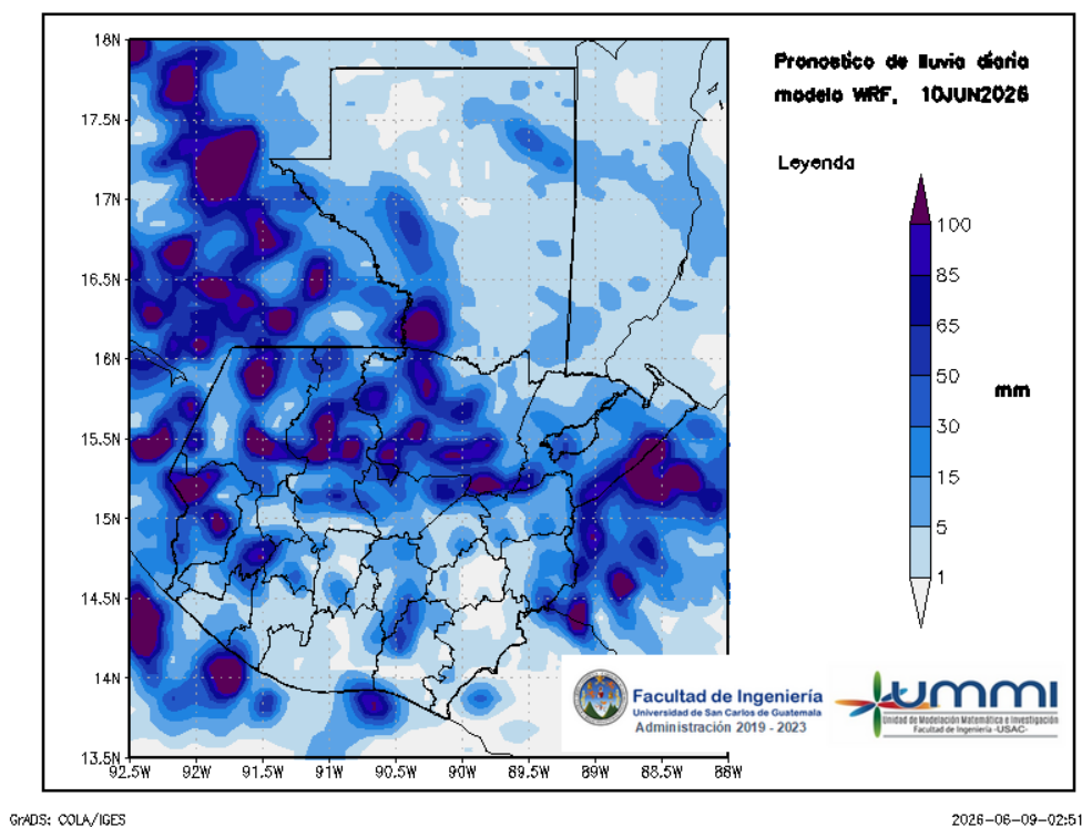
Figura 2: Pronóstico de lluvia diaria del 10 de June
