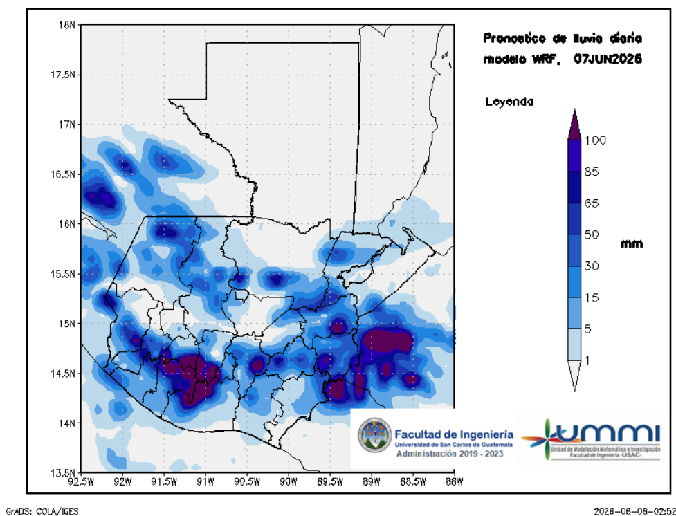
Figura 2: Pronóstico de lluvia diaria del 07 de June
