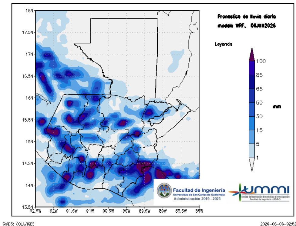
Figura 1: Pronóstico de lluvia diaria del 06 de June
