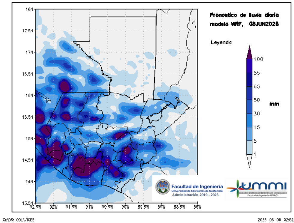
Figura 3: Pronóstico de lluvia diaria del 08 de June
