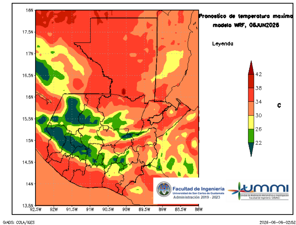
Figura 4: Pronóstico de temperatura máxima diaria del 06 de June
