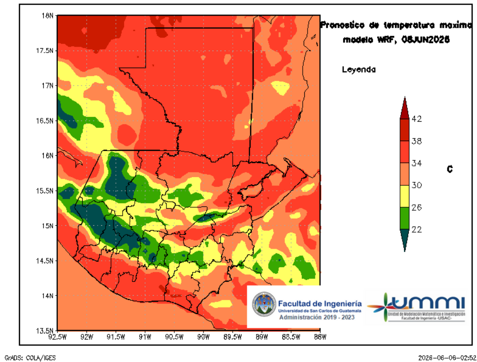
Figura 6: Pronóstico de temperatura máxima diaria del 08 de June
