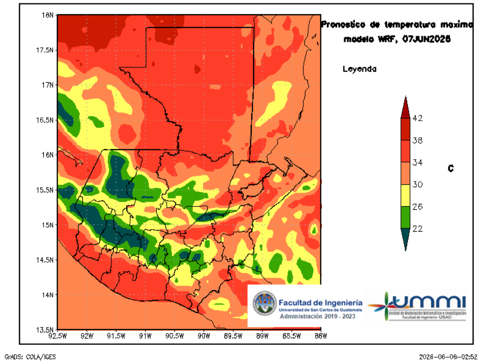
Figura 5: Pronóstico de temperatura máxima diaria del 07 de June
