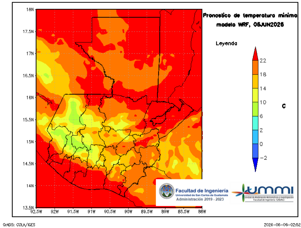
Figura 7: Pronóstico de temperatura mínima diaria del 07 de June
