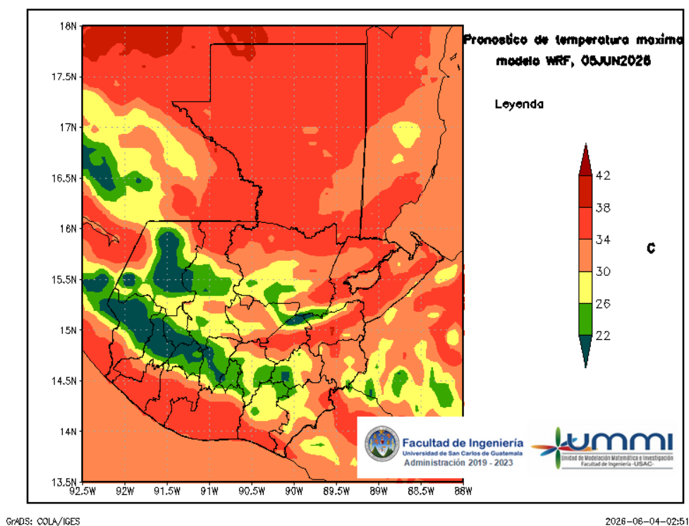
Figura 5: Pronóstico de temperatura máxima diaria del 05 de June
