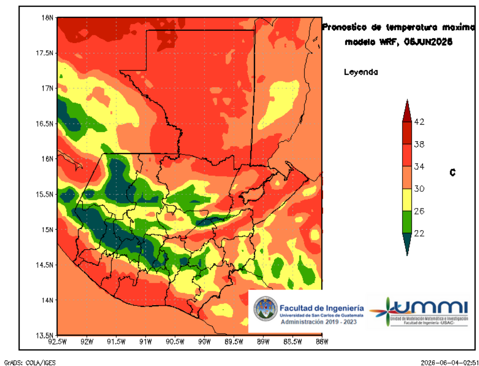
Figura 6: Pronóstico de temperatura máxima diaria del 06 de June
