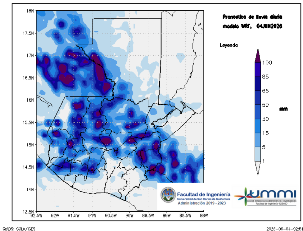
Figura 1: Pronóstico de lluvia diaria del 04 de June
