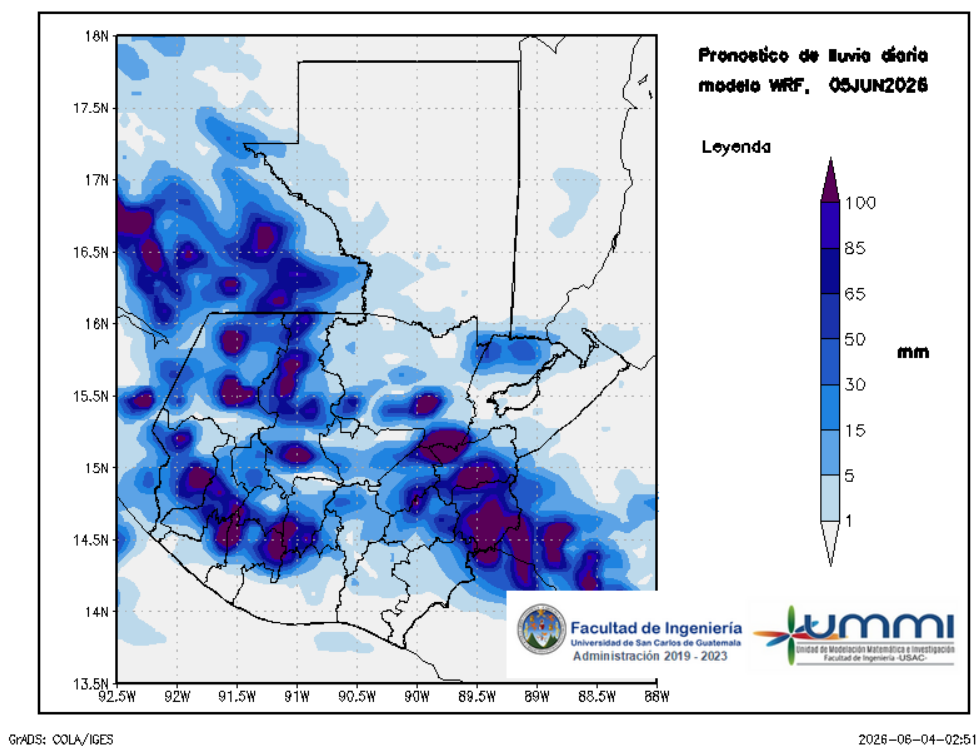
Figura 2: Pronóstico de lluvia diaria del 05 de June
