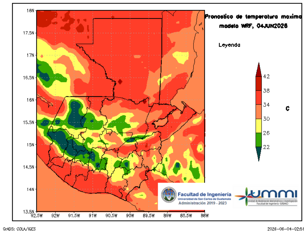
Figura 4: Pronóstico de temperatura máxima diaria del 04 de June
