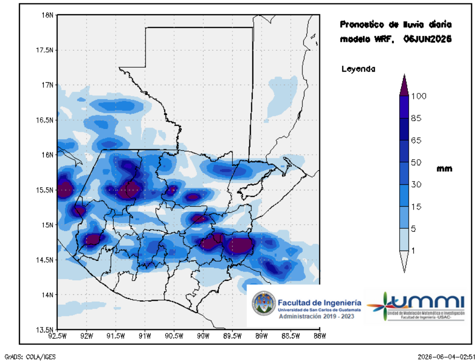
Figura 3: Pronóstico de lluvia diaria del 06 de June
