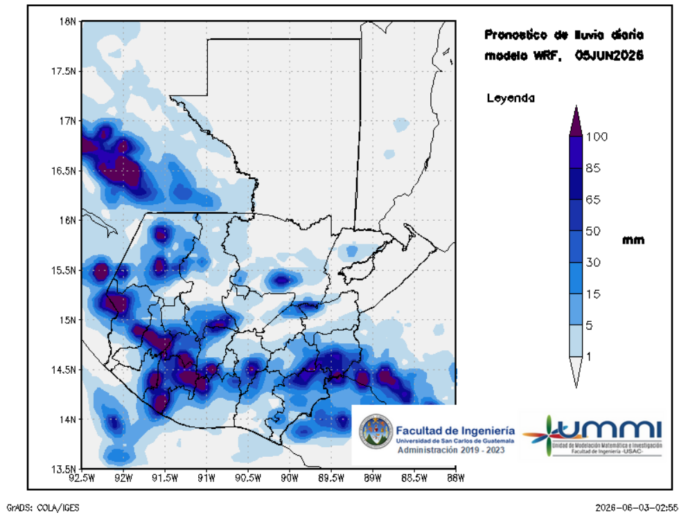
Figura 3: Pronóstico de lluvia diaria del 05 de June
