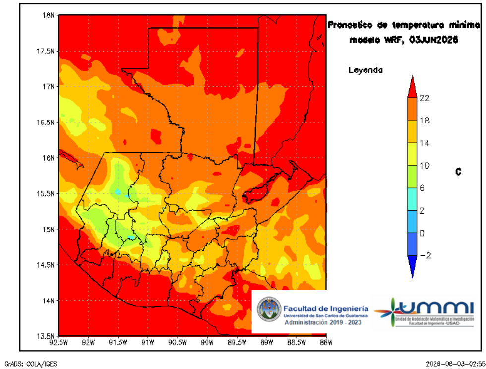
Figura 7: Pronóstico de temperatura mínima diaria del 04 de June
