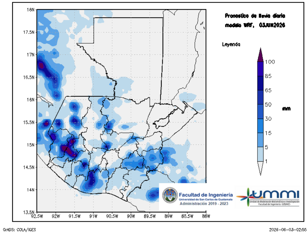
Figura 1: Pronóstico de lluvia diaria del 03 de June
