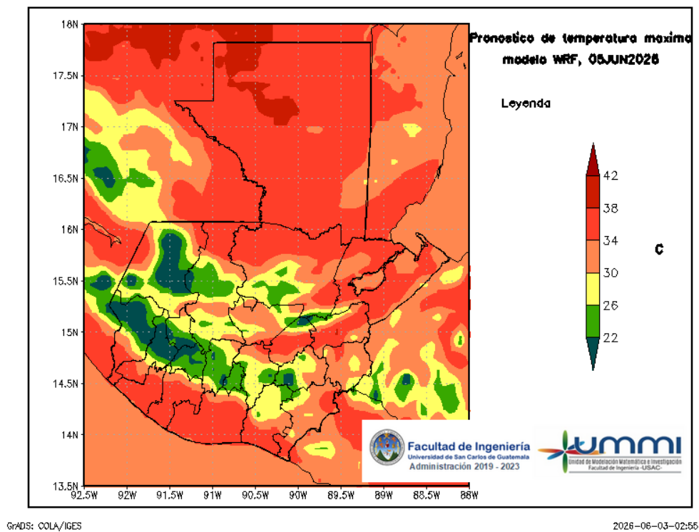
Figura 6: Pronóstico de temperatura máxima diaria del 05 de June
