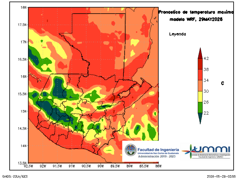
Figura 5: Pronóstico de temperatura máxima diaria del 29 de May
