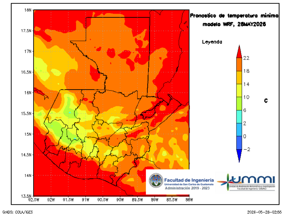
Figura 7: Pronóstico de temperatura mínima diaria del 29 de May
