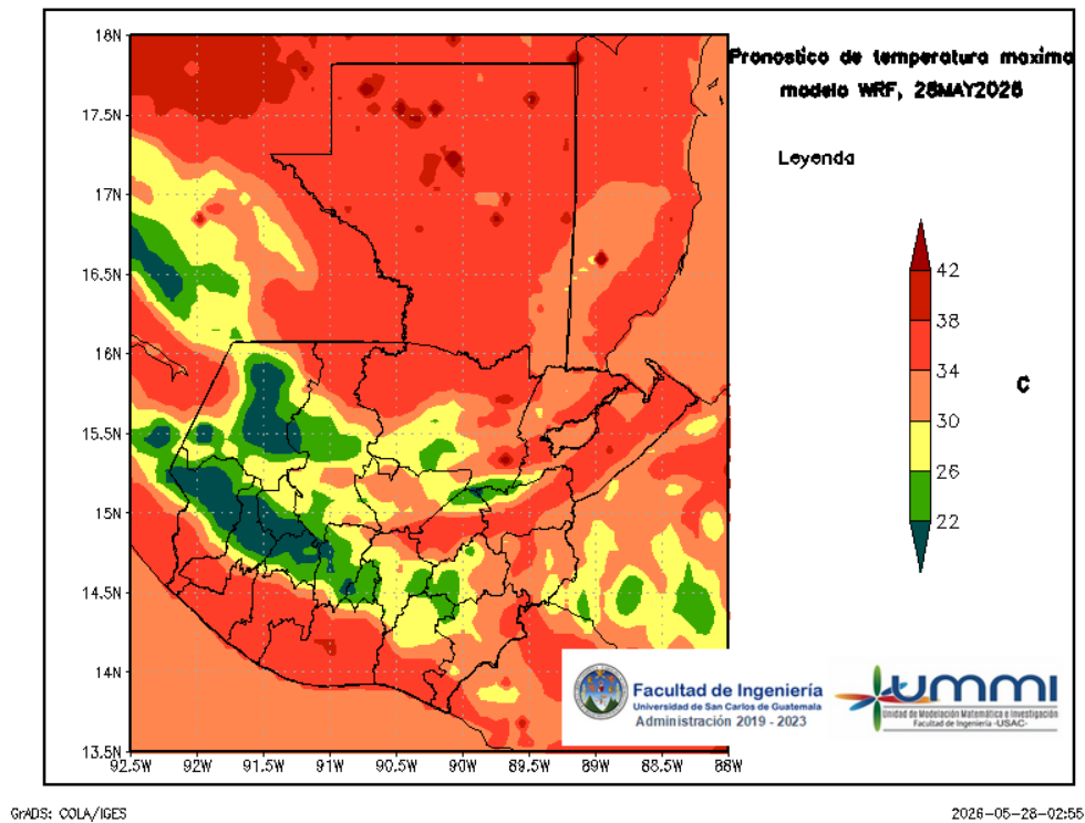
Figura 4: Pronóstico de temperatura máxima diaria del 28 de May
