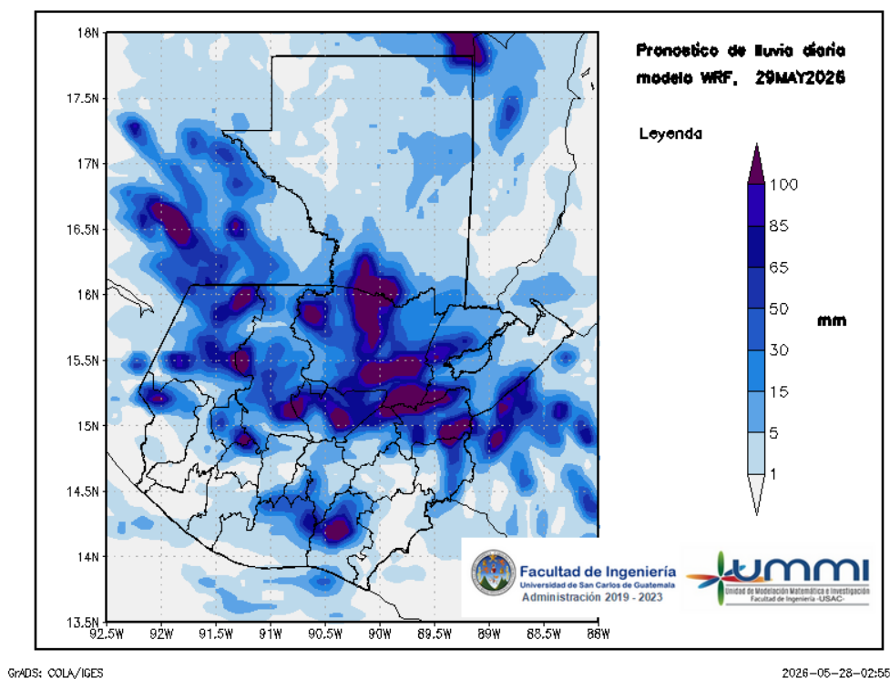
Figura 2: Pronóstico de lluvia diaria del 29 de May
