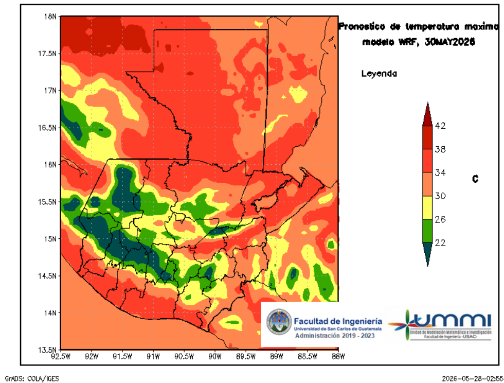
Figura 6: Pronóstico de temperatura máxima diaria del 30 de May
