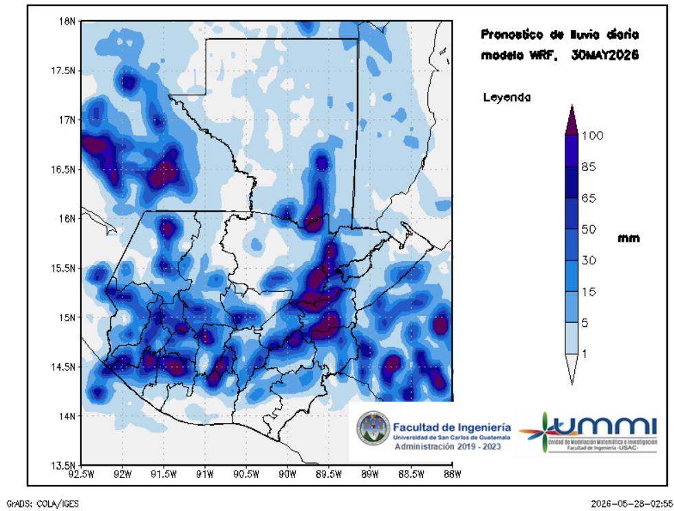
Figura 3: Pronóstico de lluvia diaria del 30 de May
