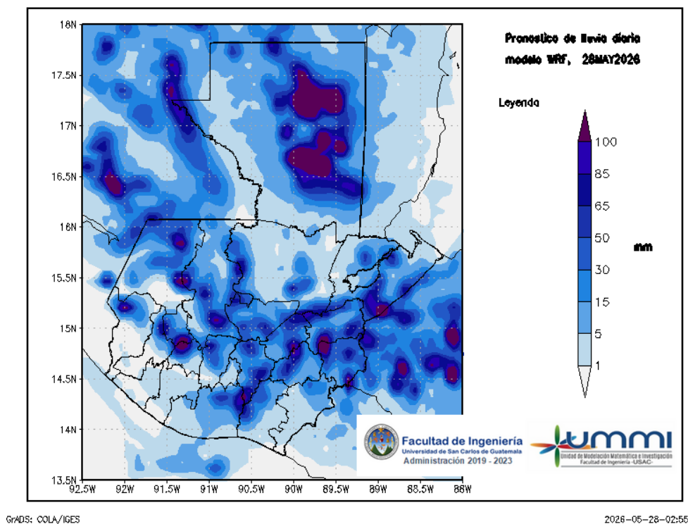
Figura 1: Pronóstico de lluvia diaria del 28 de May
