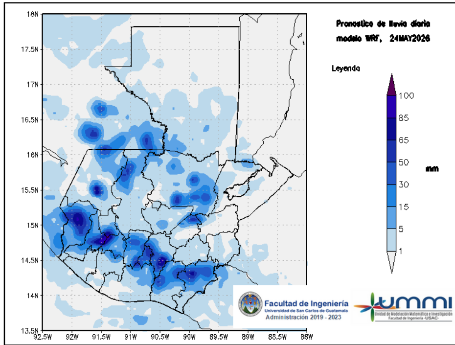
Figura 1: Pronóstico de lluvia diaria del 24 de May
