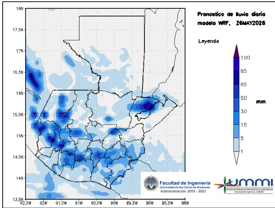
Figura 3: Pronóstico de lluvia diaria del 26 de May
