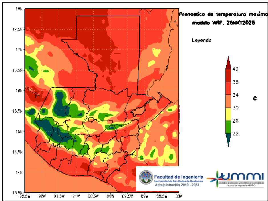
Figura 5: Pronóstico de temperatura máxima diaria del 25 de May
