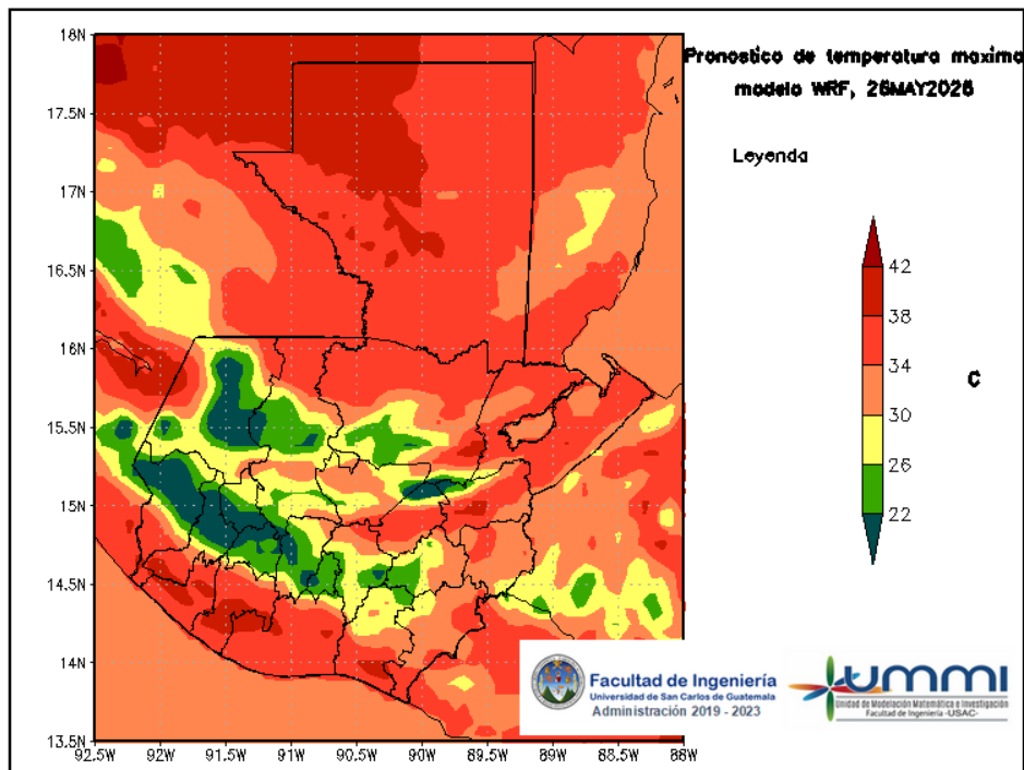
Figura 6: Pronóstico de temperatura máxima diaria del 26 de May
