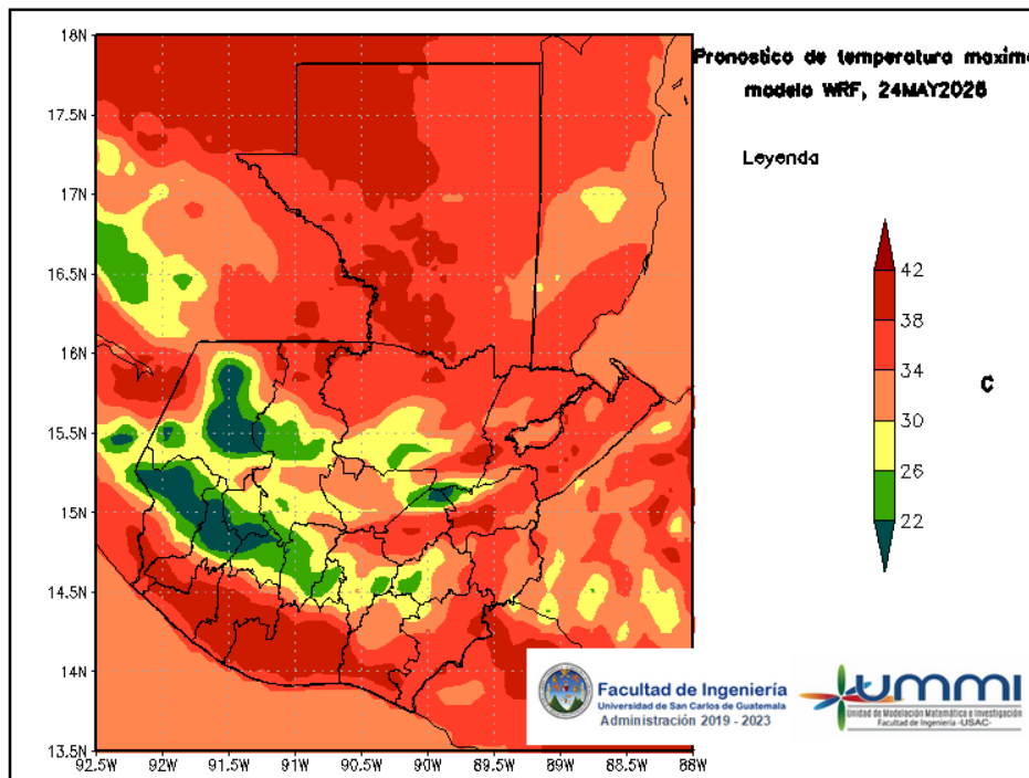
Figura 4: Pronóstico de temperatura máxima diaria del 24 de May
