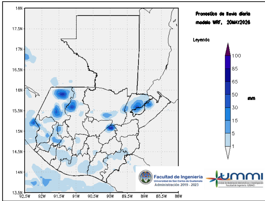
Figura 1: Pronóstico de lluvia diaria del 20 de May
