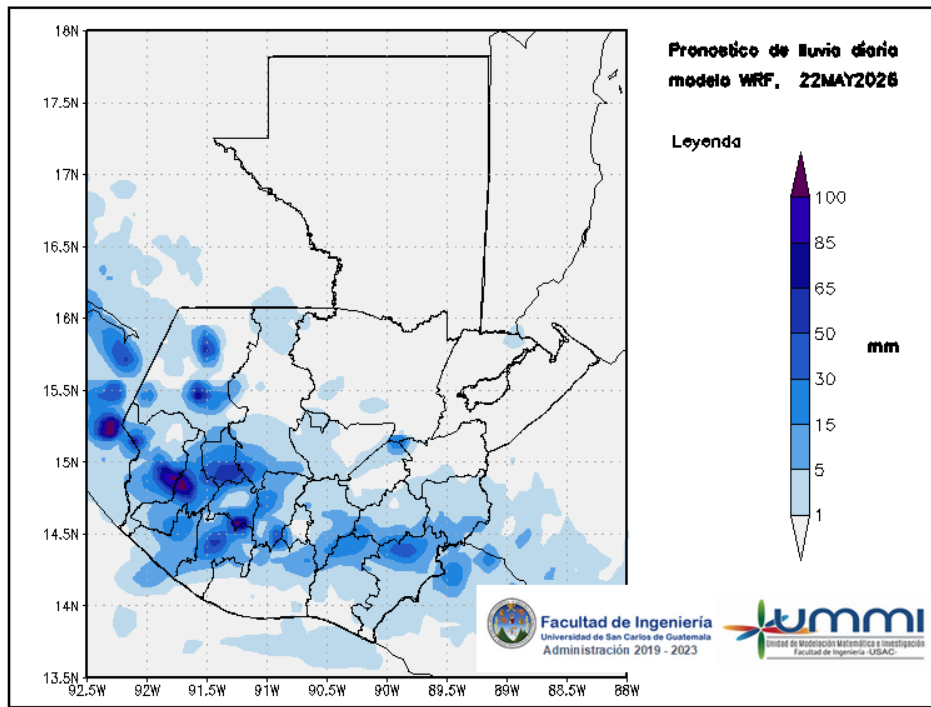
Figura 3: Pronóstico de lluvia diaria del 22 de May
