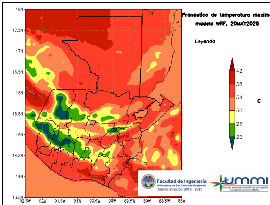
Figura 4: Pronóstico de temperatura máxima diaria del 20 de May
