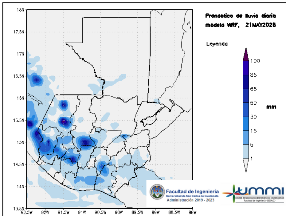
Figura 2: Pronóstico de lluvia diaria del 21 de May
