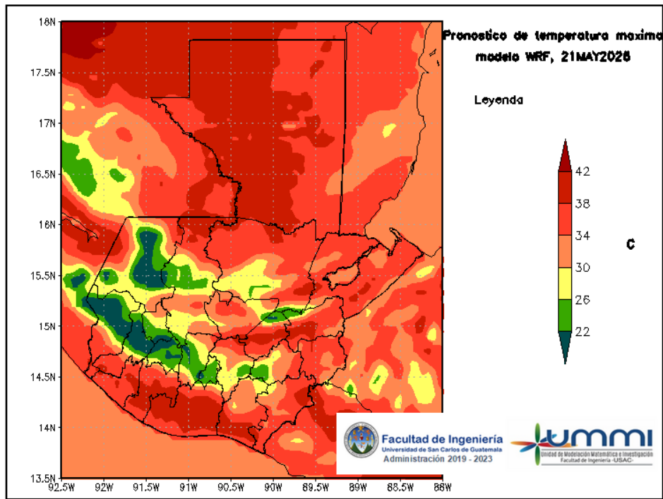
Figura 5: Pronóstico de temperatura máxima diaria del 21 de May
