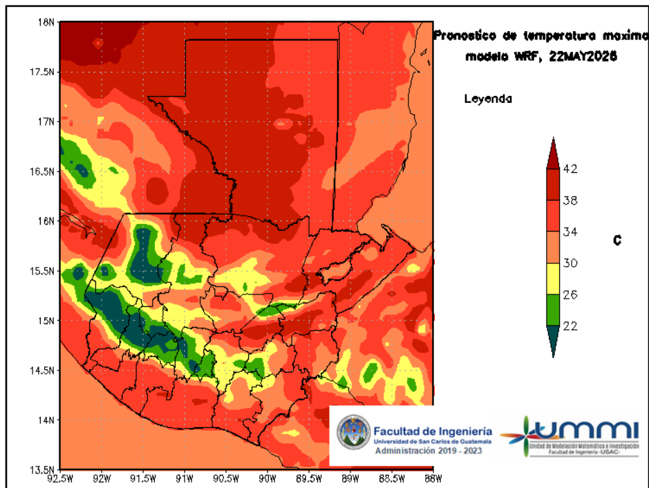
Figura 6: Pronóstico de temperatura máxima diaria del 22 de May
