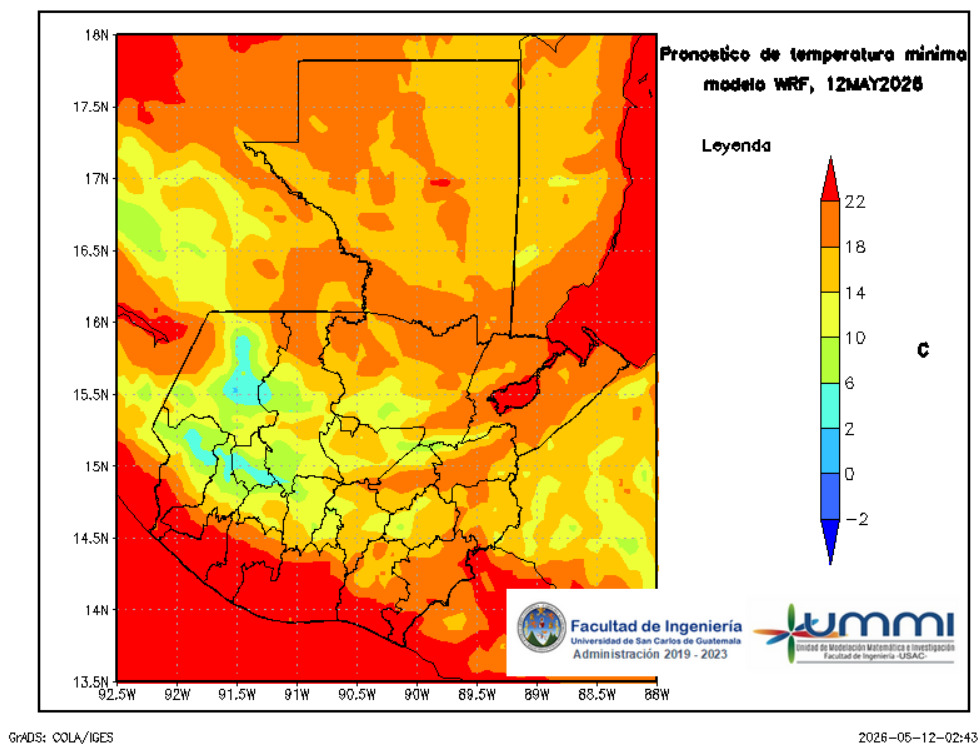
Figura 7: Pronóstico de temperatura mínima diaria del 13 de May
