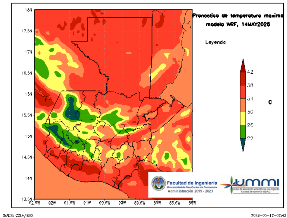
Figura 6: Pronóstico de temperatura máxima diaria del 14 de May
