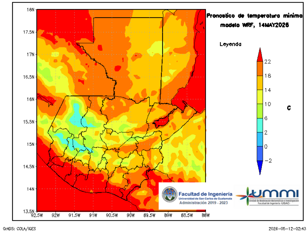
Figura 9: Pronóstico de temperatura mínima diaria del 15 de May
