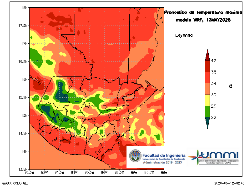
Figura 5: Pronóstico de temperatura máxima diaria del 13 de May
