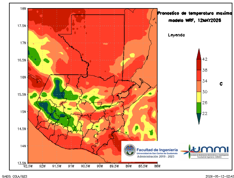
Figura 4: Pronóstico de temperatura máxima diaria del 12 de May
