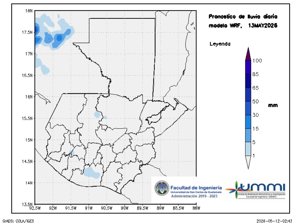
Figura 2: Pronóstico de lluvia diaria del 13 de May
