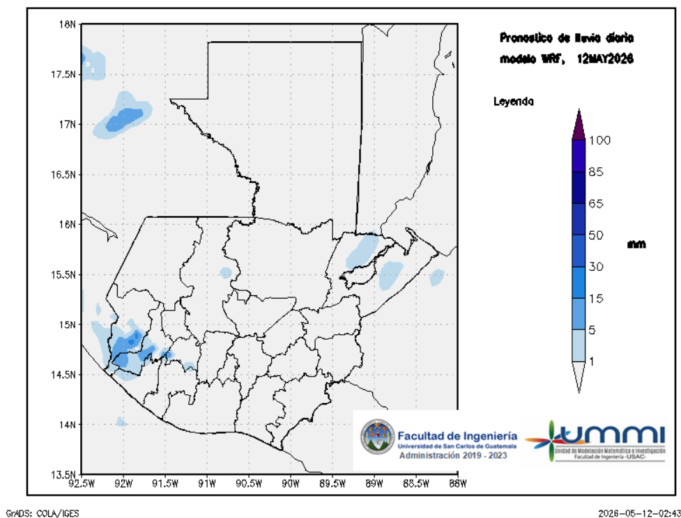
Figura 1: Pronóstico de lluvia diaria del 12 de May
