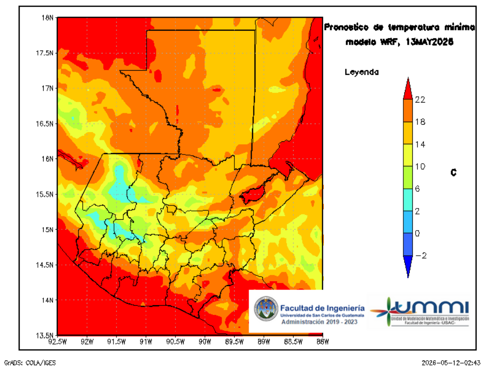
Figura 8: Pronóstico de temperatura mínima diaria del 14 de May
