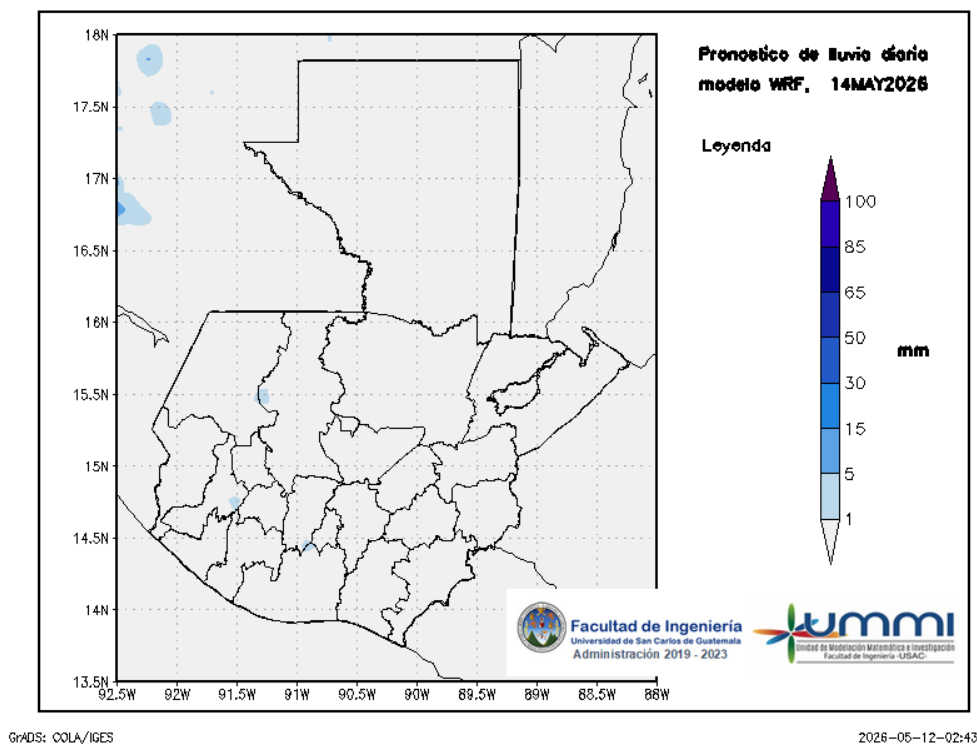
Figura 3: Pronóstico de lluvia diaria del 14 de May
