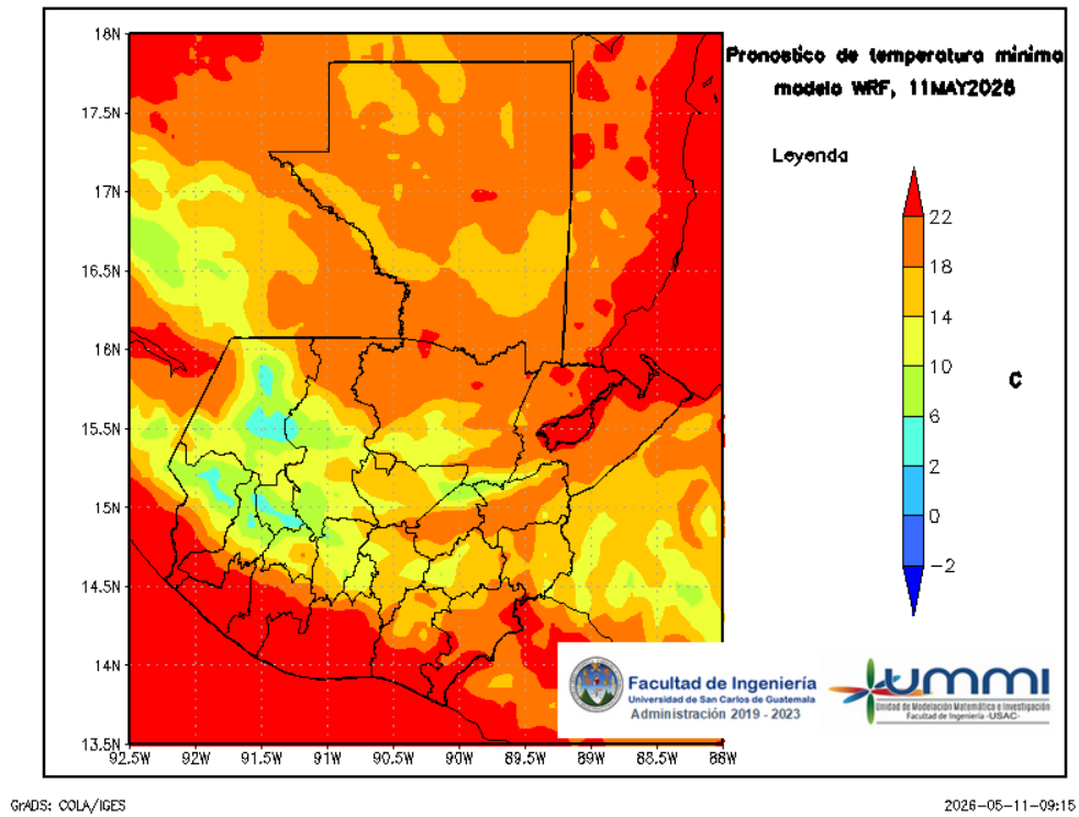
Figura 7: Pronóstico de temperatura mínima diaria del 12 de May
