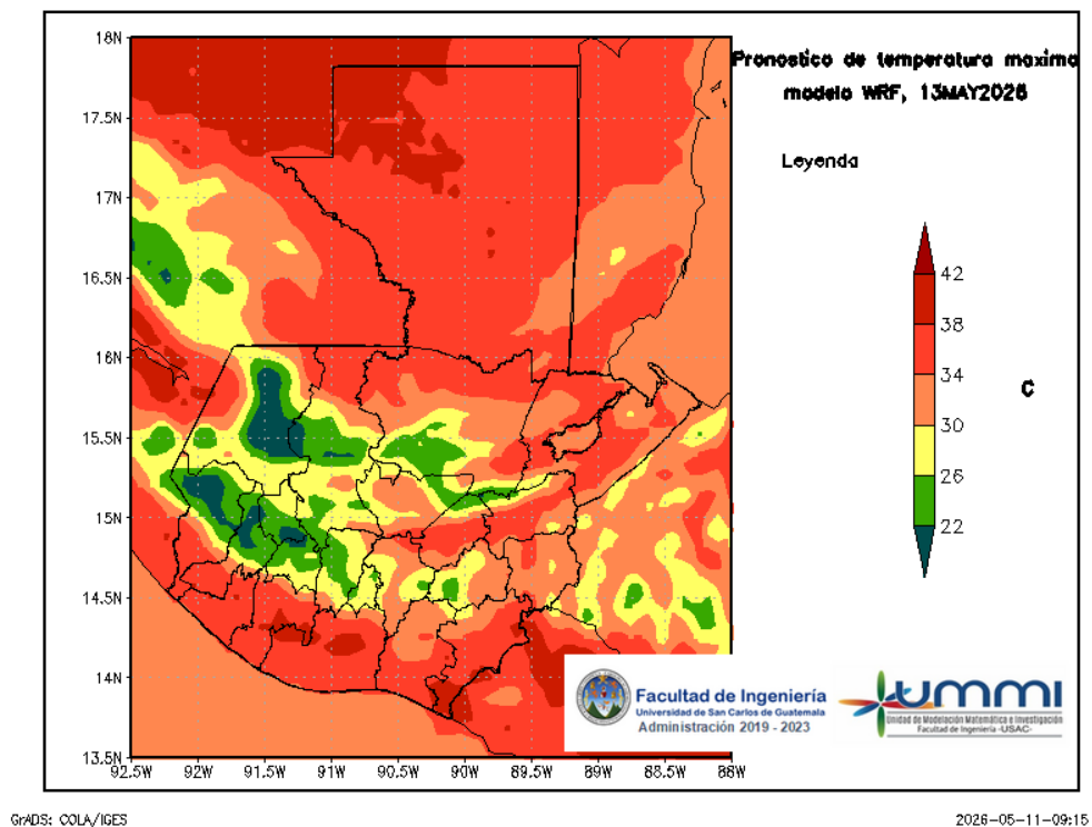
Figura 6: Pronóstico de temperatura máxima diaria del 13 de May
