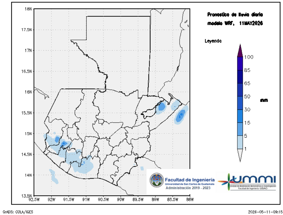
Figura 1: Pronóstico de lluvia diaria del 11 de May
