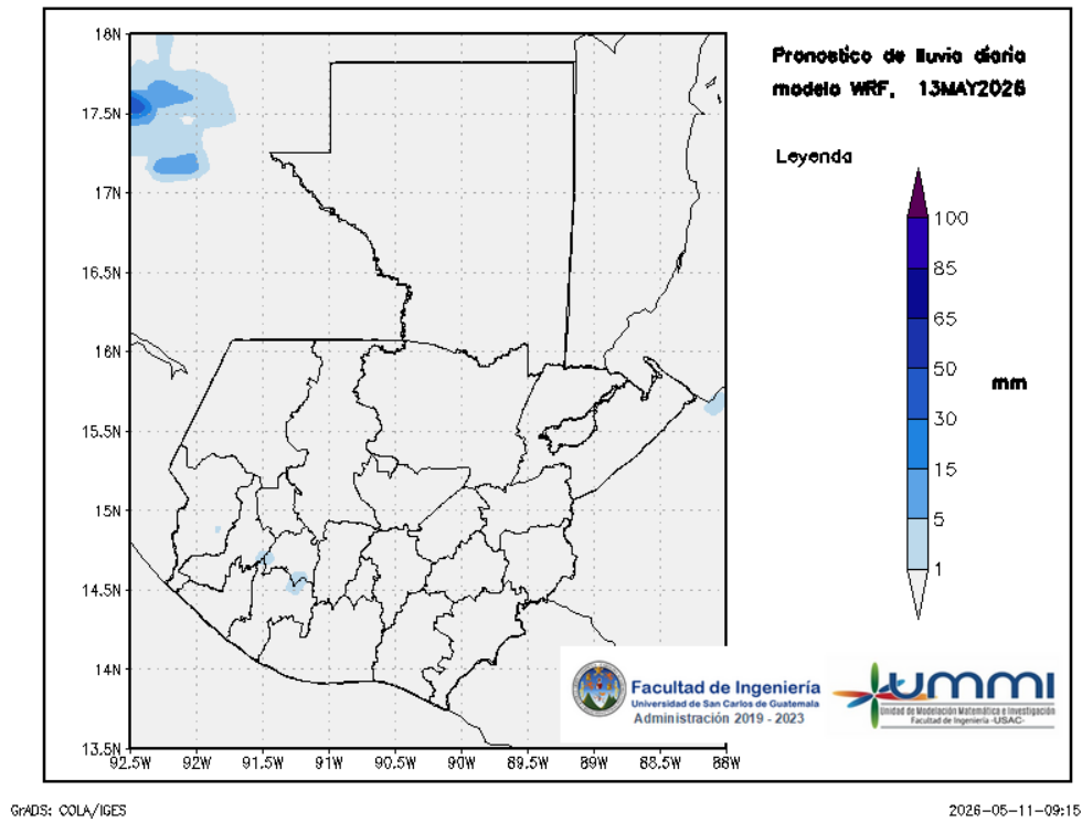
Figura 3: Pronóstico de lluvia diaria del 13 de May
