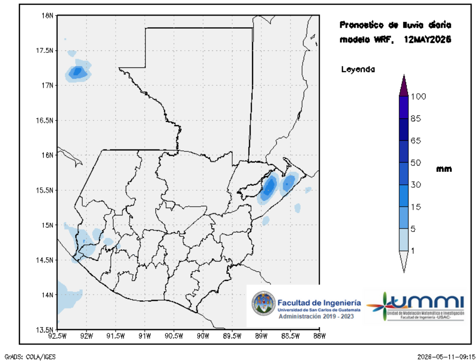
Figura 2: Pronóstico de lluvia diaria del 12 de May
