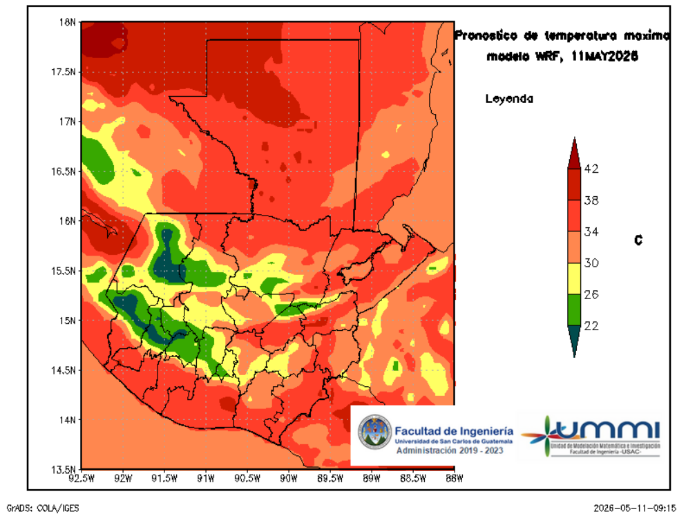
Figura 4: Pronóstico de temperatura máxima diaria del 11 de May
