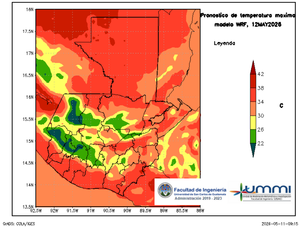
Figura 5: Pronóstico de temperatura máxima diaria del 12 de May
