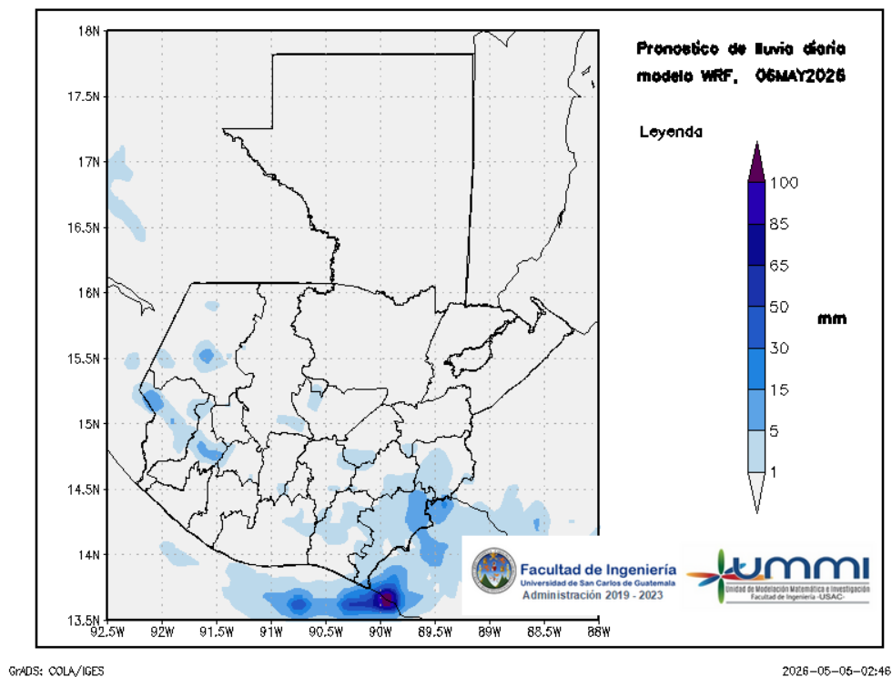
Figura 2: Pronóstico de lluvia diaria del 06 de May
