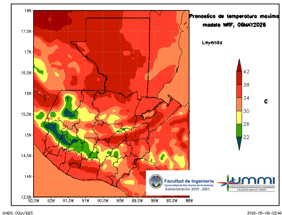
Figura 5: Pronóstico de temperatura máxima diaria del 06 de May
