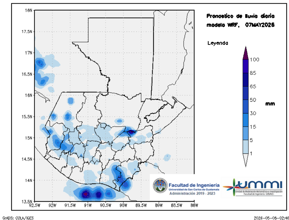
Figura 3: Pronóstico de lluvia diaria del 07 de May
