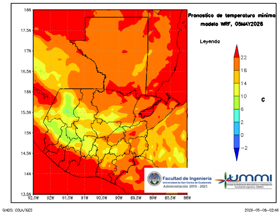
Figura 7: Pronóstico de temperatura mínima diaria del 06 de May
