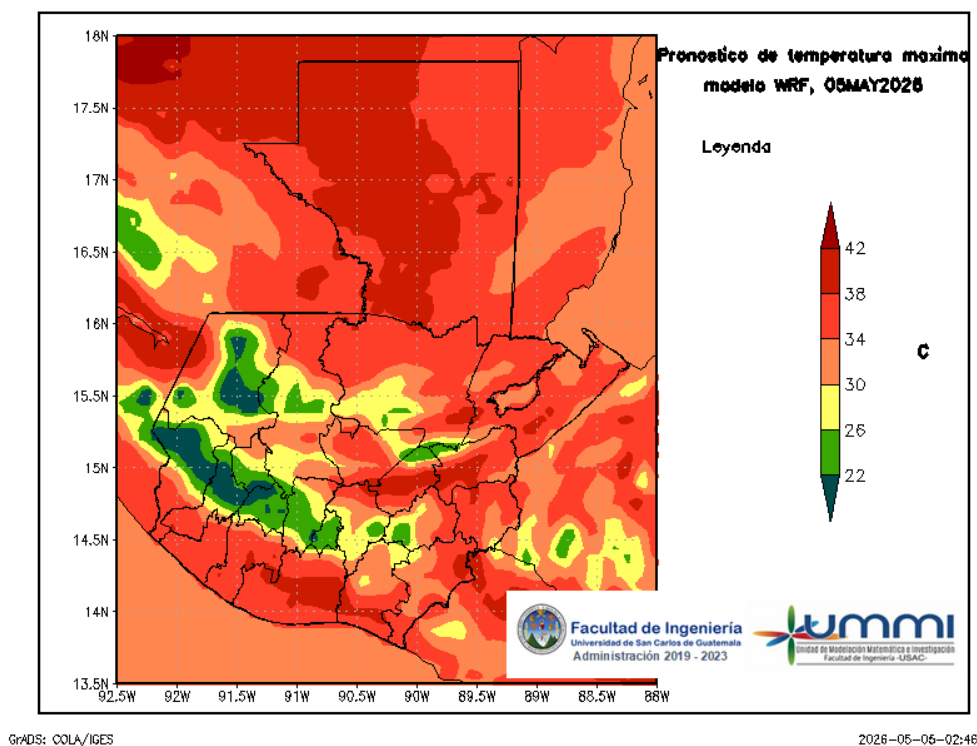
Figura 4: Pronóstico de temperatura máxima diaria del 05 de May
