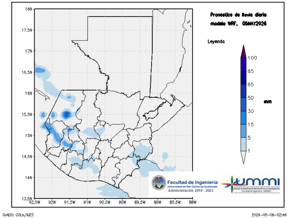
Figura 1: Pronóstico de lluvia diaria del 05 de May
