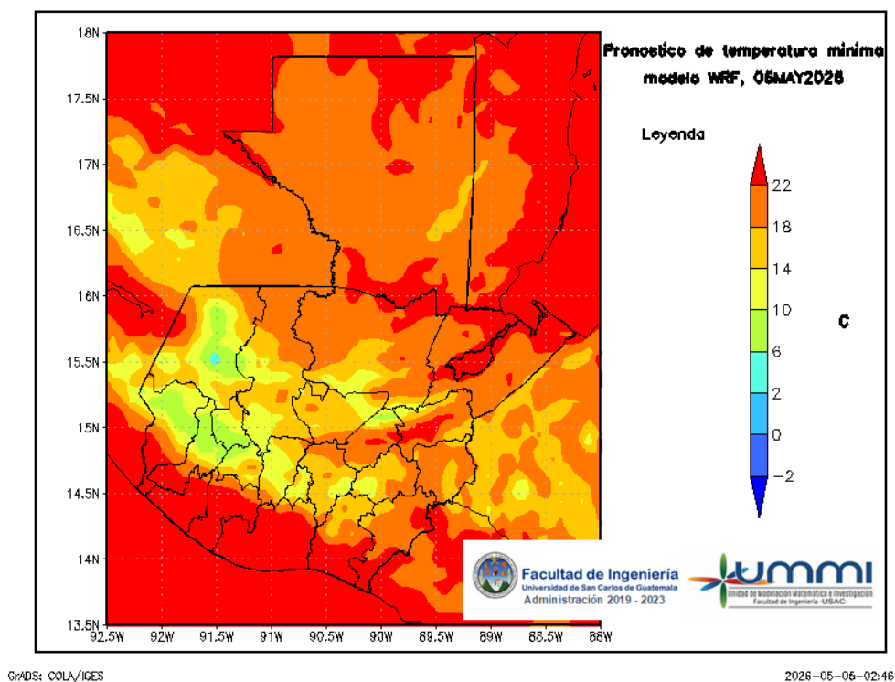
Figura 8: Pronóstico de temperatura mínima diaria del 07 de May
