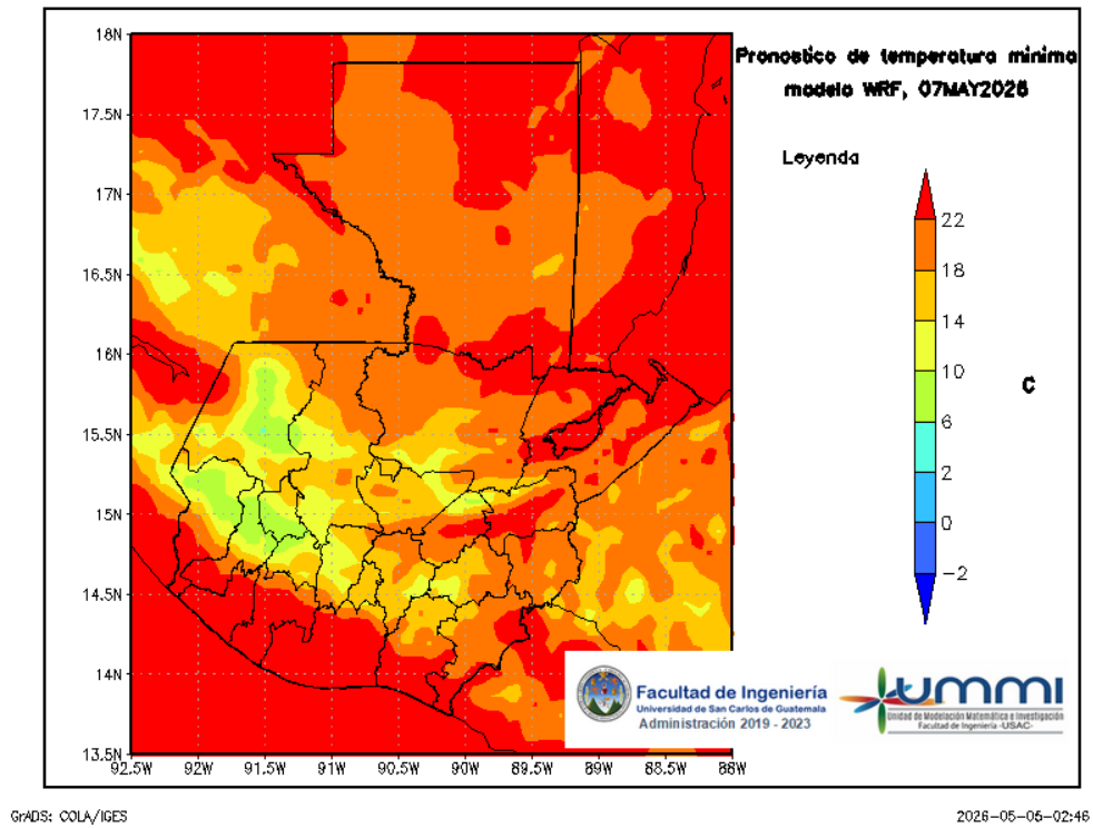
Figura 9: Pronóstico de temperatura mínima diaria del 08 de May
