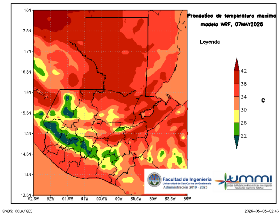
Figura 6: Pronóstico de temperatura máxima diaria del 07 de May
