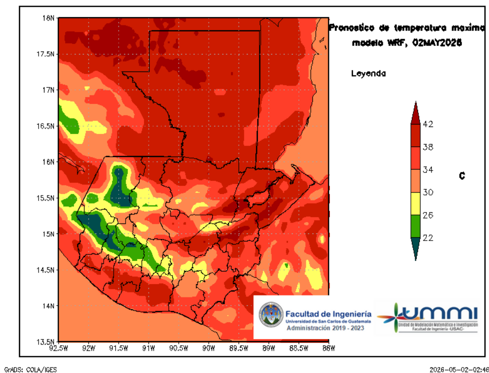
Figura 4: Pronóstico de temperatura máxima diaria del 02 de May
