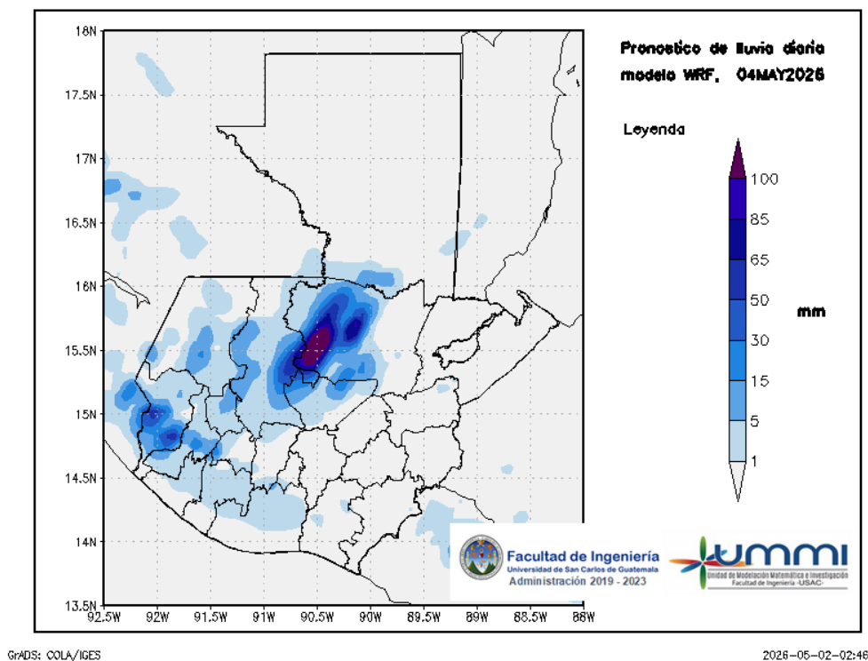
Figura 3: Pronóstico de lluvia diaria del 04 de May
