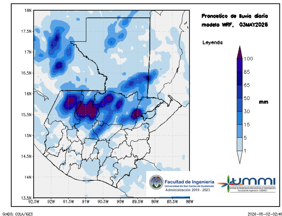
Figura 2: Pronóstico de lluvia diaria del 03 de May
