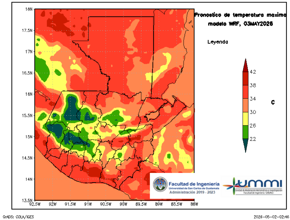
Figura 5: Pronóstico de temperatura máxima diaria del 03 de May
