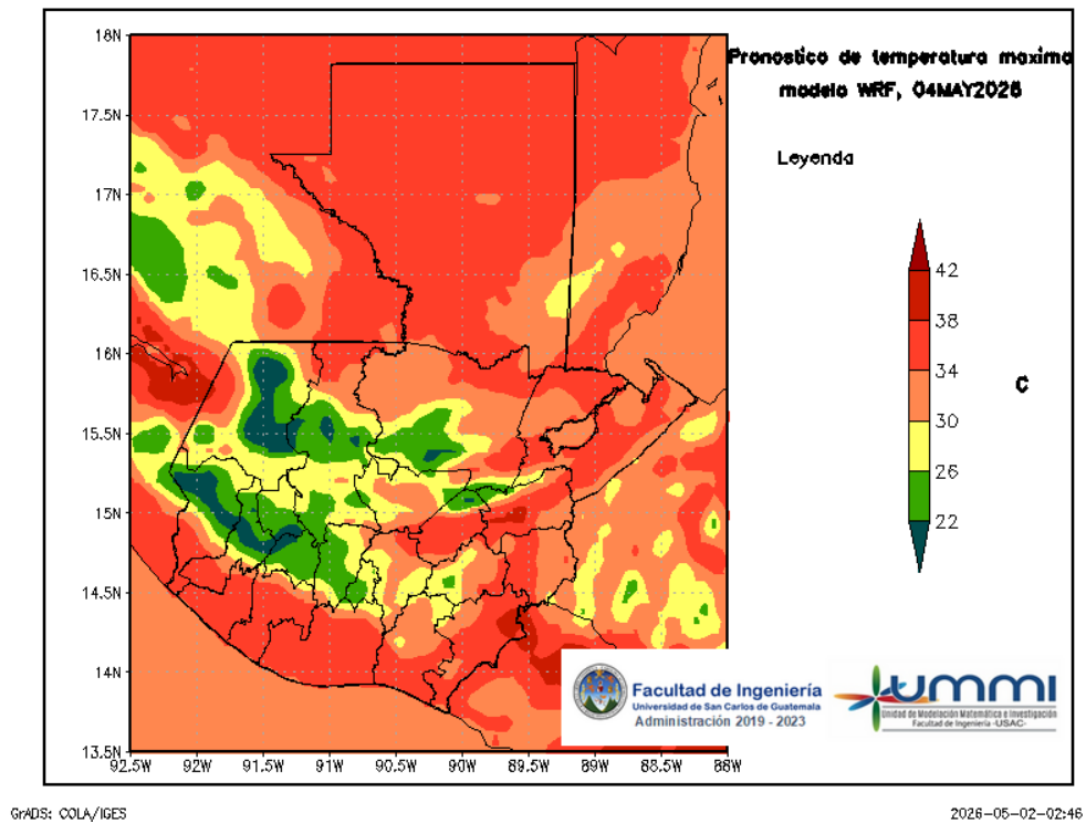
Figura 6: Pronóstico de temperatura máxima diaria del 04 de May
