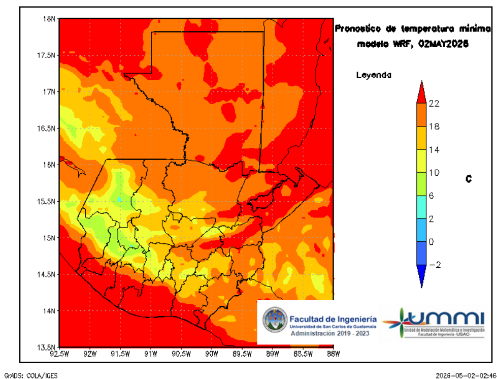
Figura 7: Pronóstico de temperatura mínima diaria del 03 de May
