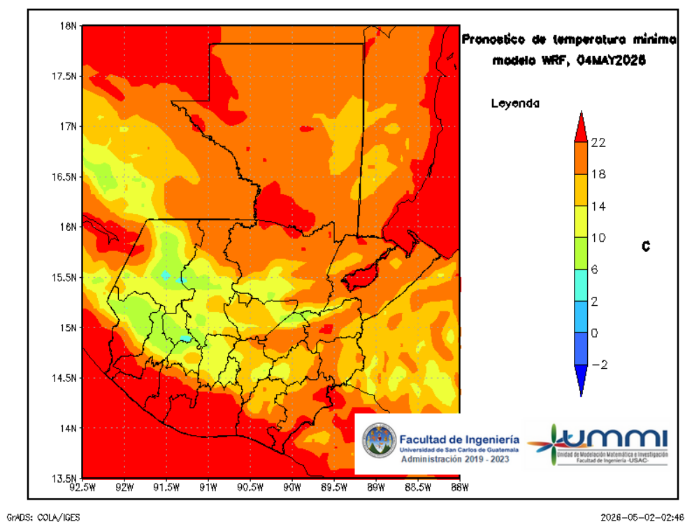
Figura 9: Pronóstico de temperatura mínima diaria del 05 de May
