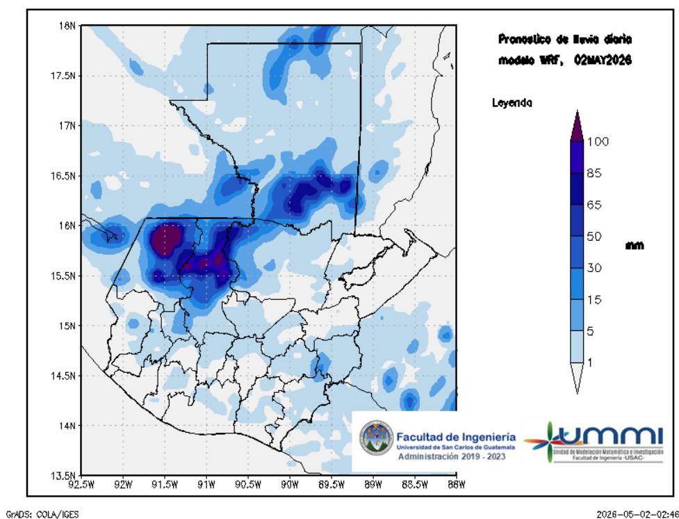
Figura 1: Pronóstico de lluvia diaria del 02 de May
