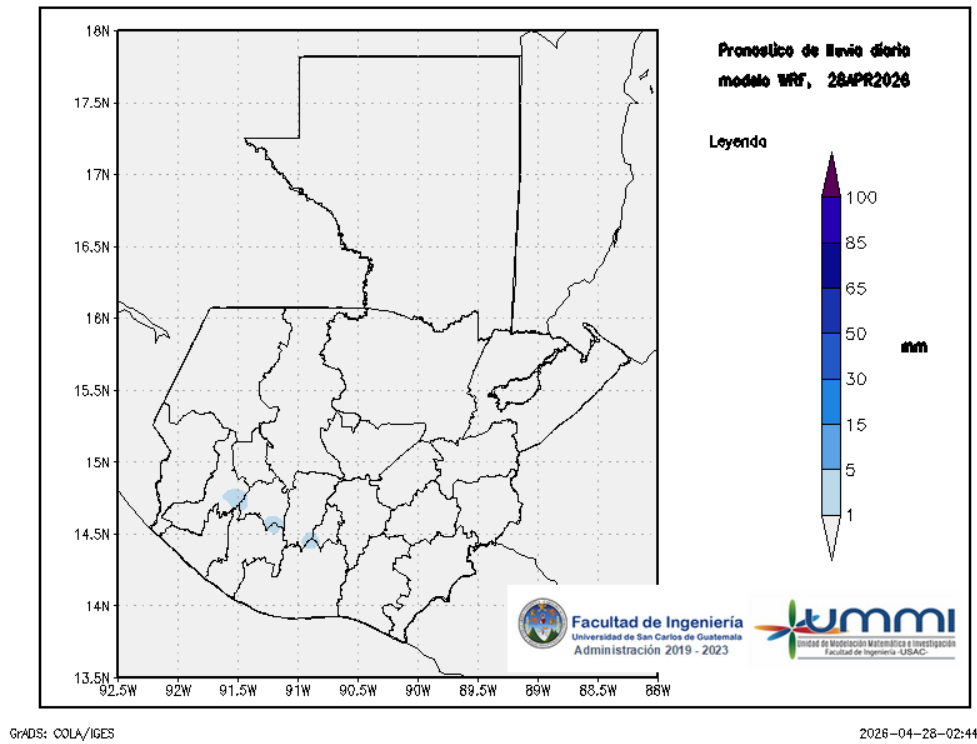
Figura 1: Pronóstico de lluvia diaria del 28 de April
