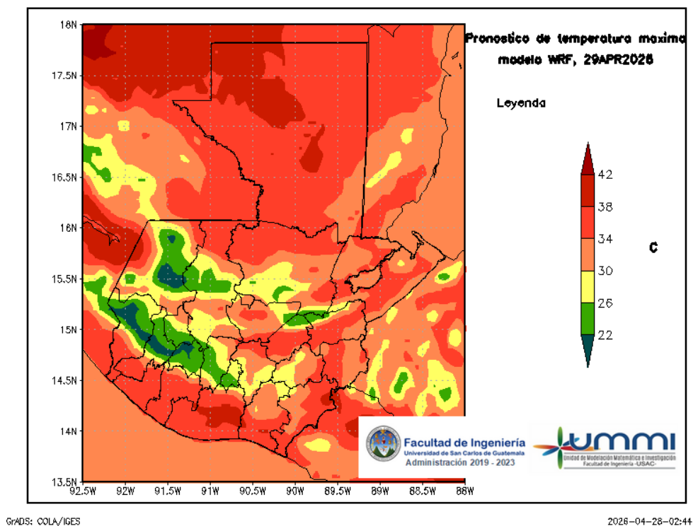
Figura 5: Pronóstico de temperatura máxima diaria del 29 de April
