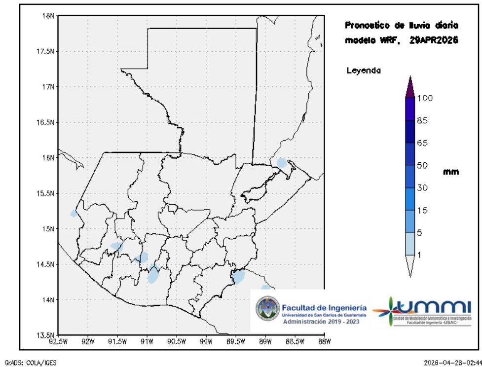
Figura 2: Pronóstico de lluvia diaria del 29 de April
