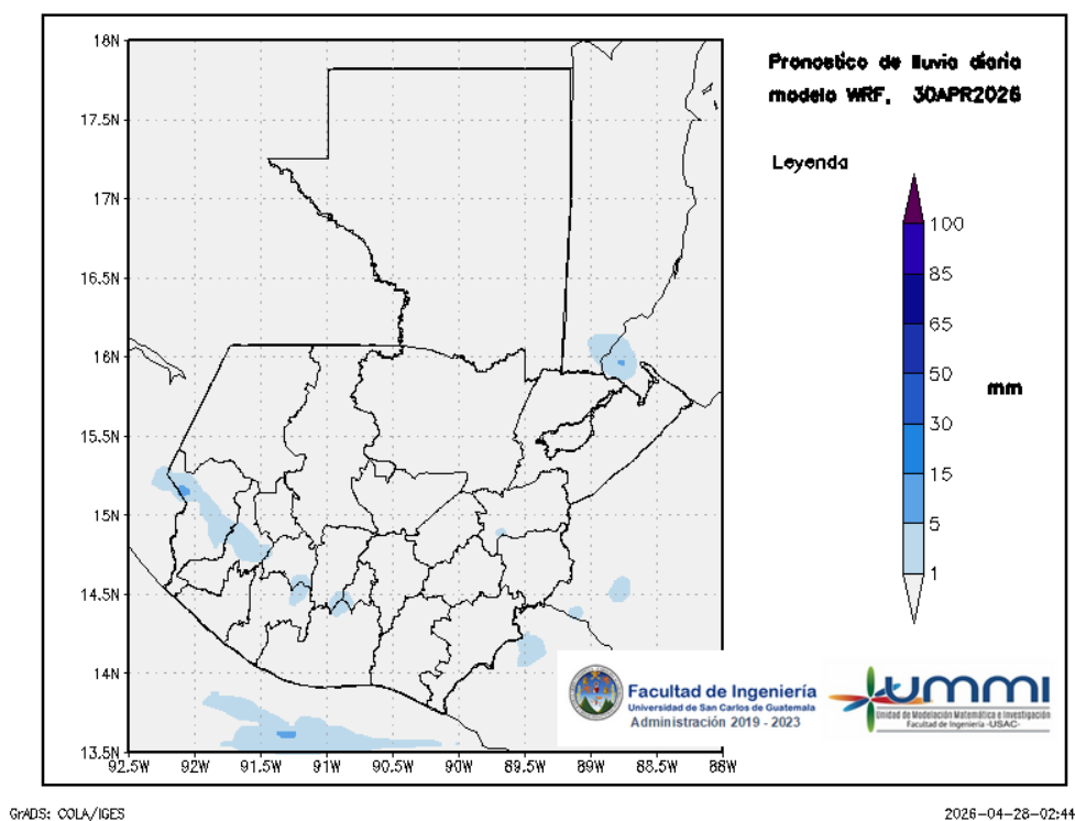
Figura 3: Pronóstico de lluvia diaria del 30 de April
