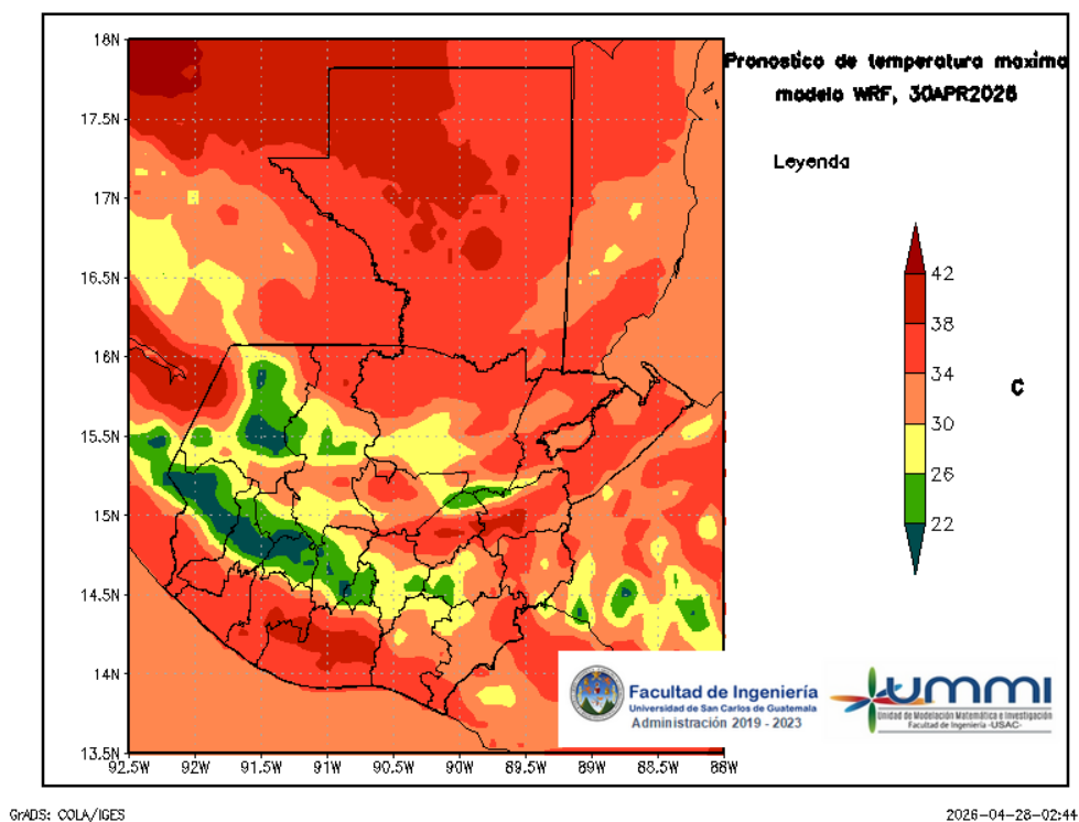
Figura 6: Pronóstico de temperatura máxima diaria del 30 de April
