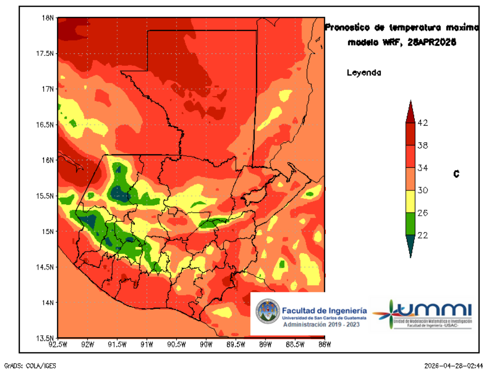
Figura 4: Pronóstico de temperatura máxima diaria del 28 de April
