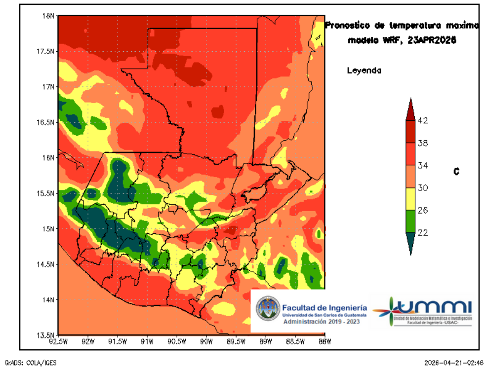
Figura 6: Pronóstico de temperatura máxima diaria del 23 de April
