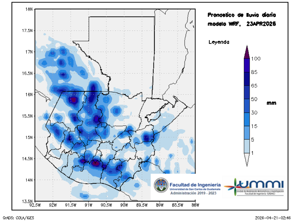
Figura 3: Pronóstico de lluvia diaria del 23 de April
