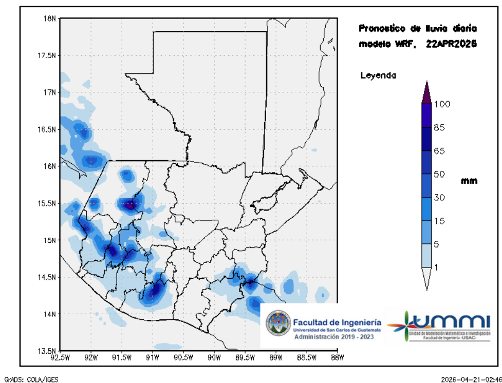
Figura 2: Pronóstico de lluvia diaria del 22 de April
