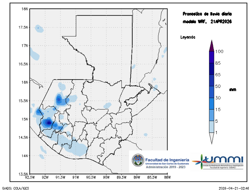
Figura 1: Pronóstico de lluvia diaria del 21 de April
