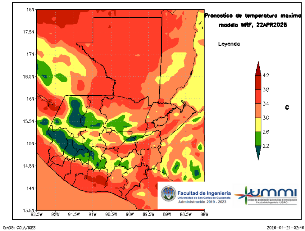
Figura 5: Pronóstico de temperatura máxima diaria del 22 de April
