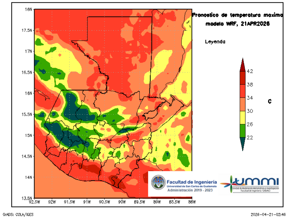
Figura 4: Pronóstico de temperatura máxima diaria del 21 de April
