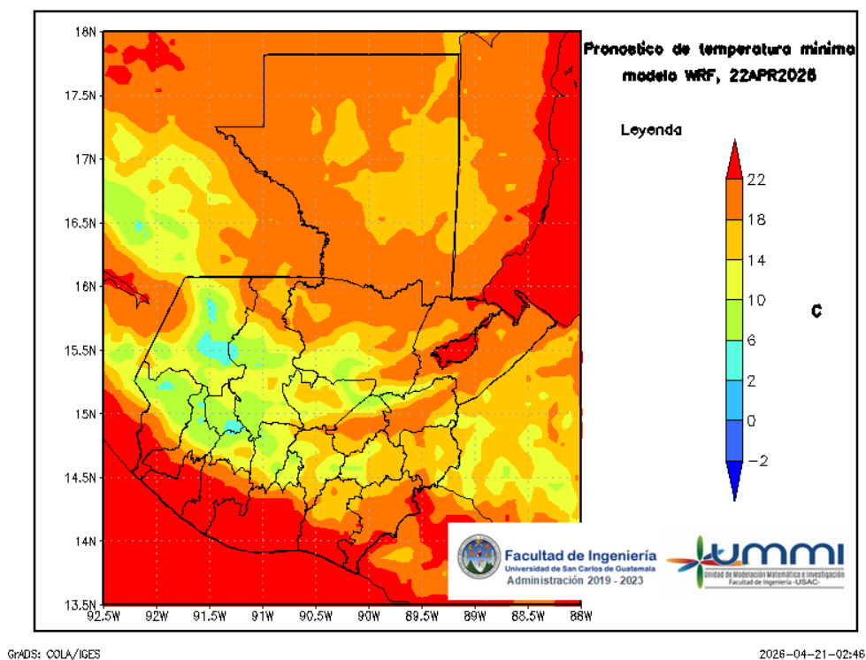
Figura 8: Pronóstico de temperatura mínima diaria del 23 de April
