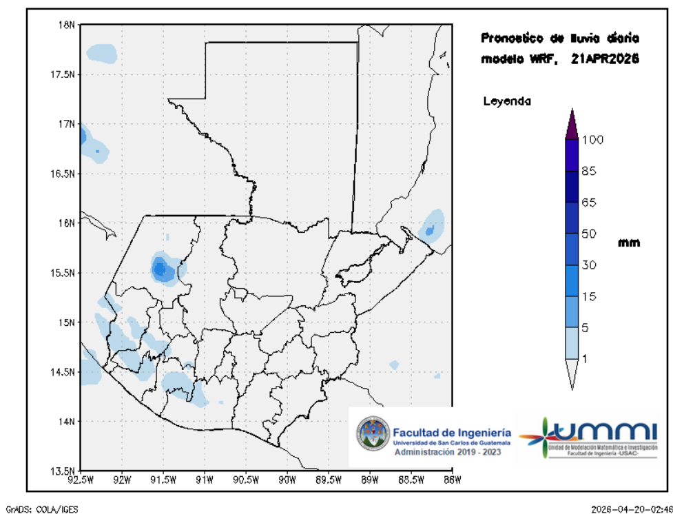
Figura 2: Pronóstico de lluvia diaria del 21 de April
