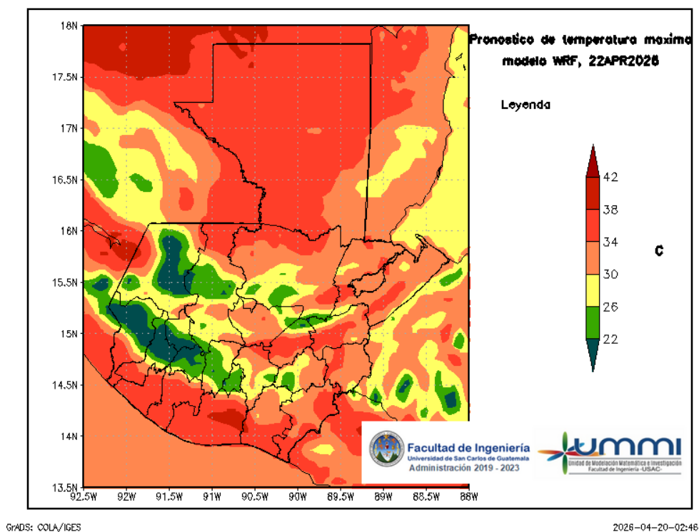
Figura 6: Pronóstico de temperatura máxima diaria del 22 de April
