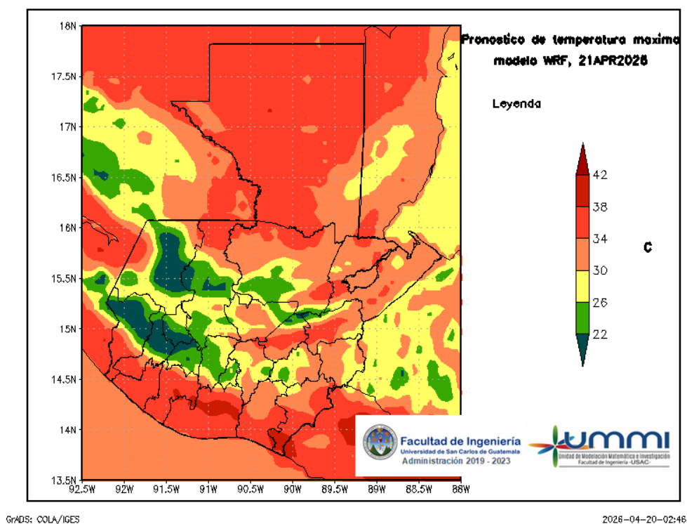
Figura 5: Pronóstico de temperatura máxima diaria del 21 de April
