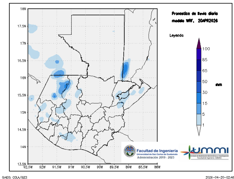
Figura 1: Pronóstico de lluvia diaria del 20 de April
