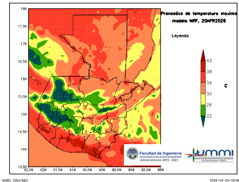
Figura 4: Pronóstico de temperatura máxima diaria del 20 de April
