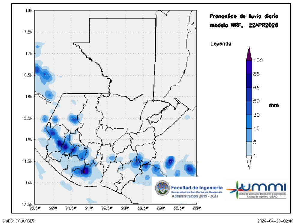
Figura 3: Pronóstico de lluvia diaria del 22 de April
