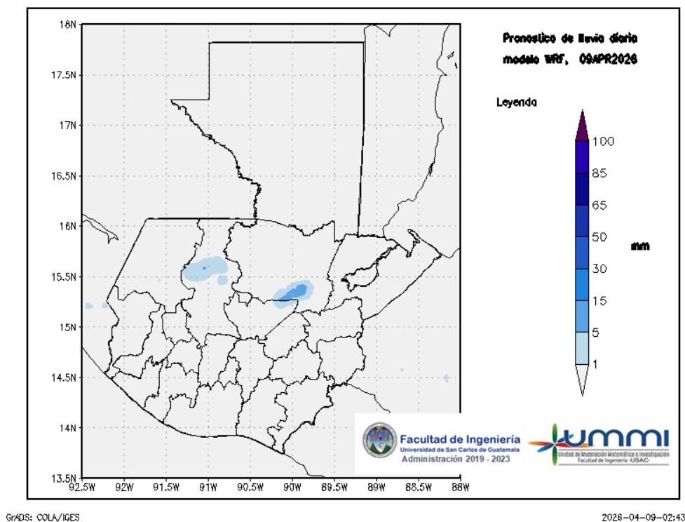
Figura 1: Pronóstico de lluvia diaria del 09 de April
