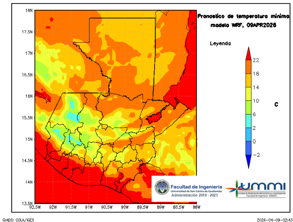
Figura 7: Pronóstico de temperatura mínima diaria del 10 de April
