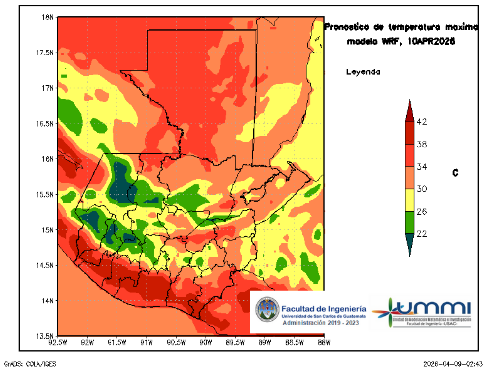
Figura 5: Pronóstico de temperatura máxima diaria del 10 de April
