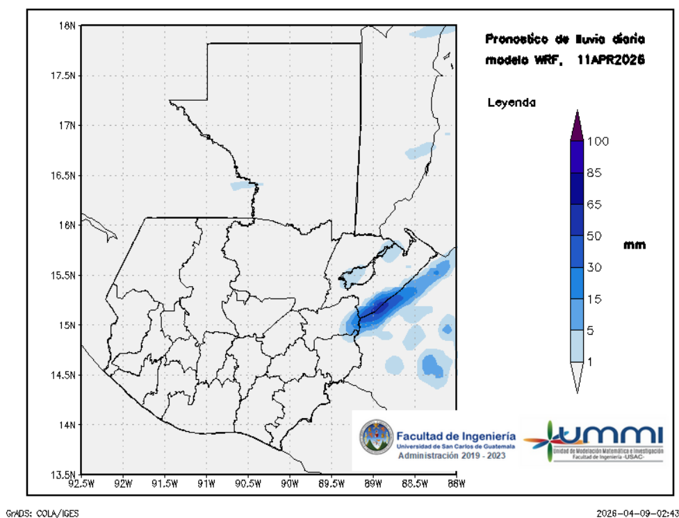
Figura 3: Pronóstico de lluvia diaria del 11 de April
