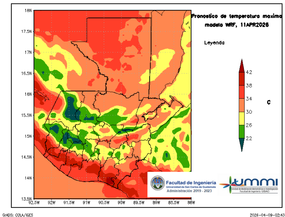
Figura 6: Pronóstico de temperatura máxima diaria del 11 de April
