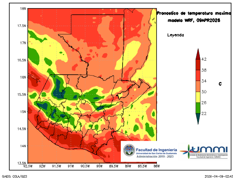
Figura 4: Pronóstico de temperatura máxima diaria del 09 de April
