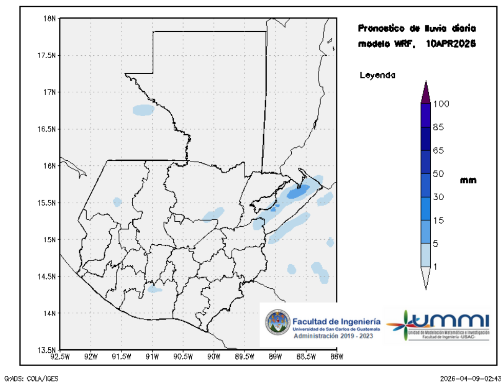
Figura 2: Pronóstico de lluvia diaria del 10 de April
