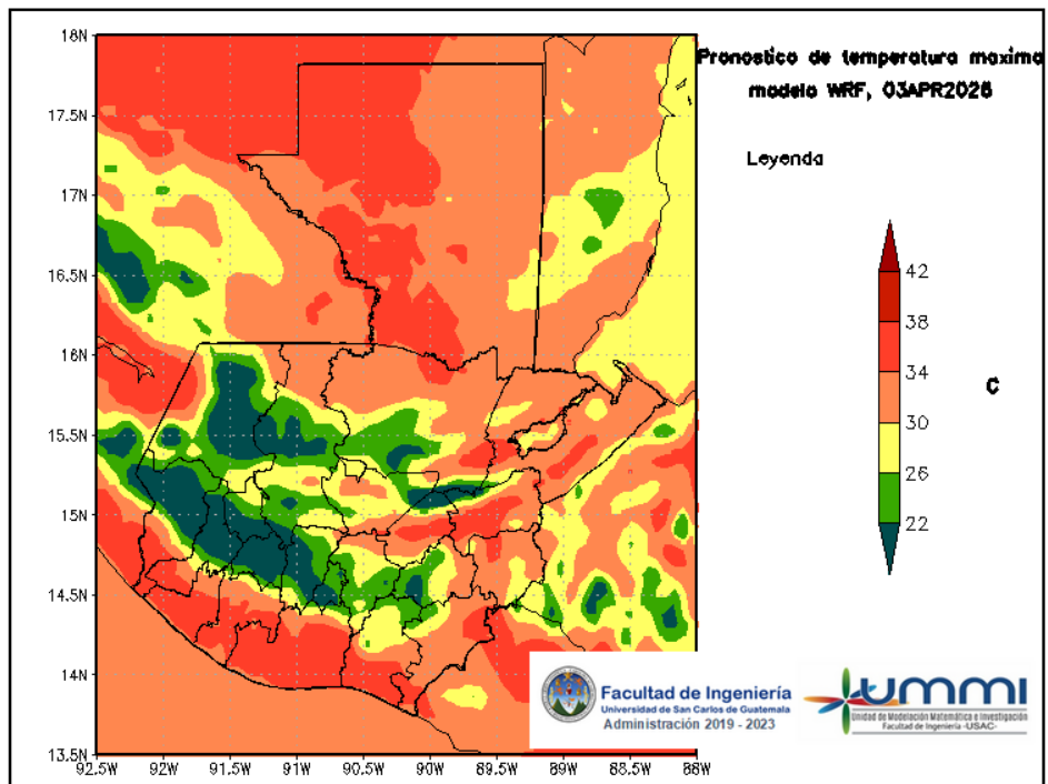
Figura 6: Pronóstico de temperatura máxima diaria del 03 de April
