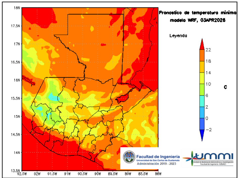
Figura 9: Pronóstico de temperatura mínima diaria del 04 de April
