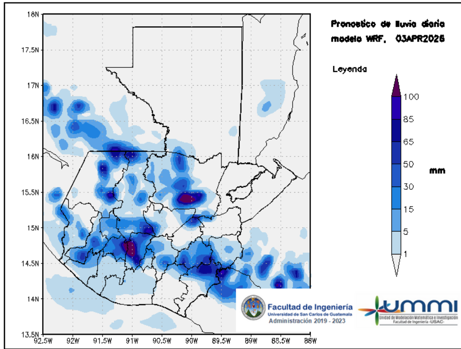
Figura 3: Pronóstico de lluvia diaria del 03 de April
