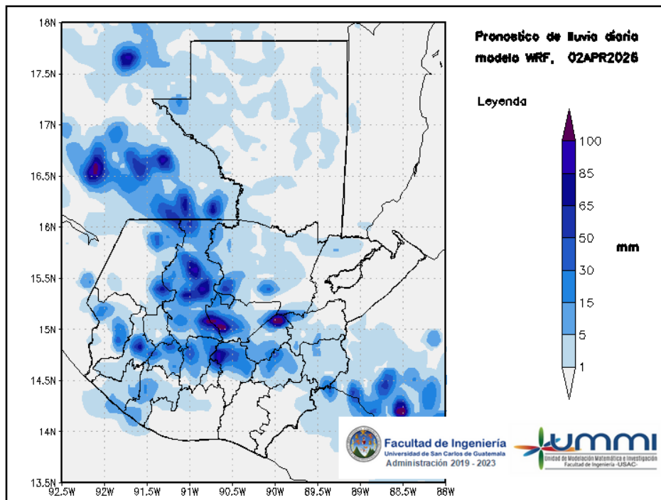
Figura 2: Pronóstico de lluvia diaria del 02 de April
