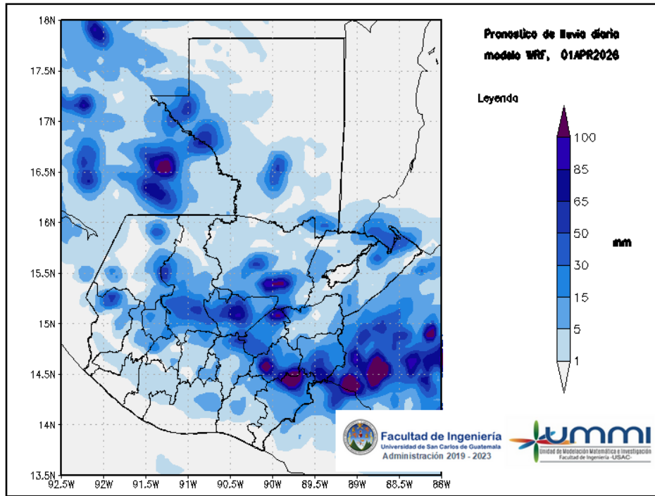
Figura 1: Pronóstico de lluvia diaria del 01 de April
