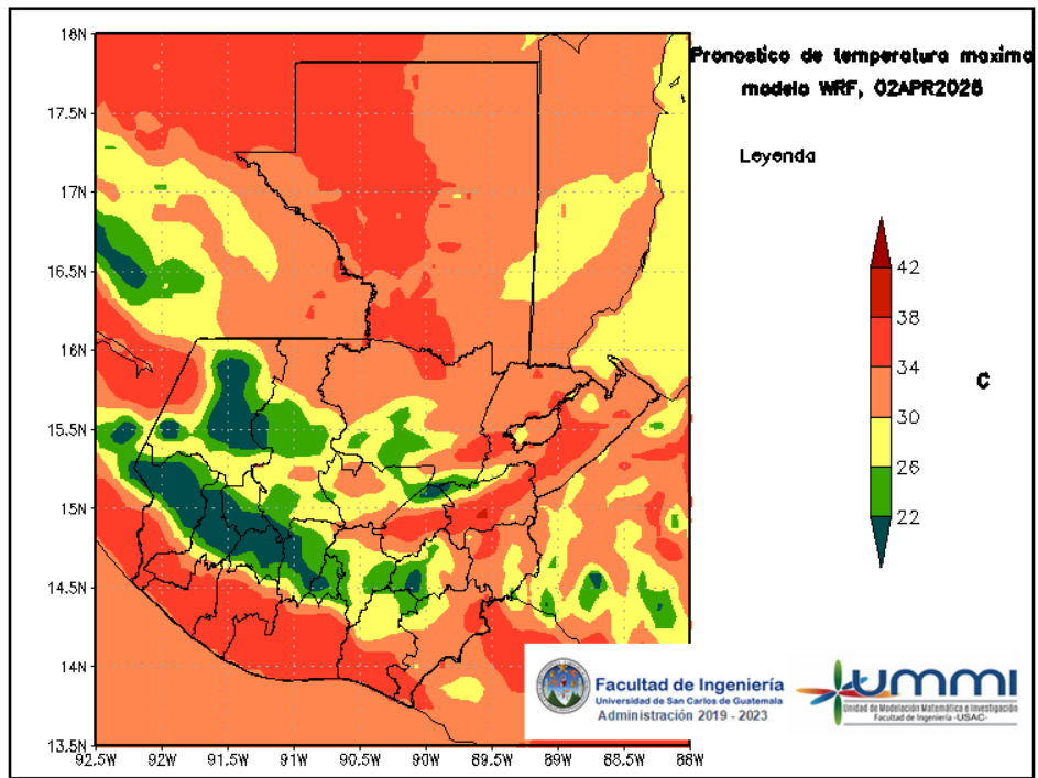
Figura 5: Pronóstico de temperatura máxima diaria del 02 de April
