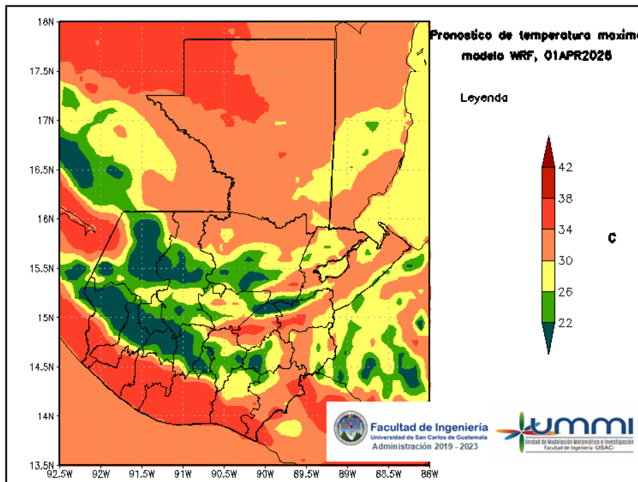
Figura 4: Pronóstico de temperatura máxima diaria del 01 de April
