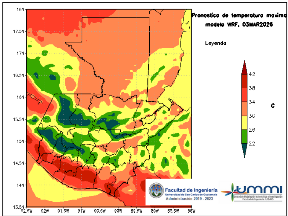
Figura 5: Pronóstico de temperatura máxima diaria del 03 de March
