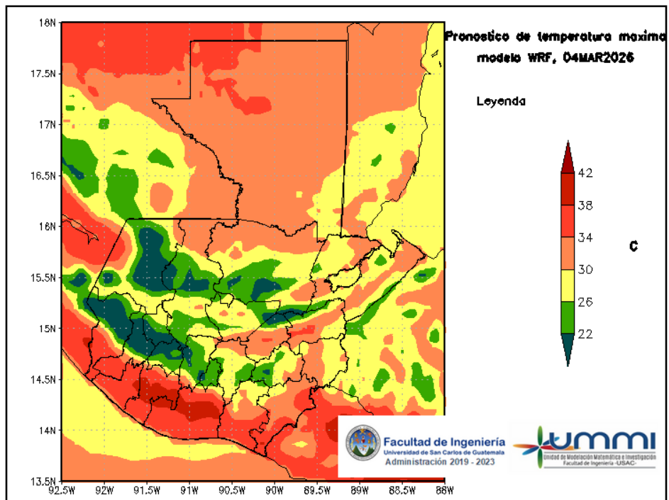
Figura 6: Pronóstico de temperatura máxima diaria del 04 de March
