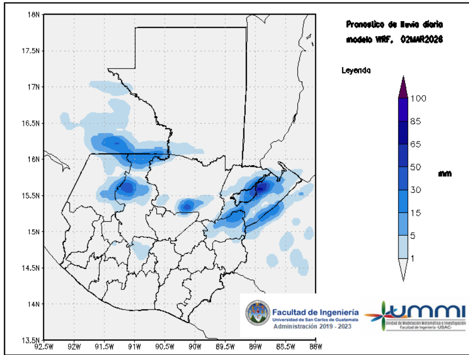
Figura 1: Pronóstico de lluvia diaria del 02 de March
