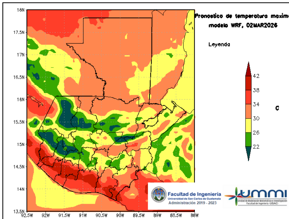
Figura 4: Pronóstico de temperatura máxima diaria del 02 de March
