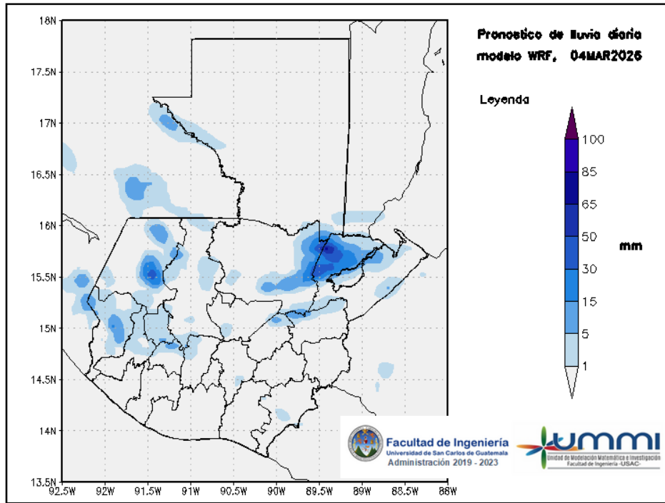
Figura 3: Pronóstico de lluvia diaria del 04 de March
