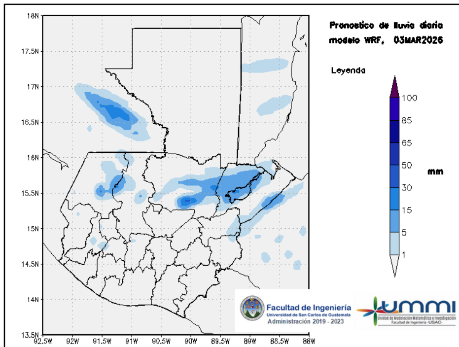
Figura 2: Pronóstico de lluvia diaria del 03 de March
