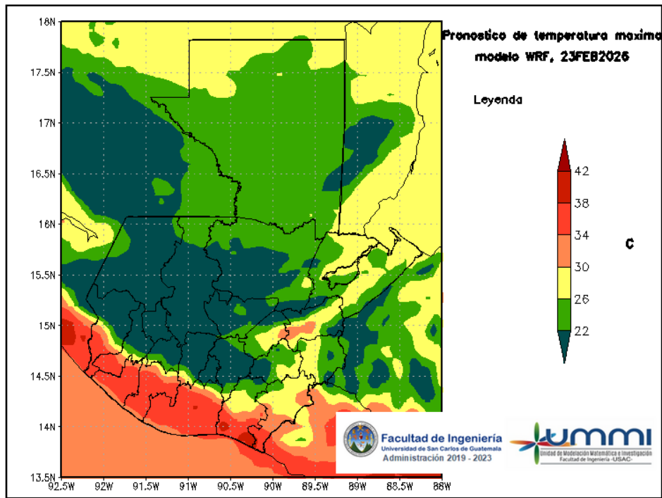
Figura 5: Pronóstico de temperatura máxima diaria del 23 de February
