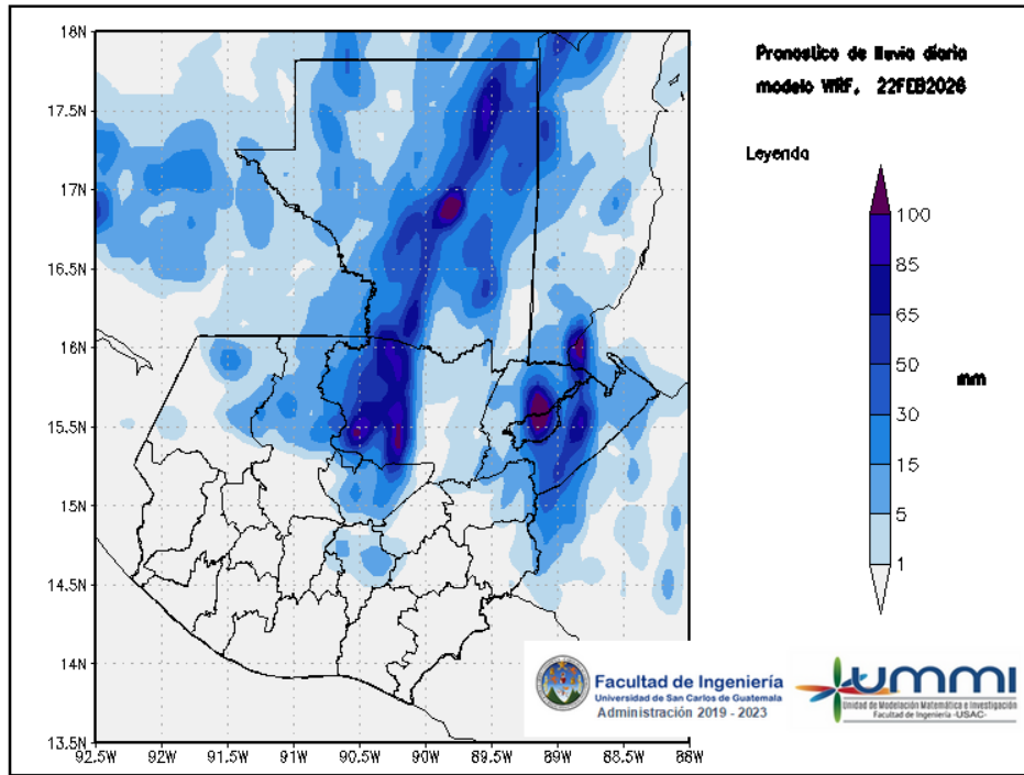
Figura 1: Pronóstico de lluvia diaria del 22 de February
