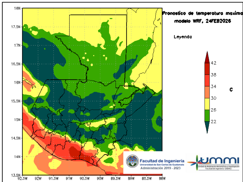
Figura 6: Pronóstico de temperatura máxima diaria del 24 de February
