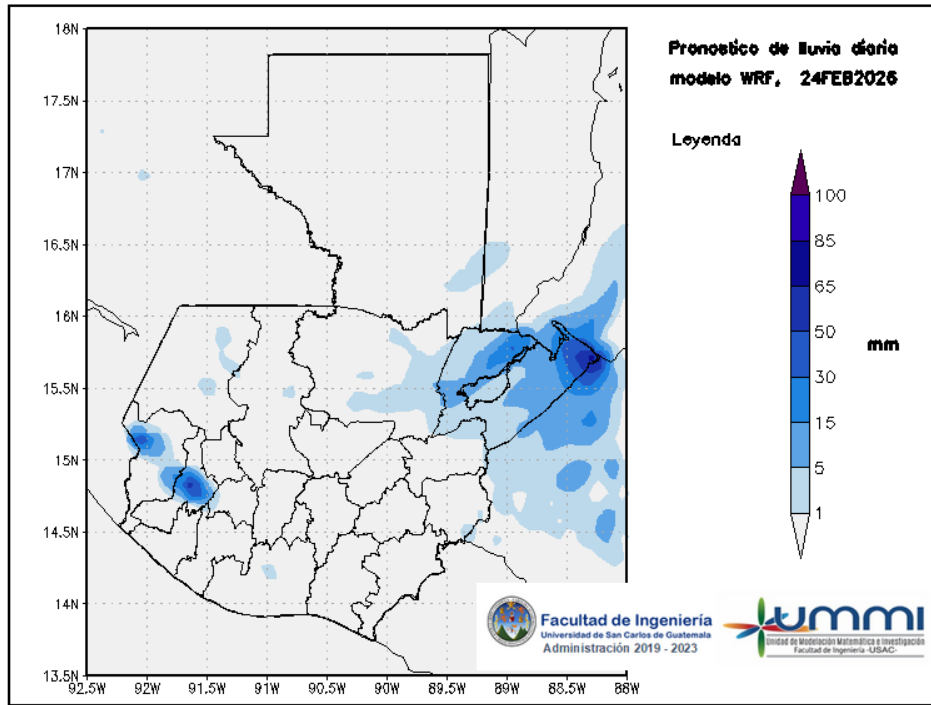
Figura 3: Pronóstico de lluvia diaria del 24 de February
