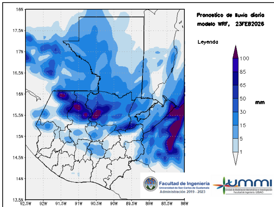
Figura 2: Pronóstico de lluvia diaria del 23 de February
