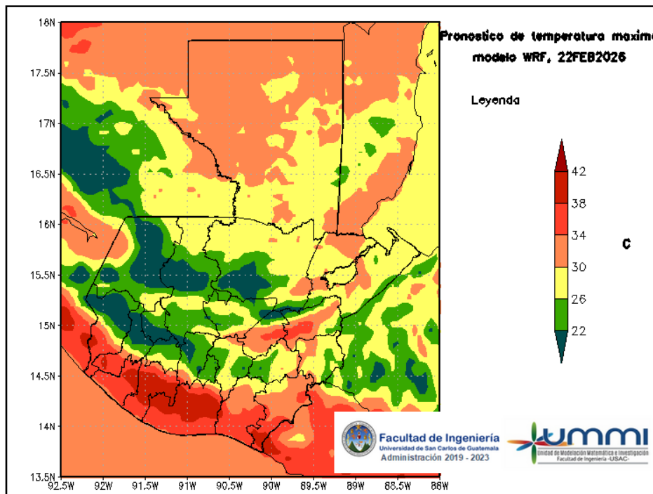
Figura 4: Pronóstico de temperatura máxima diaria del 22 de February
