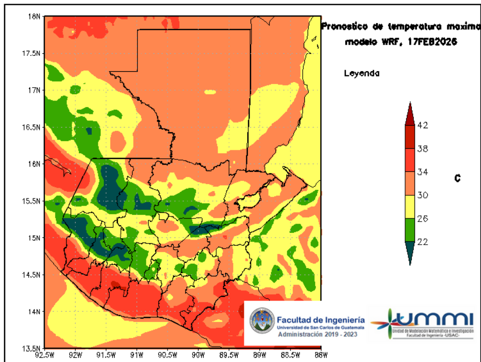
Figura 6: Pronóstico de temperatura máxima diaria del 17 de February
