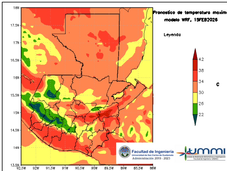
Figura 4: Pronóstico de temperatura máxima diaria del 15 de February
