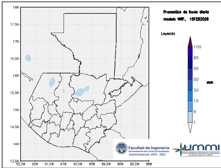
Figura 1: Pronóstico de lluvia diaria del 15 de February
