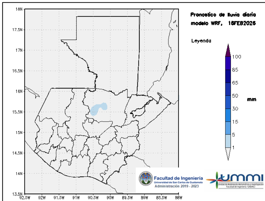
Figura 2: Pronóstico de lluvia diaria del 16 de February
