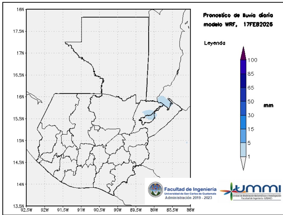
Figura 3: Pronóstico de lluvia diaria del 17 de February
