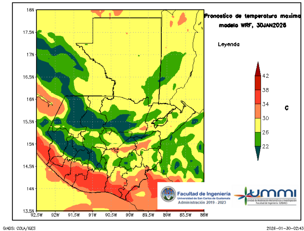
Figura 4: Pronóstico de temperatura máxima diaria del 30 de January
