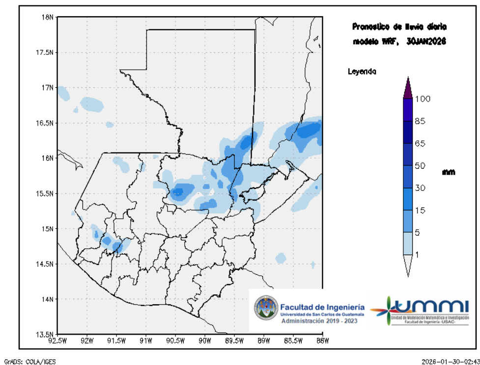
Figura 1: Pronóstico de lluvia diaria del 30 de January
