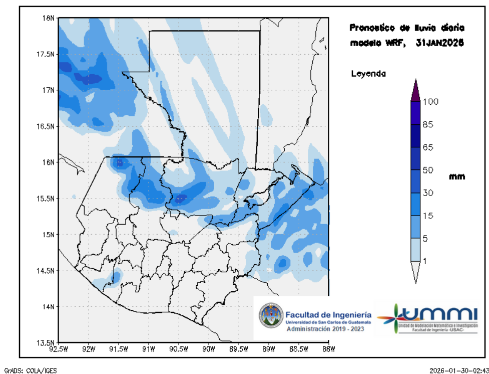
Figura 2: Pronóstico de lluvia diaria del 31 de January
