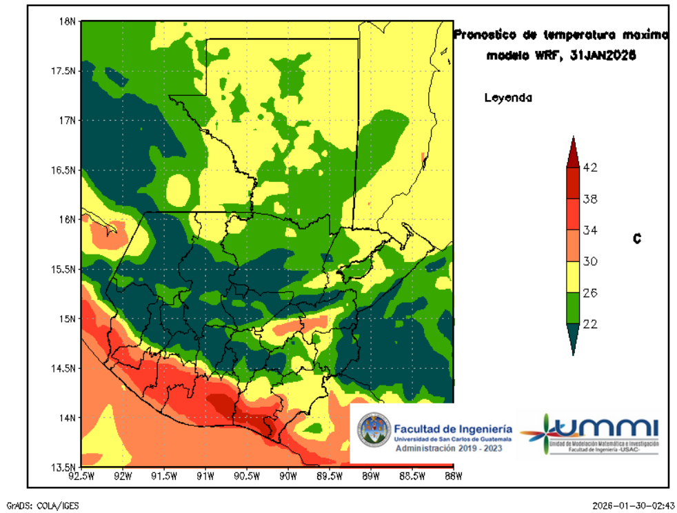
Figura 5: Pronóstico de temperatura máxima diaria del 31 de January
