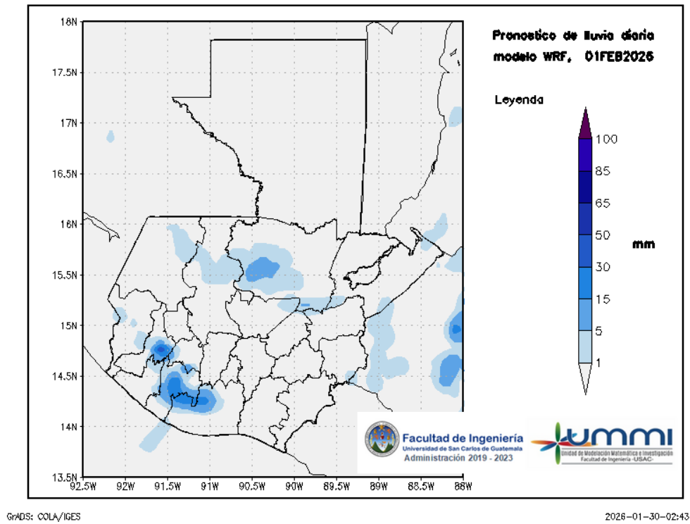
Figura 3: Pronóstico de lluvia diaria del 01 de February
