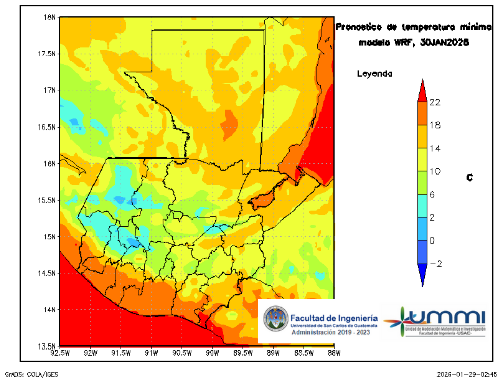
Figura 8: Pronóstico de temperatura mínima diaria del 31 de January
