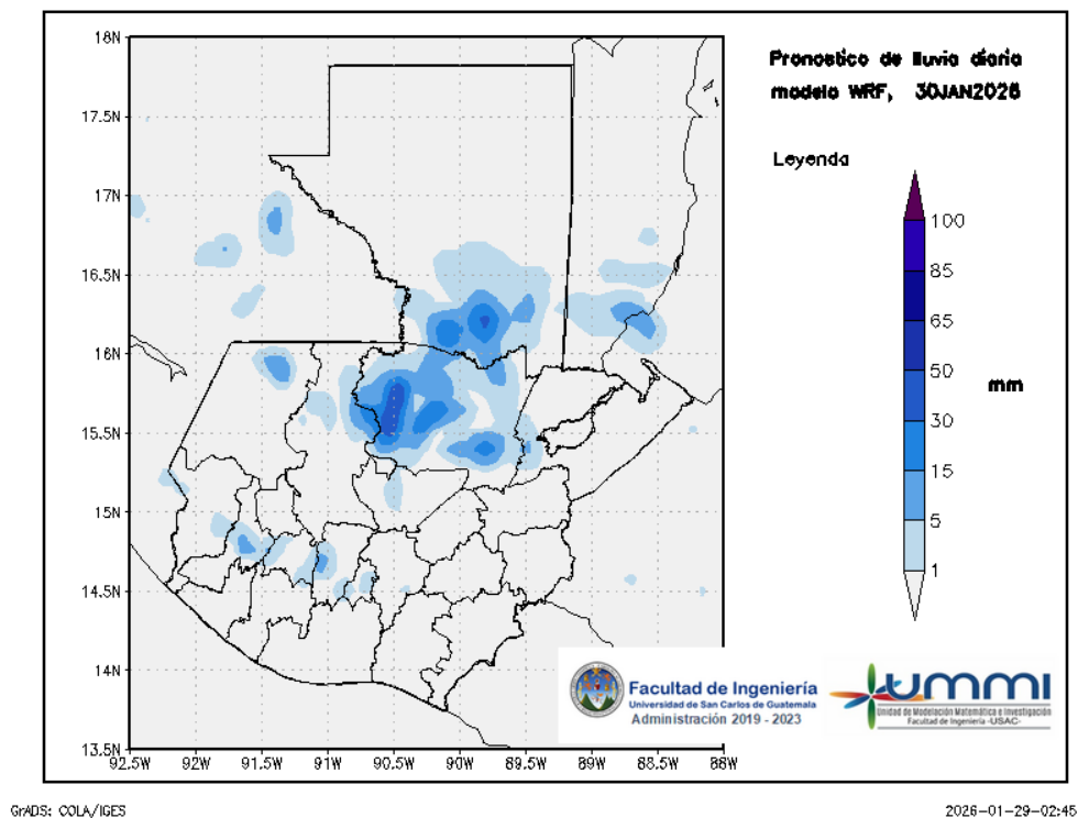
Figura 2: Pronóstico de lluvia diaria del 30 de January
