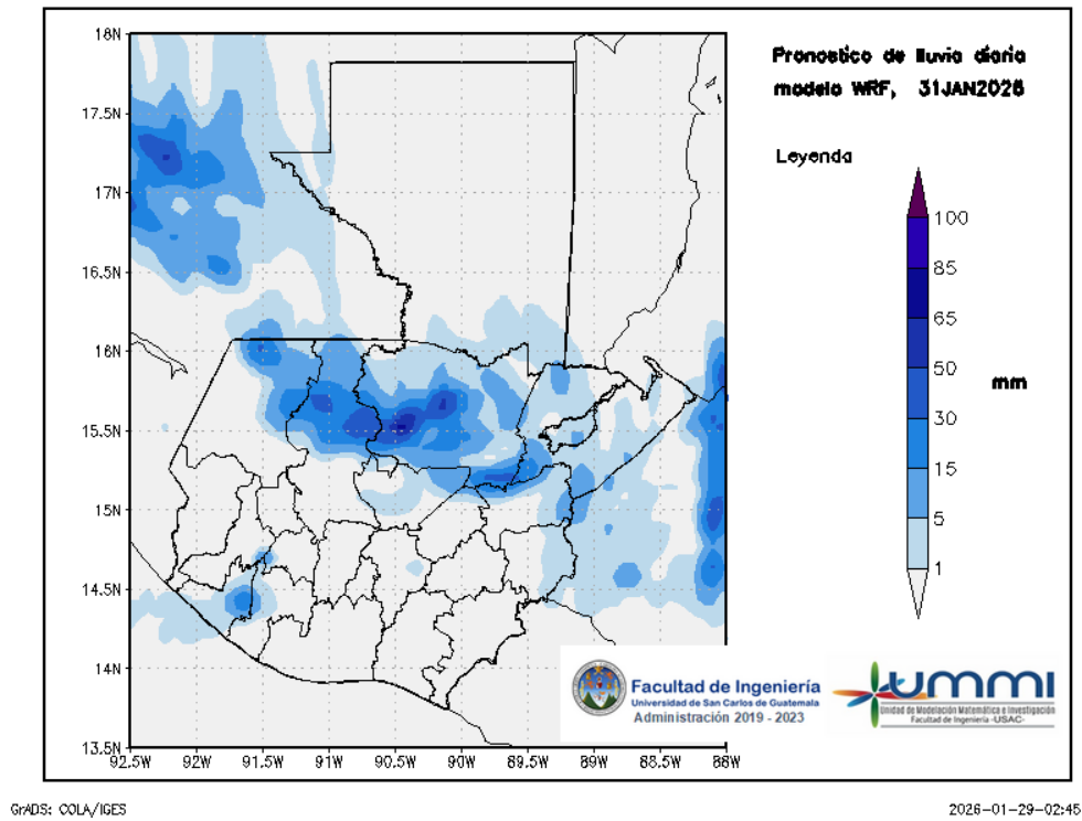
Figura 3: Pronóstico de lluvia diaria del 31 de January
