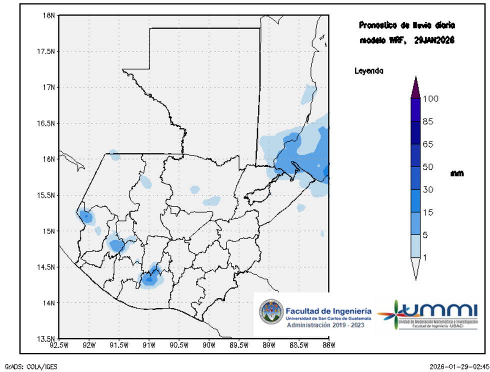
Figura 1: Pronóstico de lluvia diaria del 29 de January
