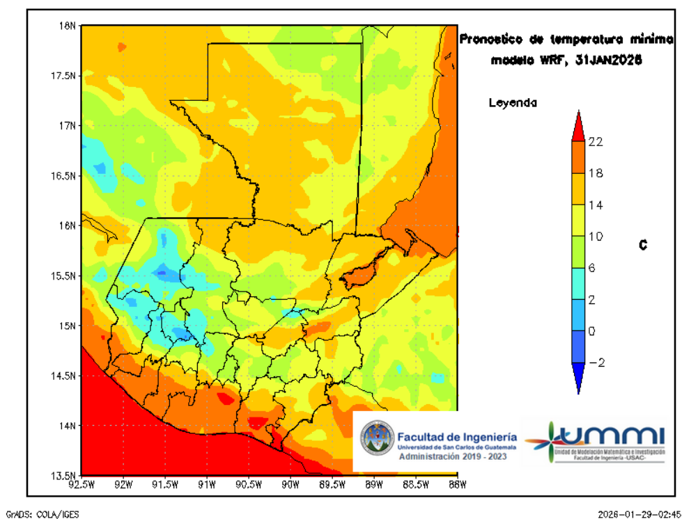
Figura 9: Pronóstico de temperatura mínima diaria del 01 de February
