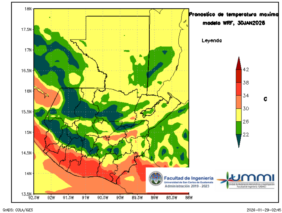
Figura 5: Pronóstico de temperatura máxima diaria del 30 de January
