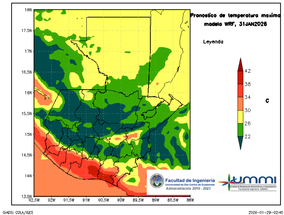
Figura 6: Pronóstico de temperatura máxima diaria del 31 de January
