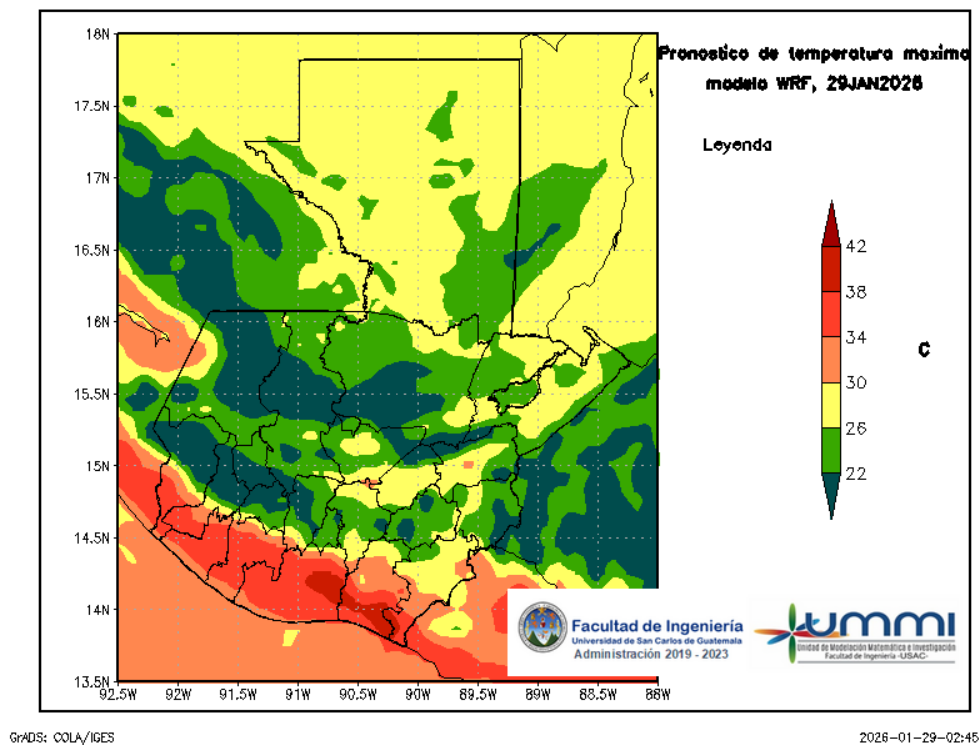
Figura 4: Pronóstico de temperatura máxima diaria del 29 de January
