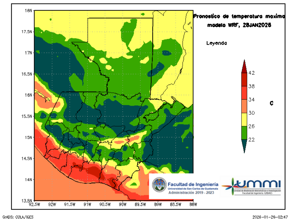
Figura 6: Pronóstico de temperatura máxima diaria del 28 de January
