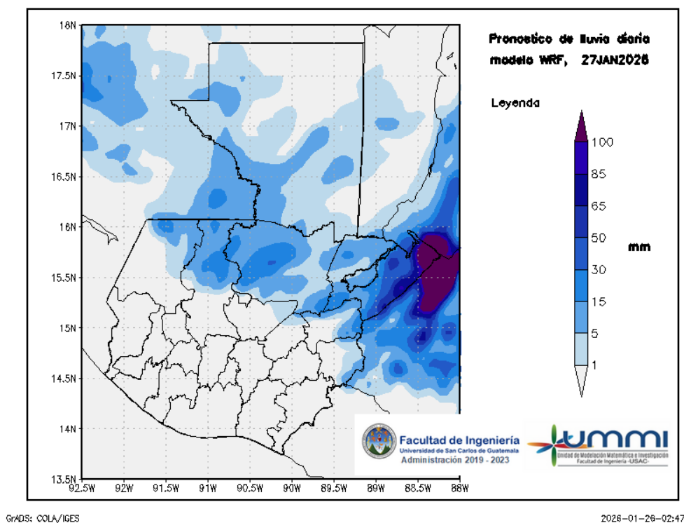
Figura 2: Pronóstico de lluvia diaria del 27 de January
