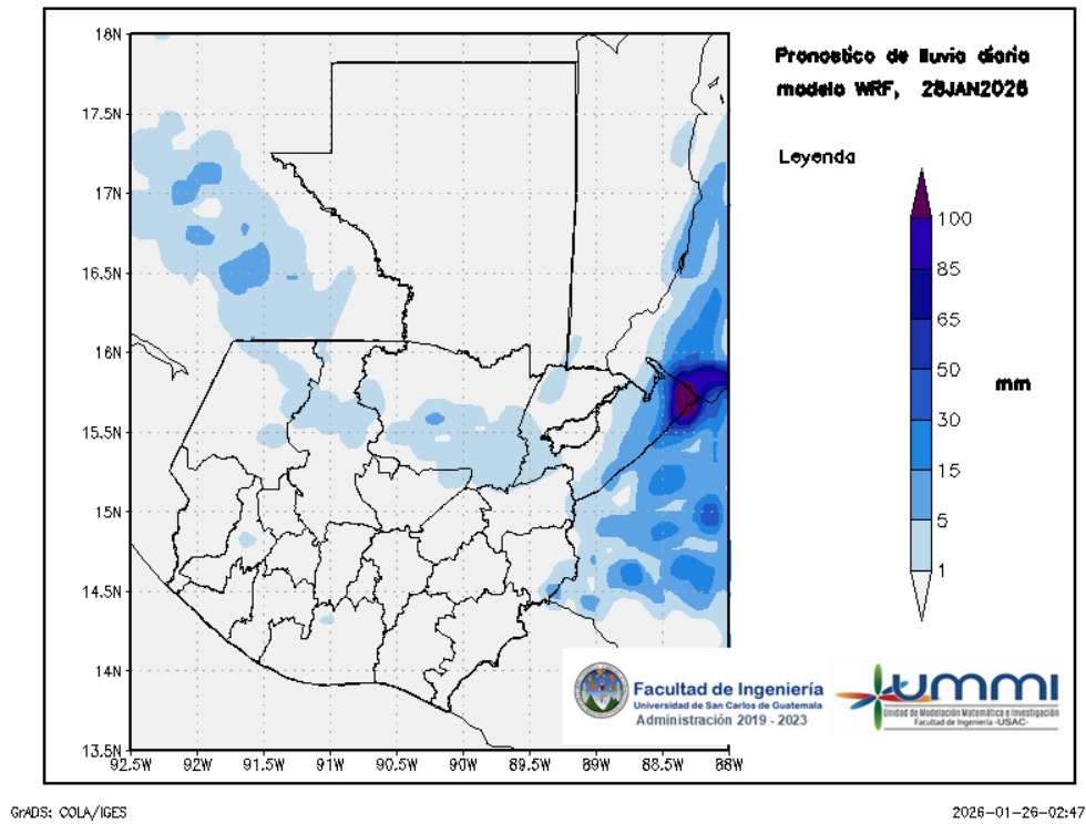
Figura 3: Pronóstico de lluvia diaria del 28 de January
