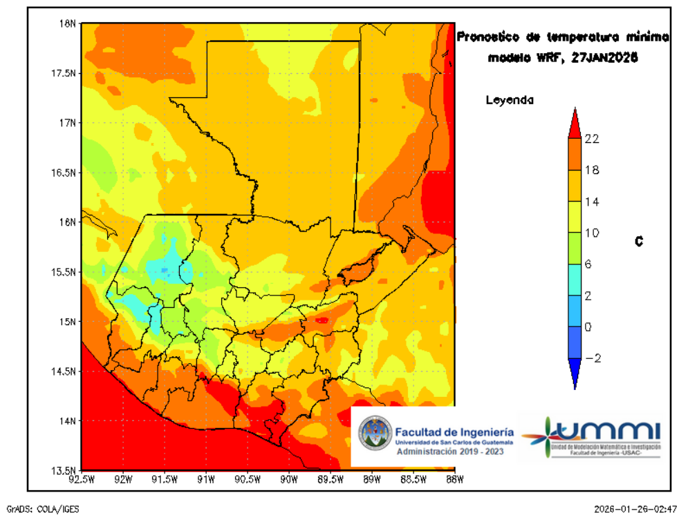
Figura 8: Pronóstico de temperatura mínima diaria del 28 de January
