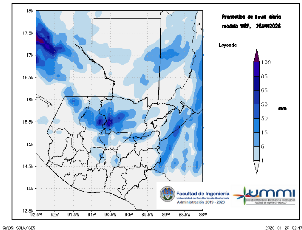
Figura 1: Pronóstico de lluvia diaria del 26 de January
