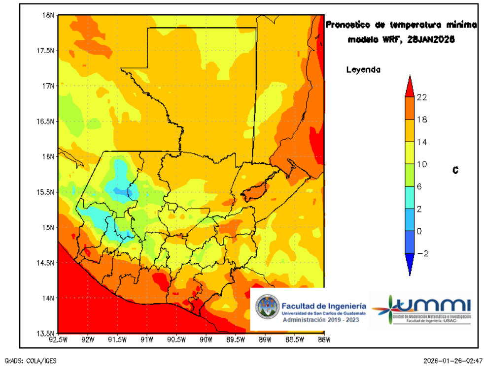
Figura 9: Pronóstico de temperatura mínima diaria del 29 de January
