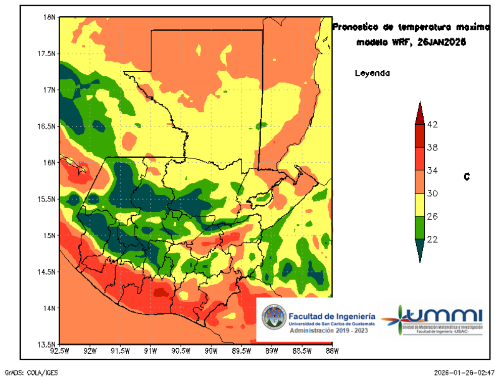
Figura 4: Pronóstico de temperatura máxima diaria del 26 de January
