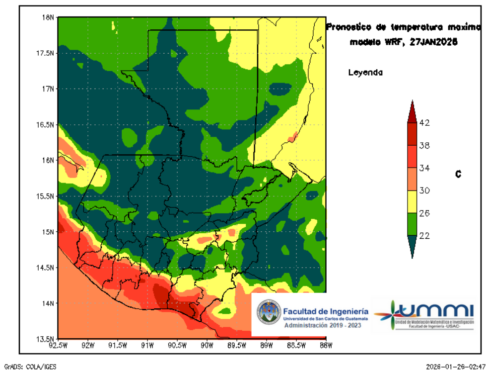
Figura 5: Pronóstico de temperatura máxima diaria del 27 de January
