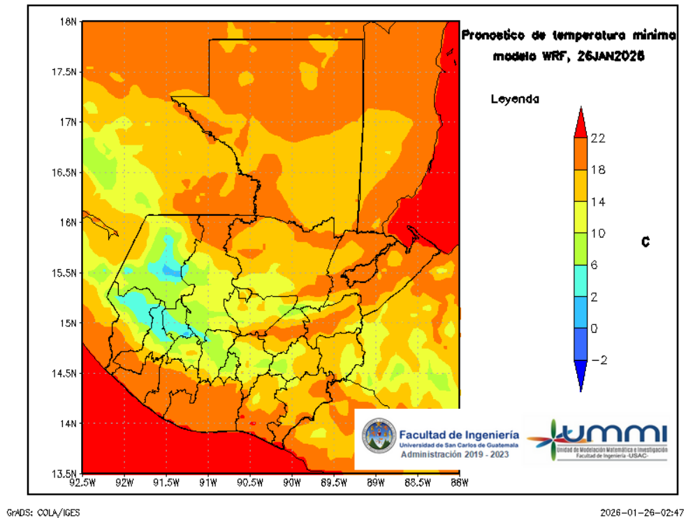
Figura 7: Pronóstico de temperatura mínima diaria del 27 de January
