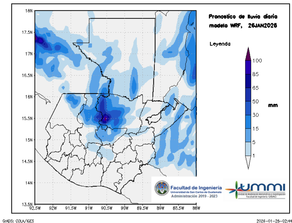
Figura 2: Pronóstico de lluvia diaria del 26 de January
