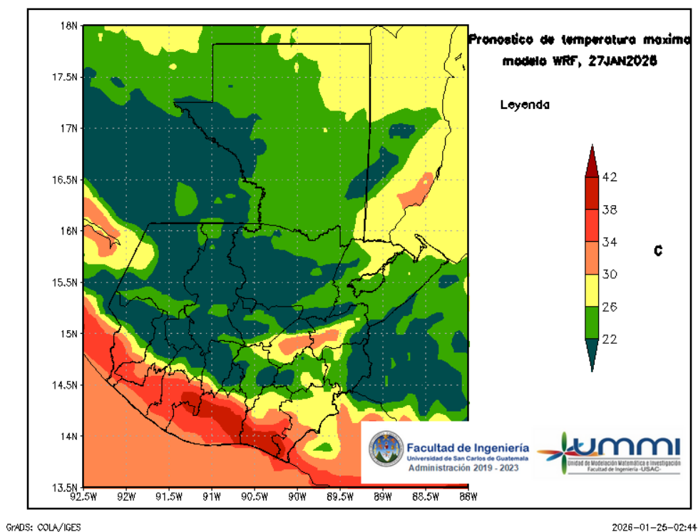
Figura 6: Pronóstico de temperatura máxima diaria del 27 de January
