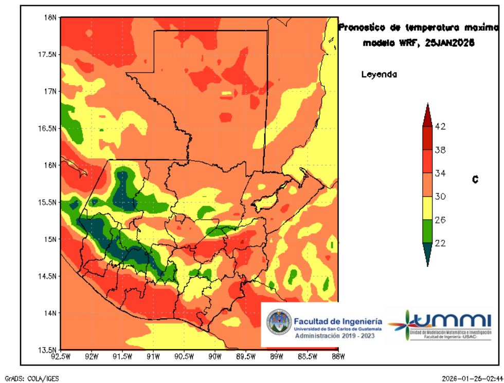
Figura 4: Pronóstico de temperatura máxima diaria del 25 de January
