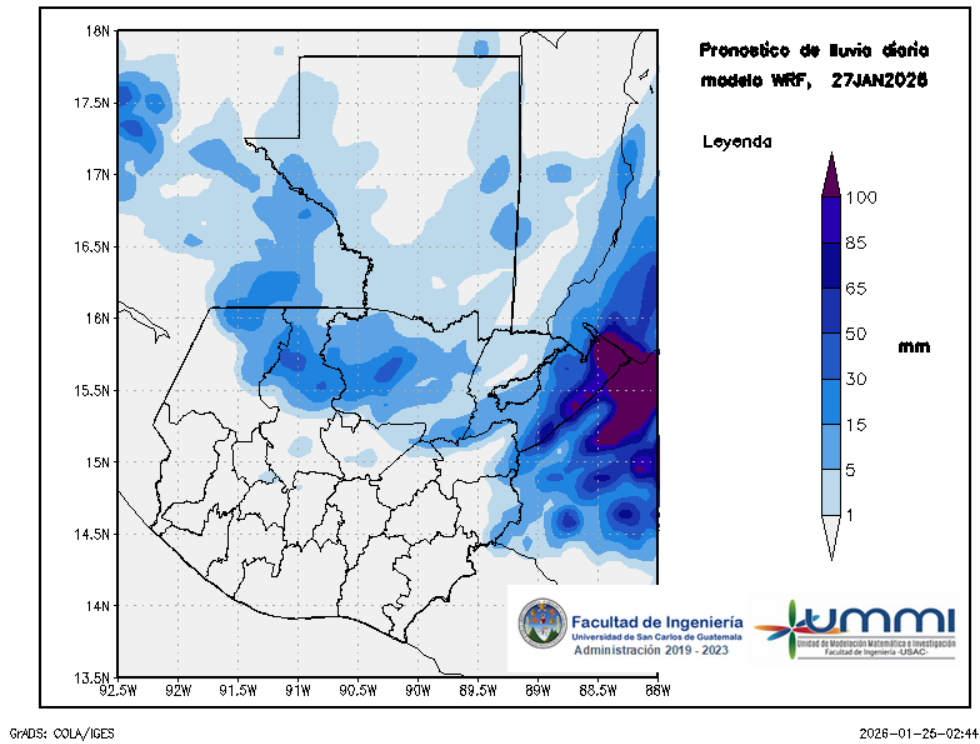
Figura 3: Pronóstico de lluvia diaria del 27 de January
