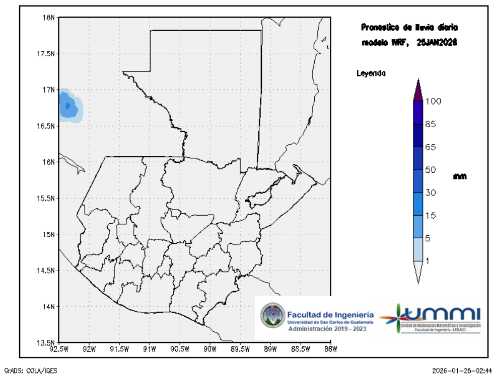
Figura 1: Pronóstico de lluvia diaria del 25 de January
