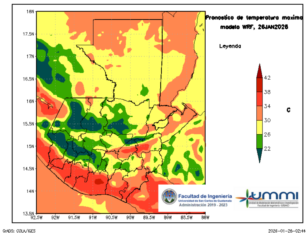
Figura 5: Pronóstico de temperatura máxima diaria del 26 de January
