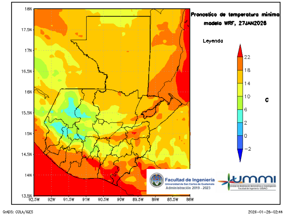
Figura 9: Pronóstico de temperatura mínima diaria del 28 de January
