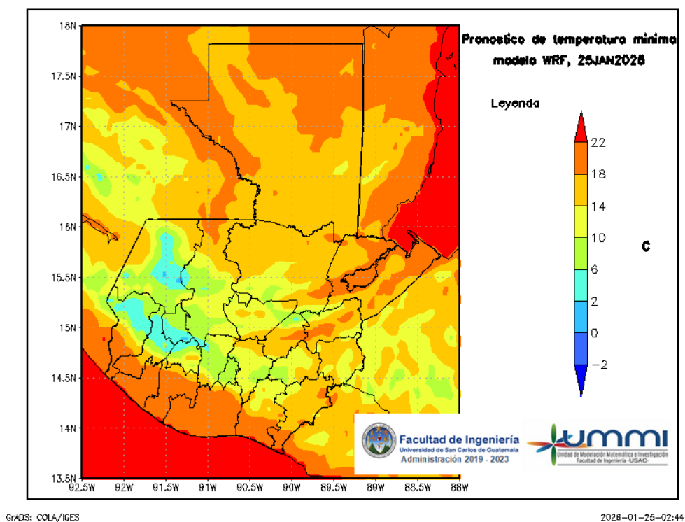
Figura 7: Pronóstico de temperatura mínima diaria del 26 de January
