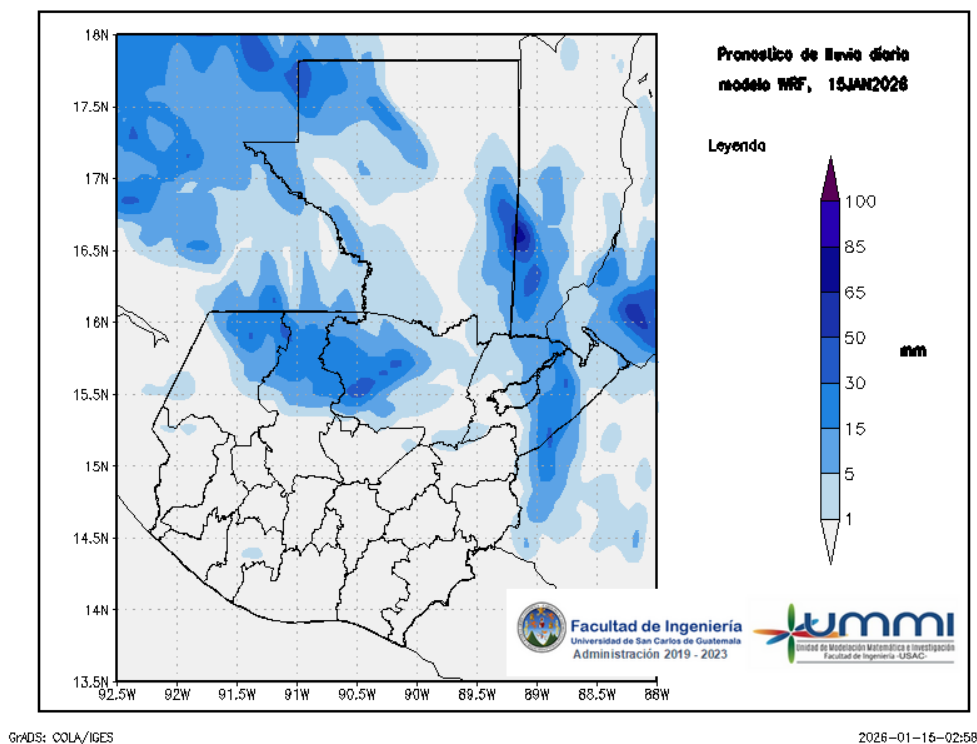
Figura 1: Pronóstico de lluvia diaria del 15 de January
