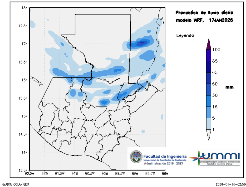
Figura 3: Pronóstico de lluvia diaria del 17 de January
