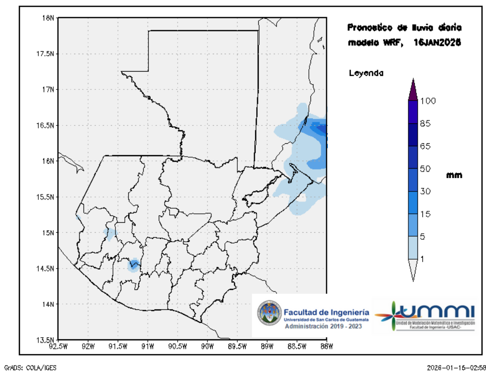
Figura 2: Pronóstico de lluvia diaria del 16 de January
