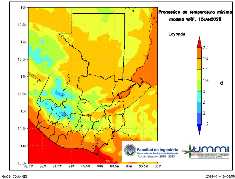
Figura 7: Pronóstico de temperatura mínima diaria del 16 de January
