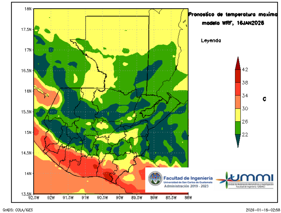
Figura 5: Pronóstico de temperatura máxima diaria del 16 de January
