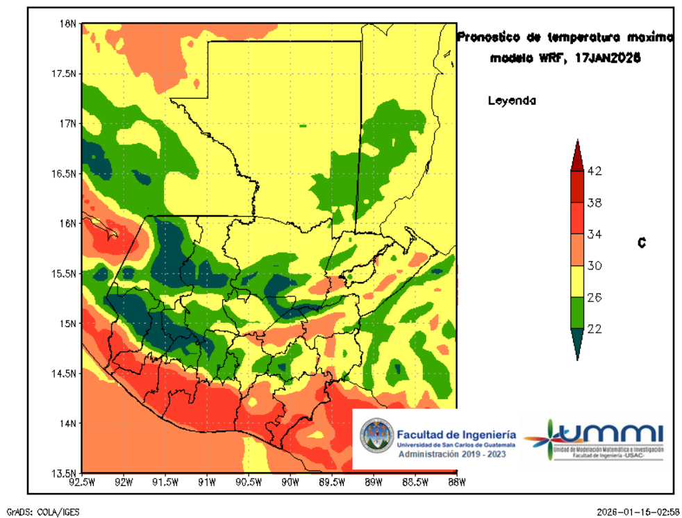
Figura 6: Pronóstico de temperatura máxima diaria del 17 de January
