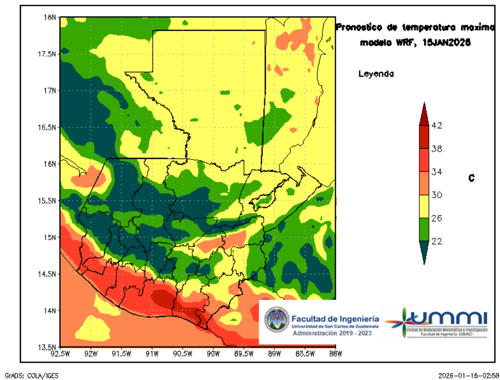
Figura 4: Pronóstico de temperatura máxima diaria del 15 de January
