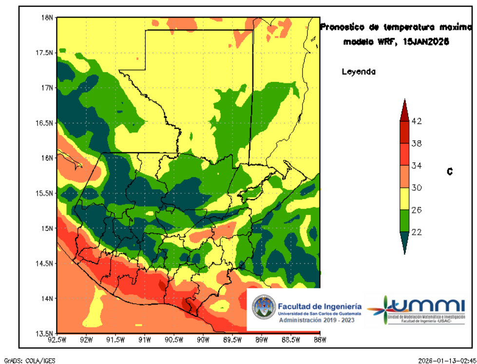
Figura 6: Pronóstico de temperatura máxima diaria del 15 de January
