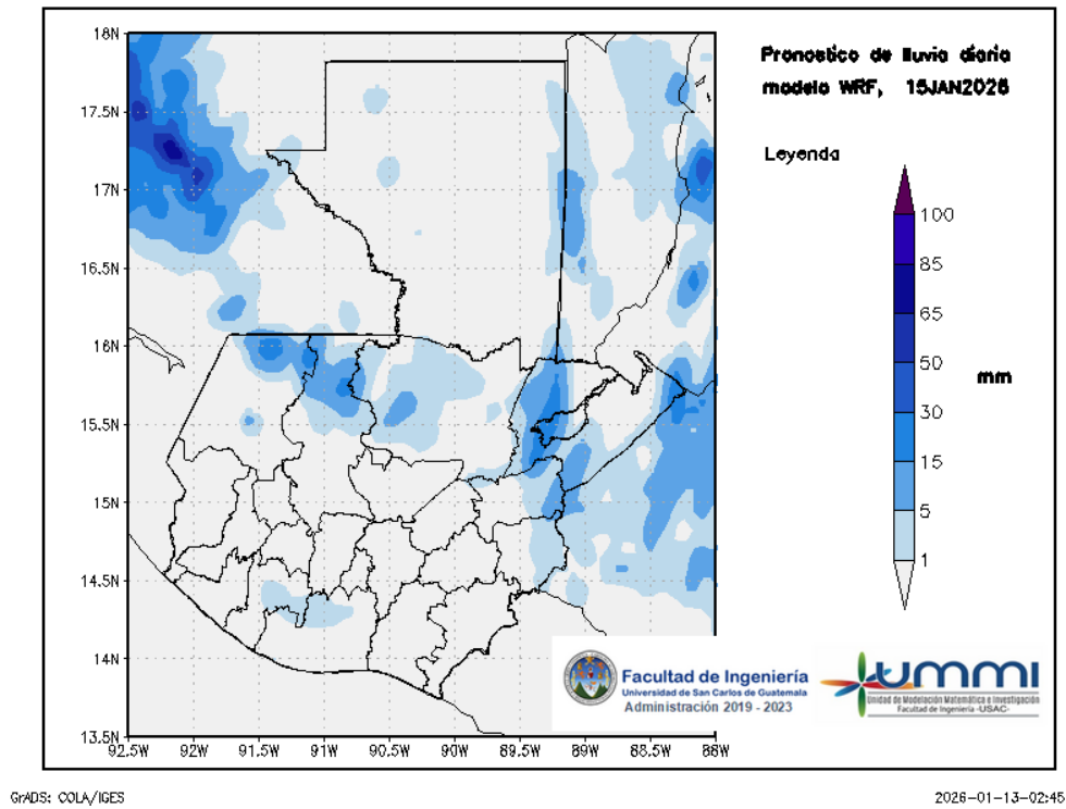
Figura 3: Pronóstico de lluvia diaria del 15 de January
