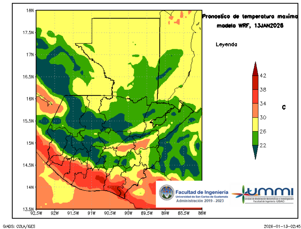
Figura 4: Pronóstico de temperatura máxima diaria del 13 de January
