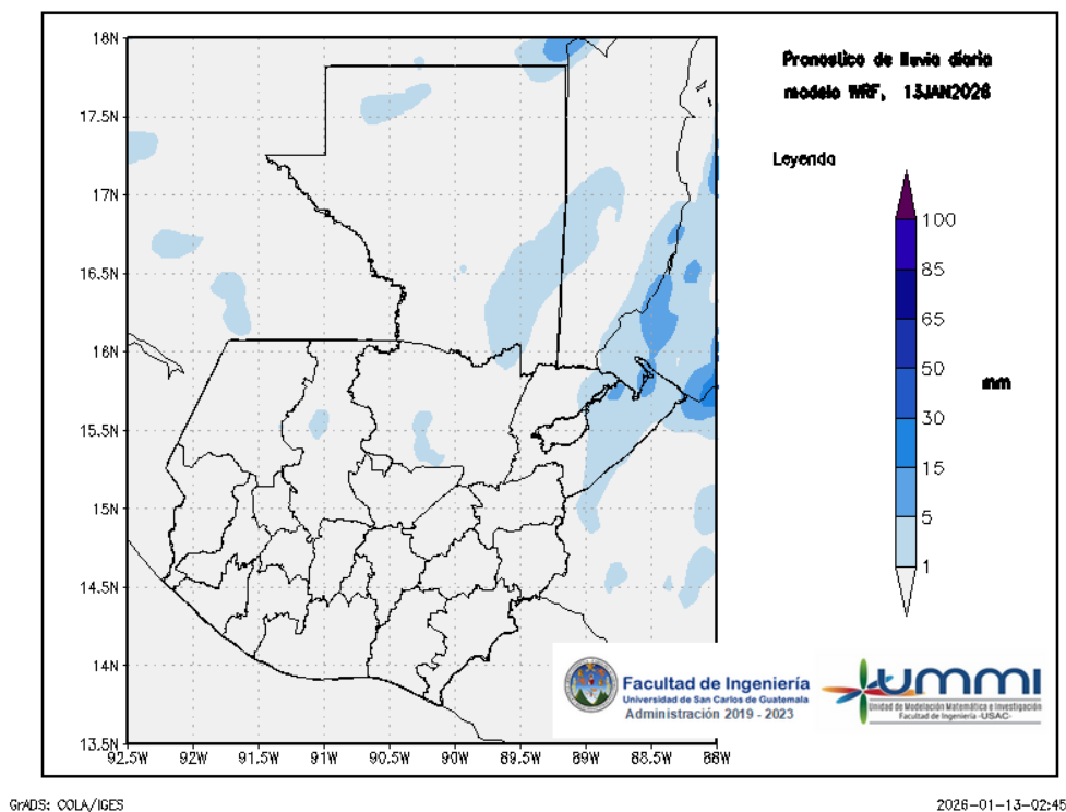
Figura 1: Pronóstico de lluvia diaria del 13 de January
