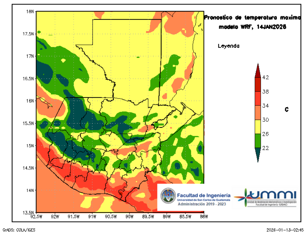
Figura 5: Pronóstico de temperatura máxima diaria del 14 de January
